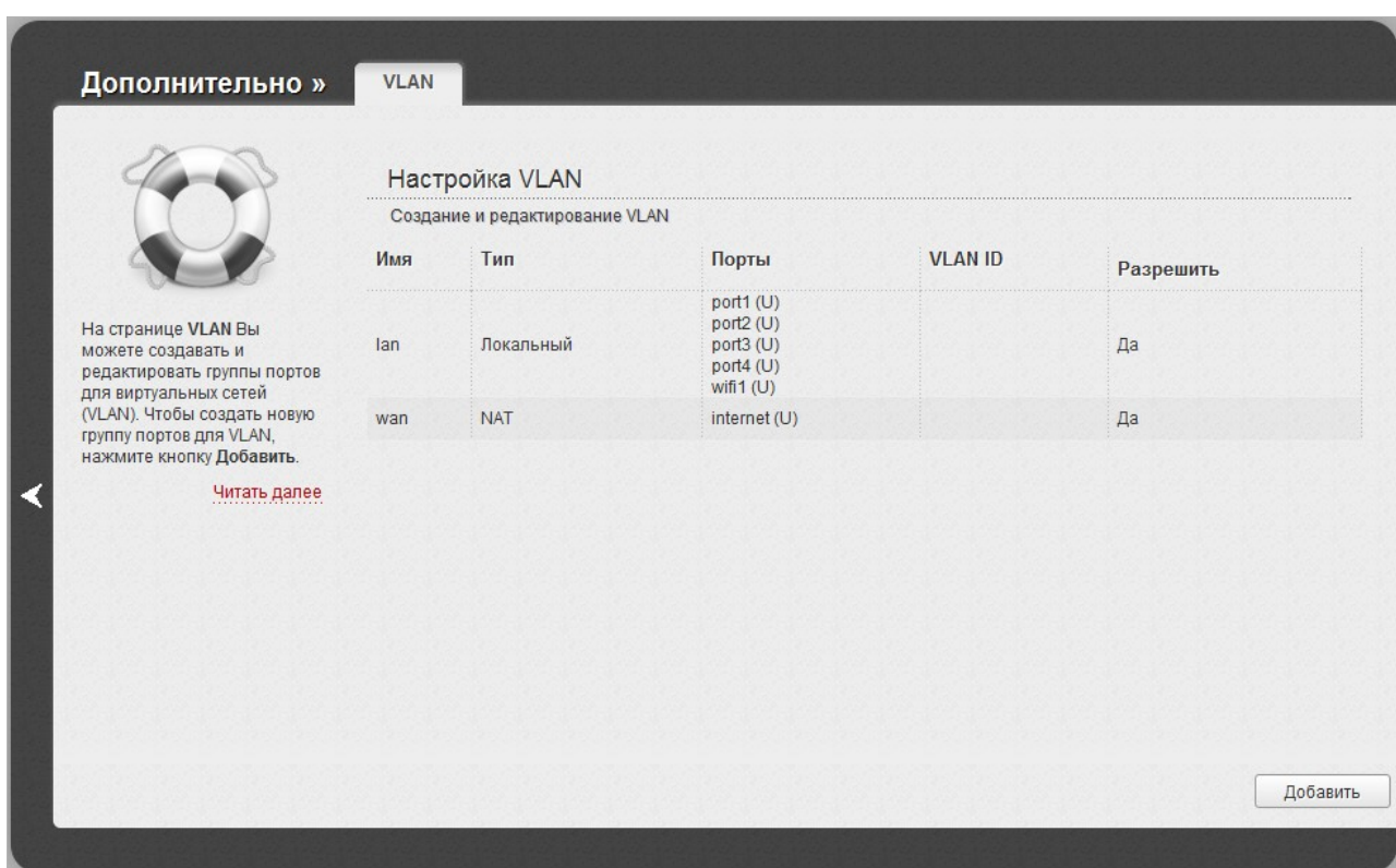
Рисунок 110. Страница Дополнительно / VLAN .
