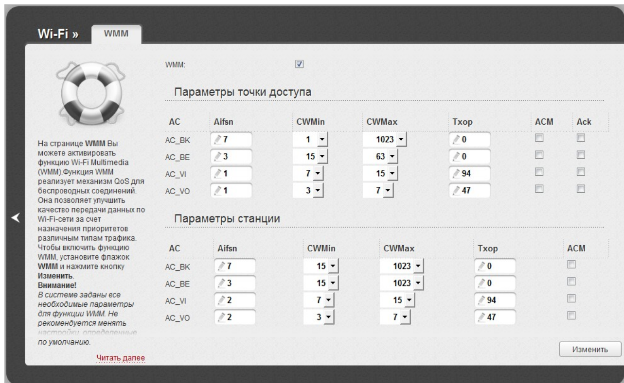
Рисунок 109. Страница для настройки функции WMM.
