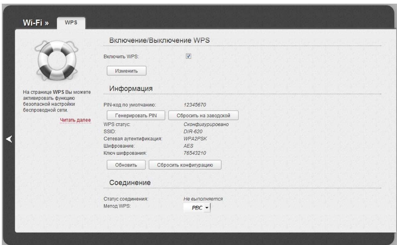
Рисунок 107. Страница для настройки функции WPS.
