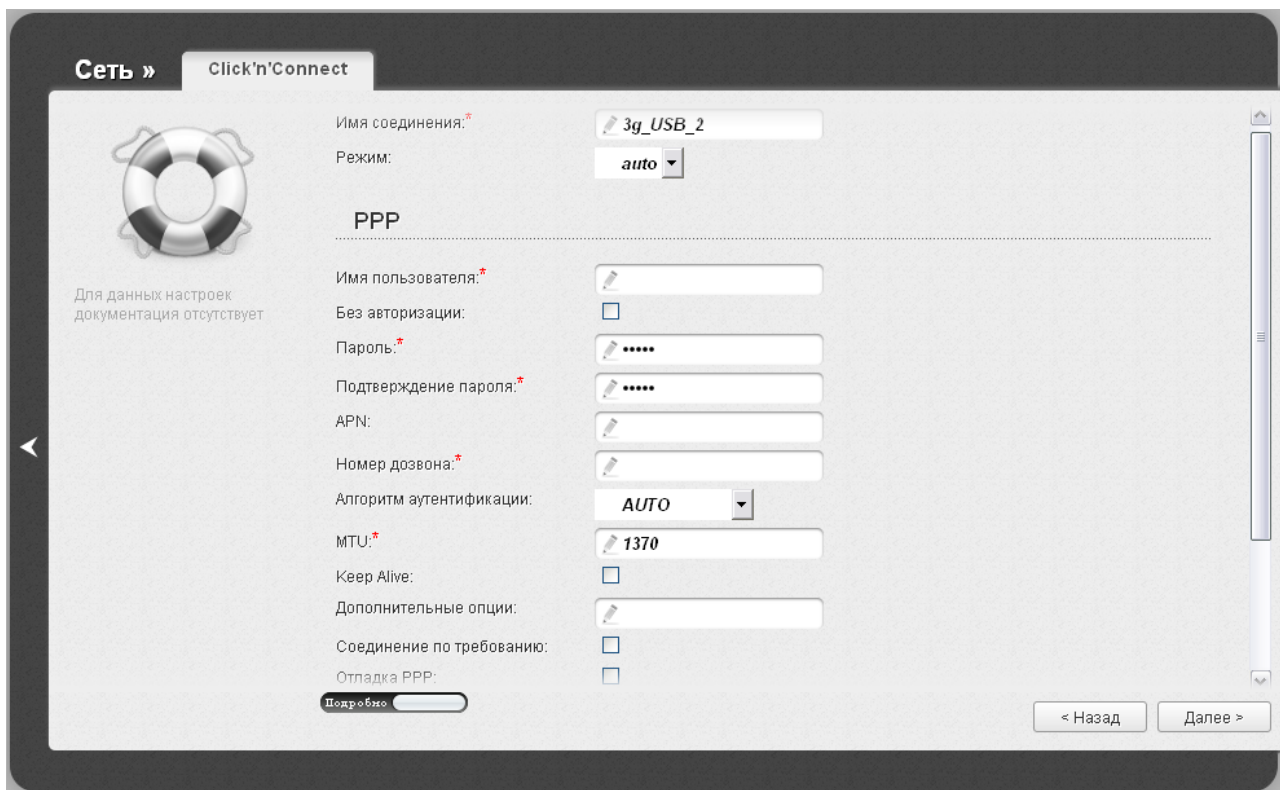
Рисунок 54. Настройка WAN-соединения типа 3G. Экспертный режим настроек. Раздел PPP.
