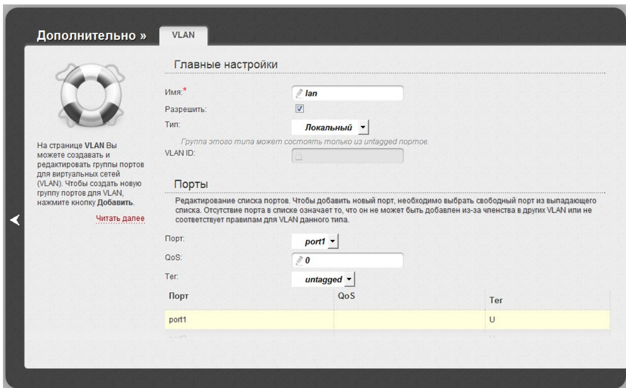
Рисунок 111. Страница редактирования группы портов для VLAN.
