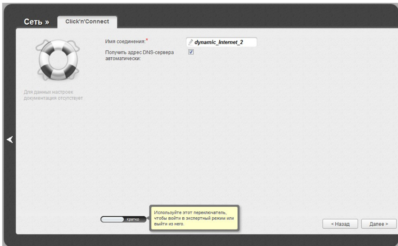
Рисунок 34. Настройка WAN-соединения типа Динамический IP.
