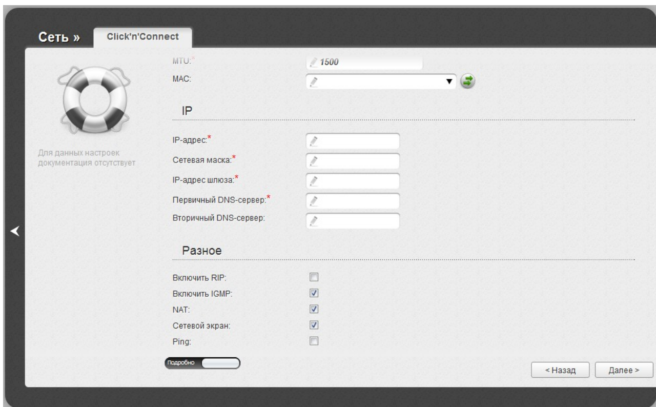
Рисунок 42. Настройка WAN-соединения типа PPTP + Статический IP. Экспертный режим настроек. Разделы IP и Разное.
