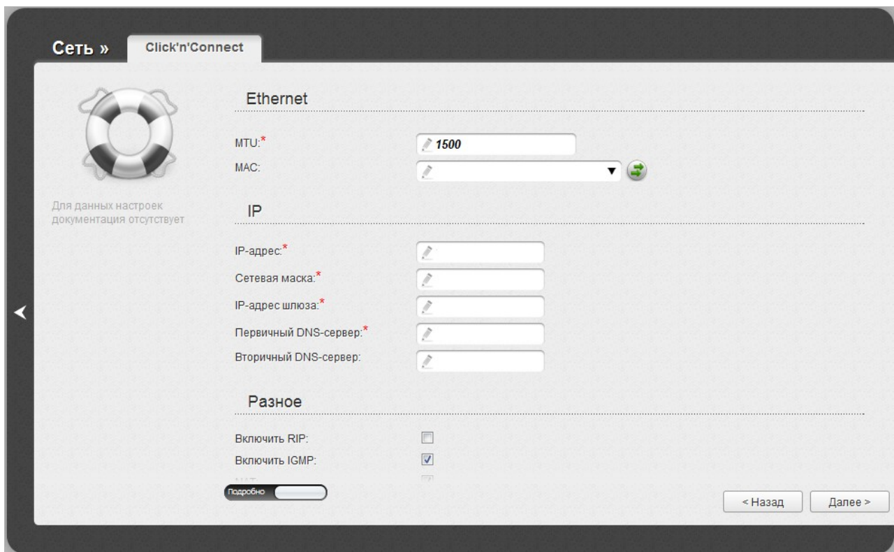
Рисунок 41. Настройка WAN-соединения типа PPTP + Статический IP. Экспертный режим настроек. Раздел Ethernet .
