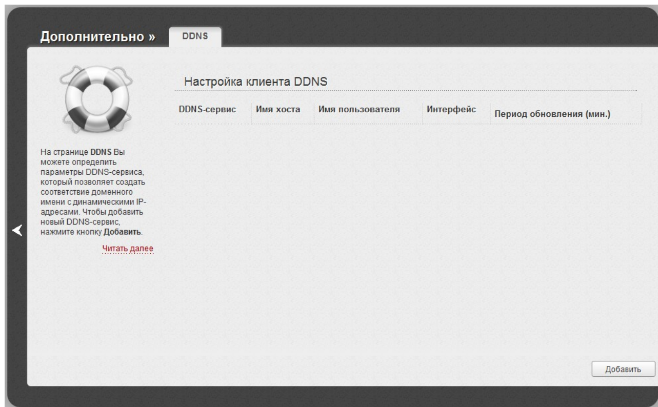
Рисунок 113. Страница Дополнительно / DDNS .
