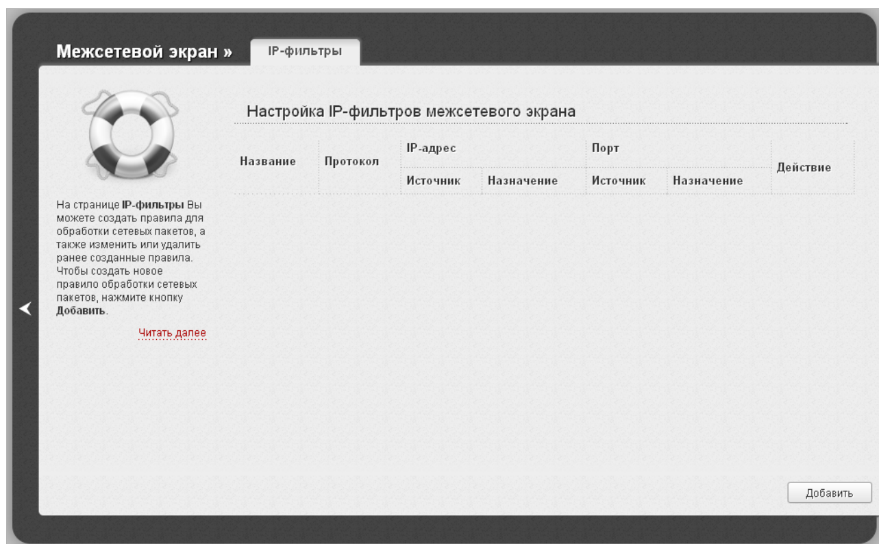
Рисунок 121. Страница Межсетевой экран / IP-фильтры .
