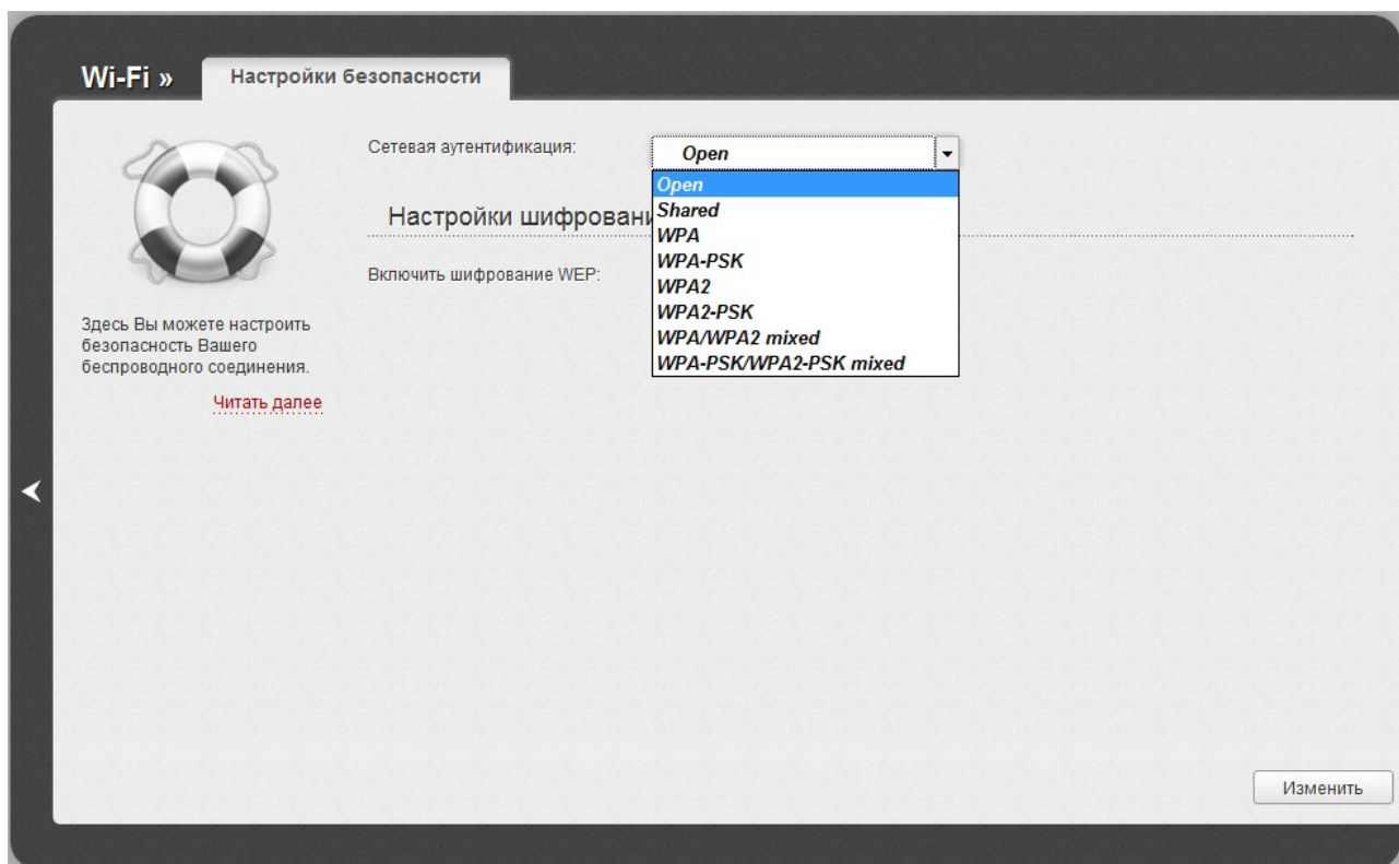
Рисунок 100. Типы аутентификации, поддерживаемые маршрутизатором.
