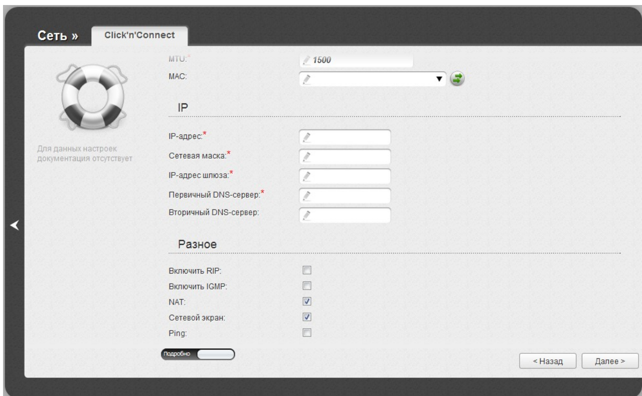
Рисунок 33. Настройка WAN-соединения типа Статический IP. Экспертный режим настроек. Разделы IP и Разное.
