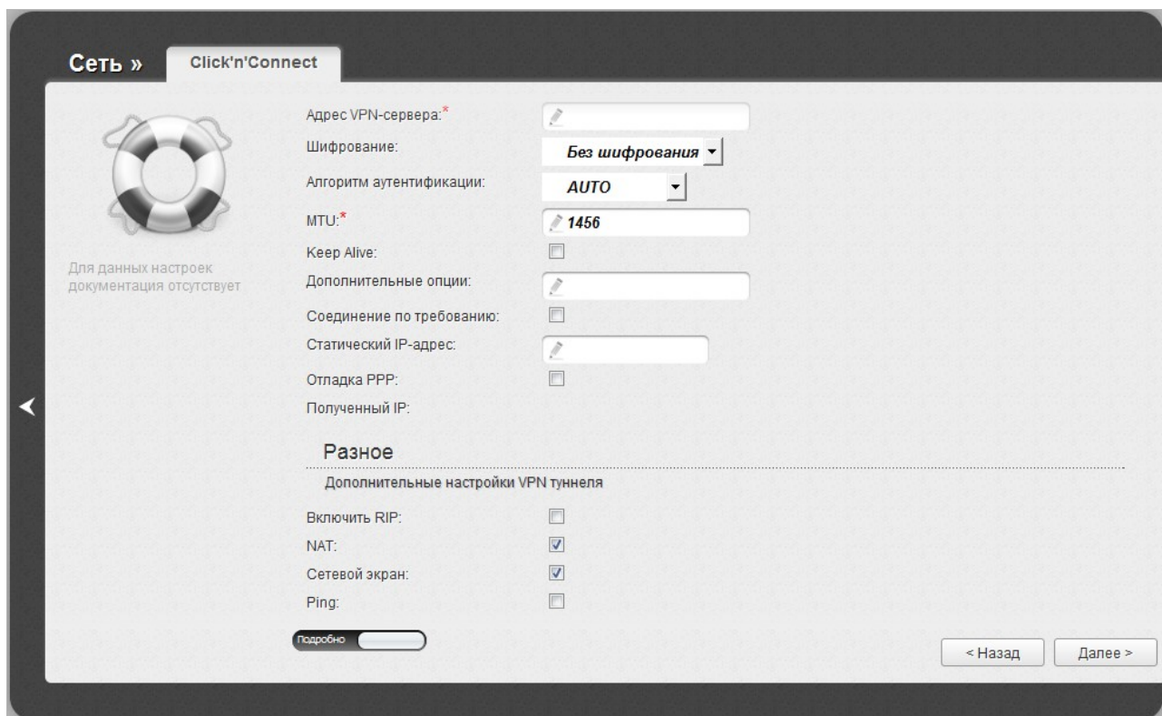
Рисунок 46. Настройка WAN-соединения типа PPTP + Статический IP. Экспертный режим настроек. Раздел Разное.
