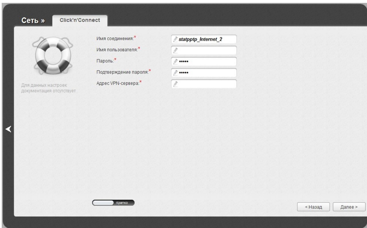
Рисунок 44. Настройка WAN-соединения типа PPTP + Статический IP.
