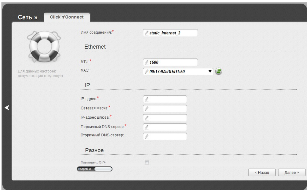
Рисунок 32. Настройка WAN-соединения типа Статический IP. Экспертный режим настроек. Раздел Ethernet .
