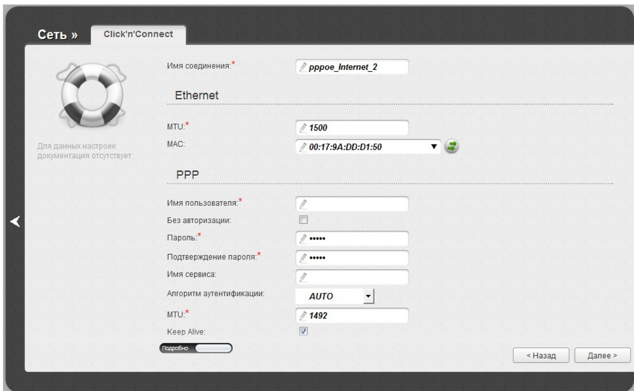
Рисунок 28. Настройка WAN-соединения типа PPPoE. Экспертный режим настроек. Раздел Ethernet.
