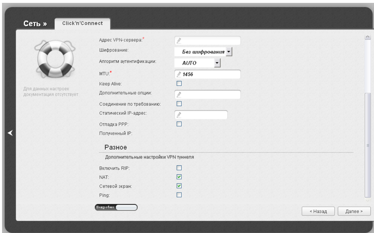
Рисунок 39. Настройка WAN-соединения типа PPTP. Экспертный режим настроек. Раздел Разное .
