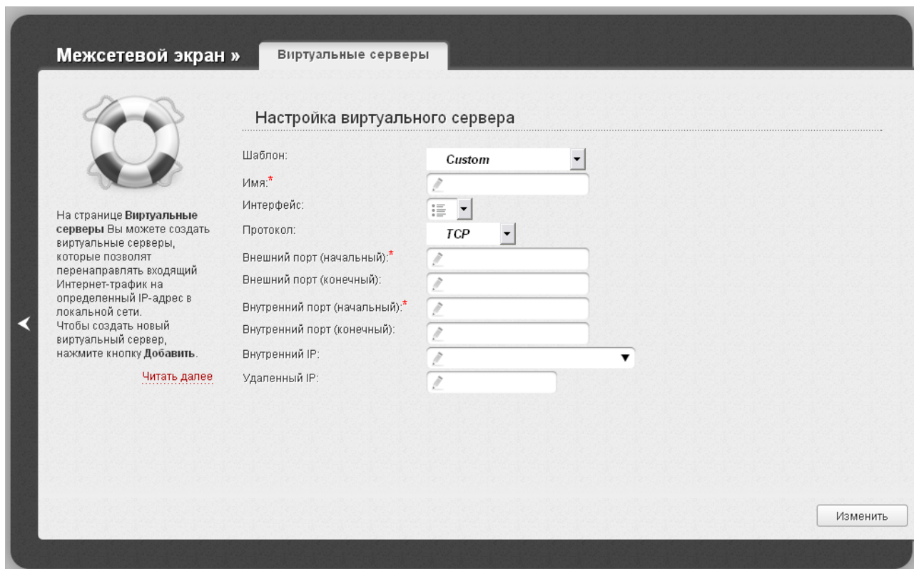
Рисунок 124. Страница добавления виртуального сервера.
