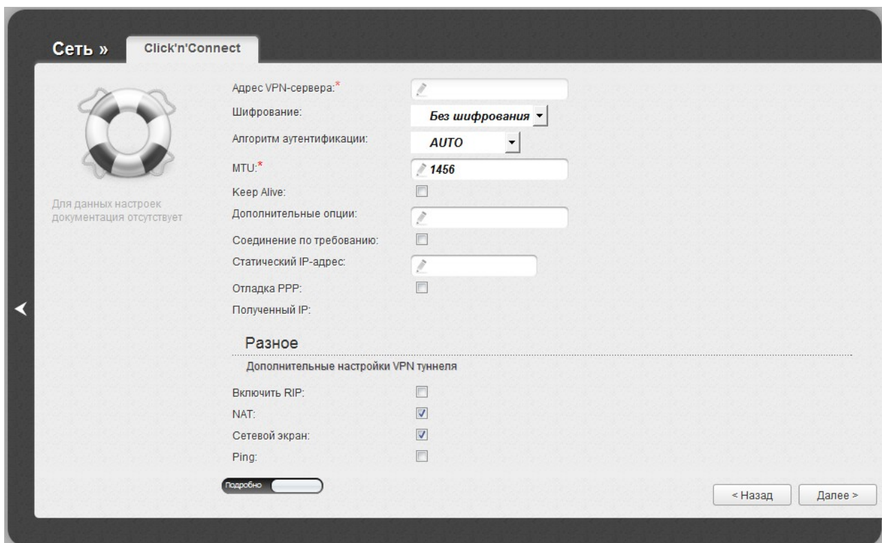
Рисунок 52. Настройка WAN-соединения типа PPTP + Динамический IP. Экспертный режим настроек. Раздел Разное .
