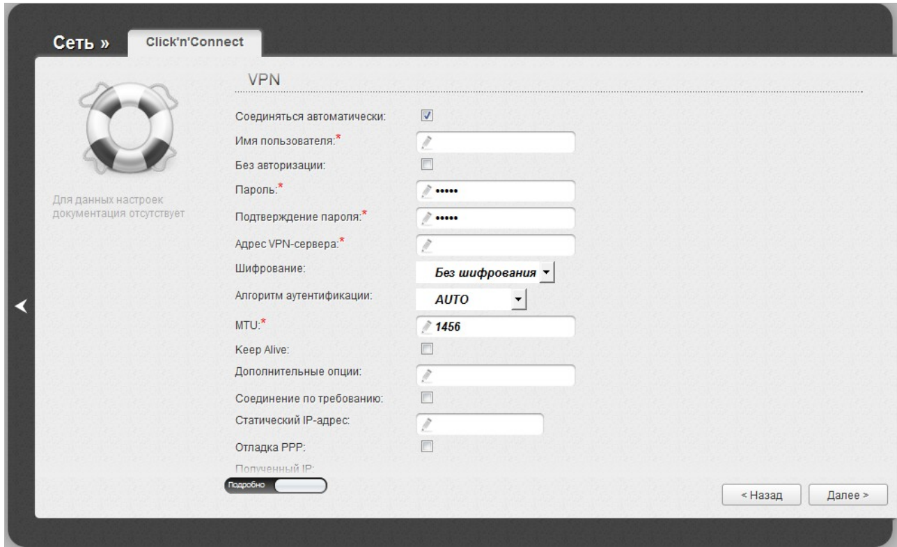
Рисунок 51. Настройка WAN-соединения типа PPTP + Динамический IP. Экспертный режим настроек. Раздел VPN.
