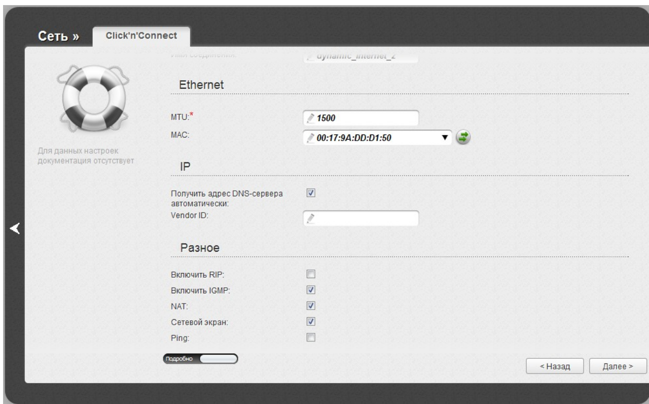
Рисунок 36. Настройка WAN-соединения типа Динамический IP. Экспертный режим настроек. Разделы IP и Разное.
