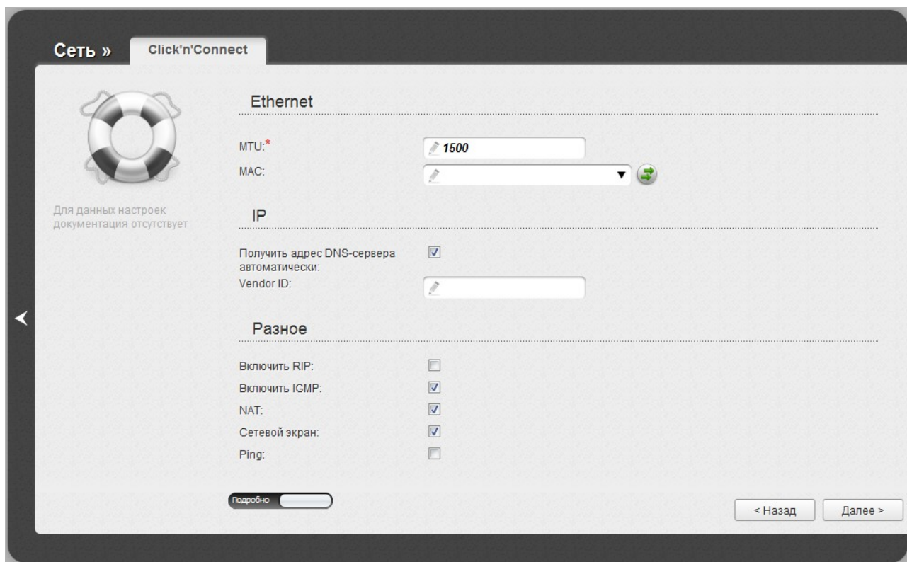
Рисунок 49. Настройка WAN-соединения типа PPTP + Динамический IP. Экспертный режим настроек. Разделы IP и Разное.
