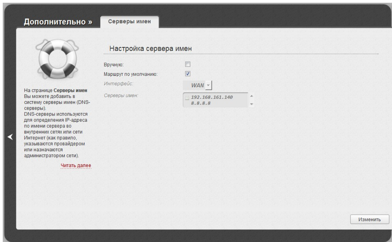
Рисунок 115. Страница Дополнительно / Серверы имен .
