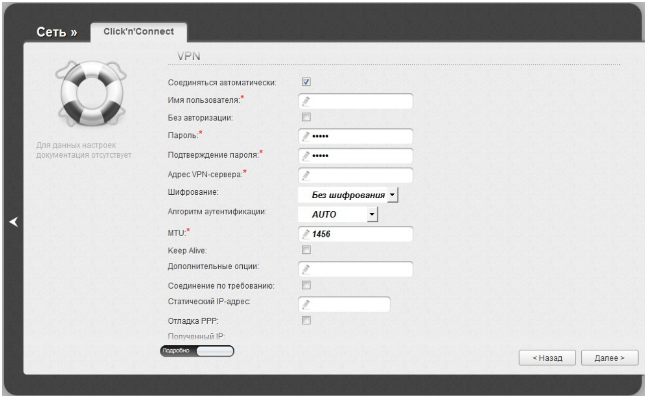
Рисунок 45. Настройка WAN-соединения типа PPTP + Статический IP. Экспертный режим настроек. Раздел VPN.
