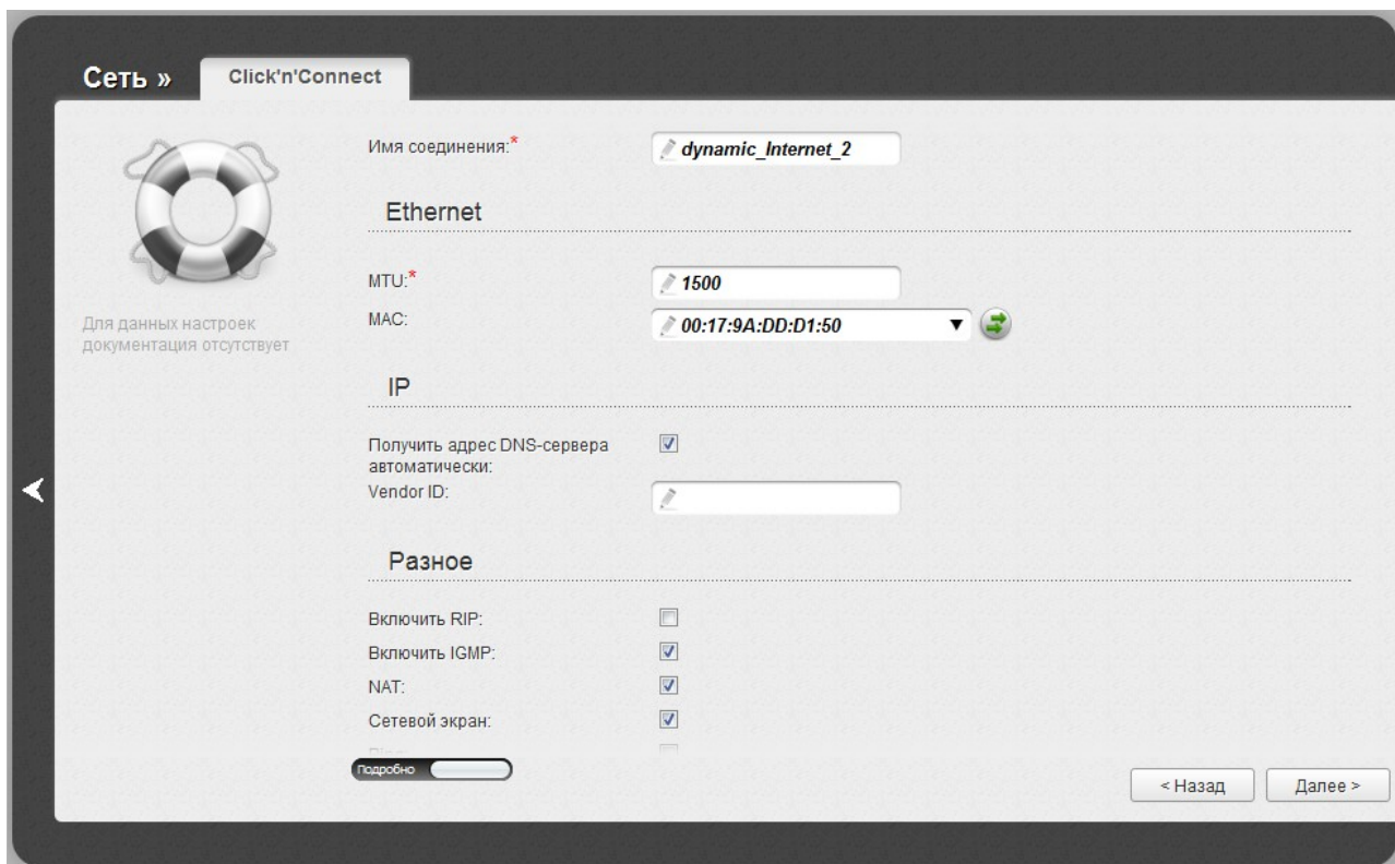
Рисунок 35. Настройка WAN-соединения типа Динамический IP. Экспертный режим настроек. Раздел Ethernet .
