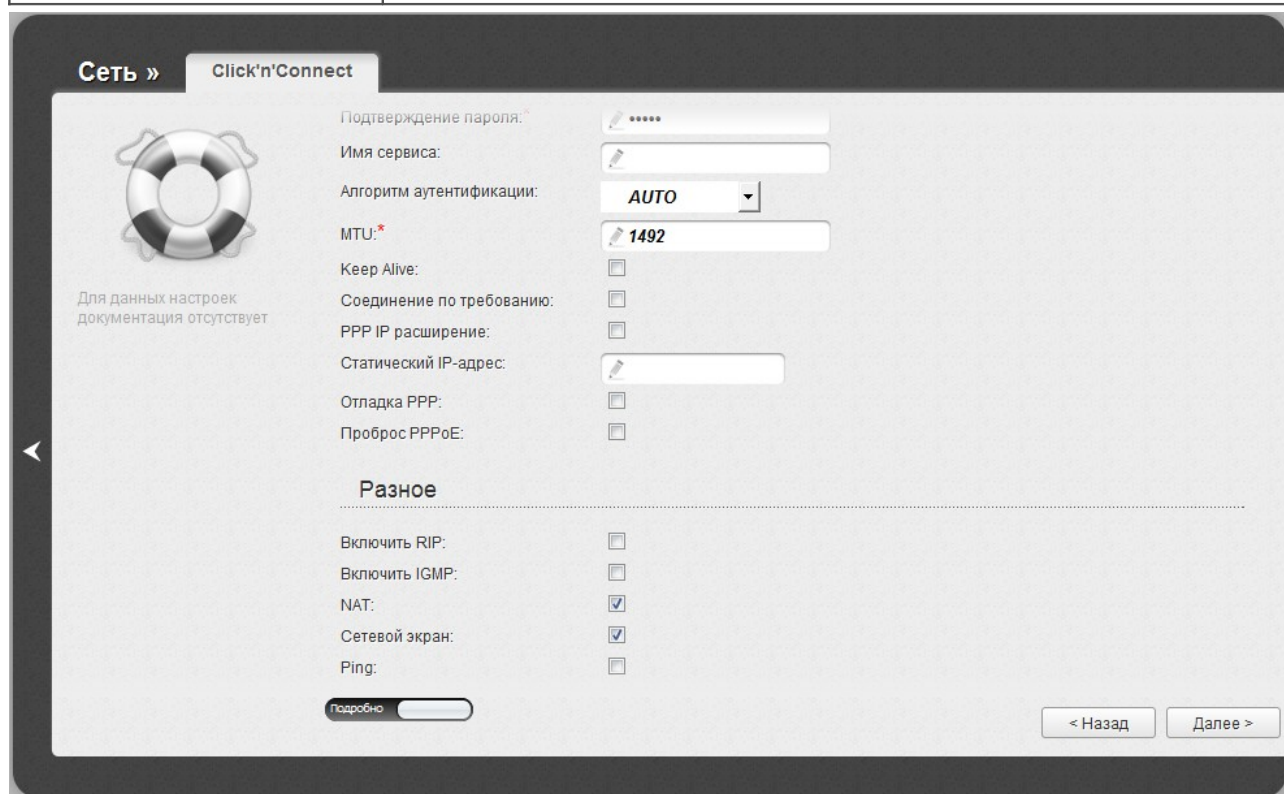
Рисунок 30. Настройка WAN-соединения типа PPPoE. Экспертный режим настроек. Раздел Разное .
