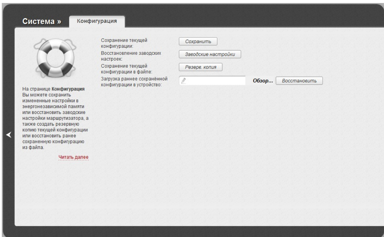
Рисунок 142. Страница Система / Конфигурация .
