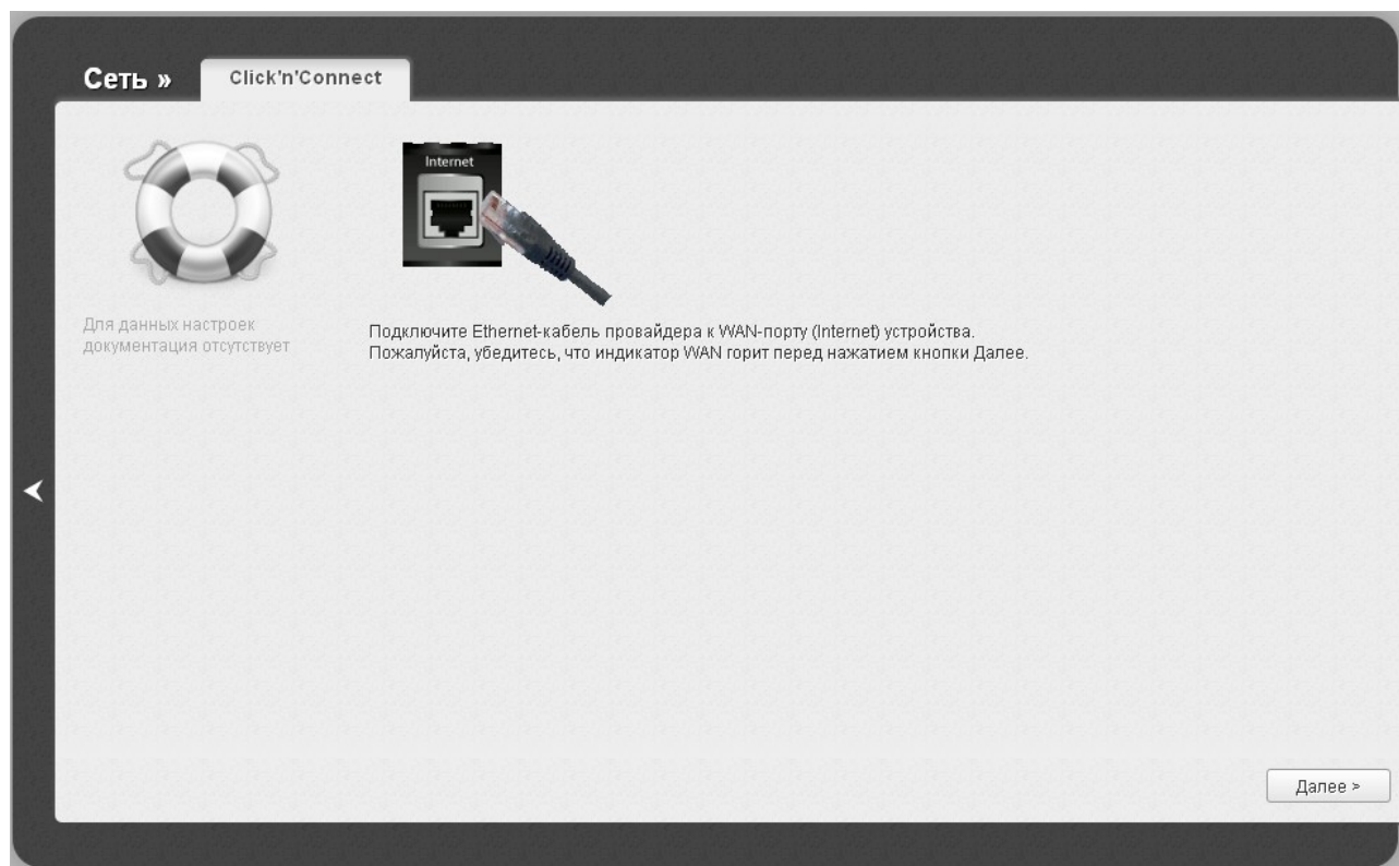
Рисунок 24. Настройка WAN-соединения.
