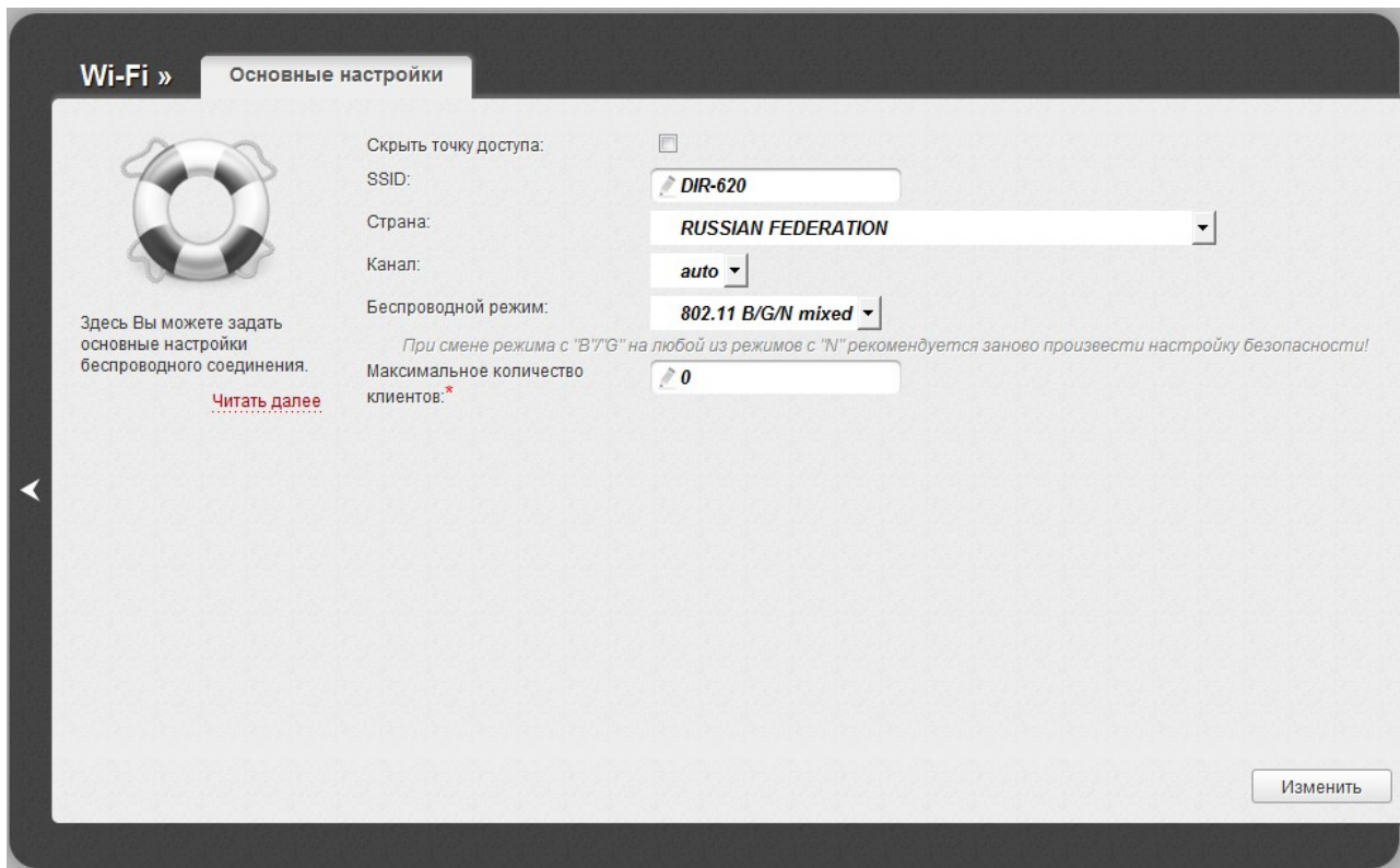
Рисунок 98. Основные настройки беспроводной локальной сети.
