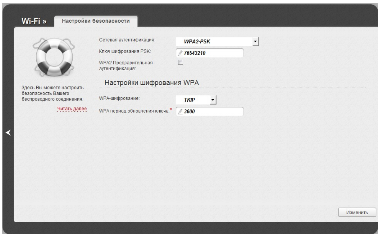
Рисунок 102. Значение WPA2-PSK в раскрывающемся списке Сетевая аутентификация .
