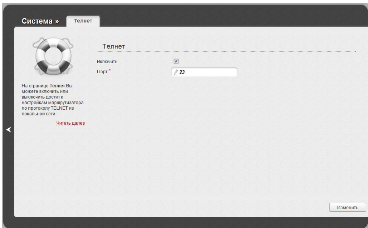
Рисунок 149. Страница Система / Телнет .
