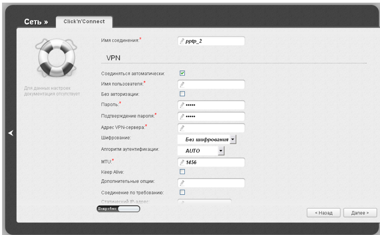
Рисунок 38. Настройка WAN-соединения типа PPTP. Экспертный режим настроек. Раздел VPN.
