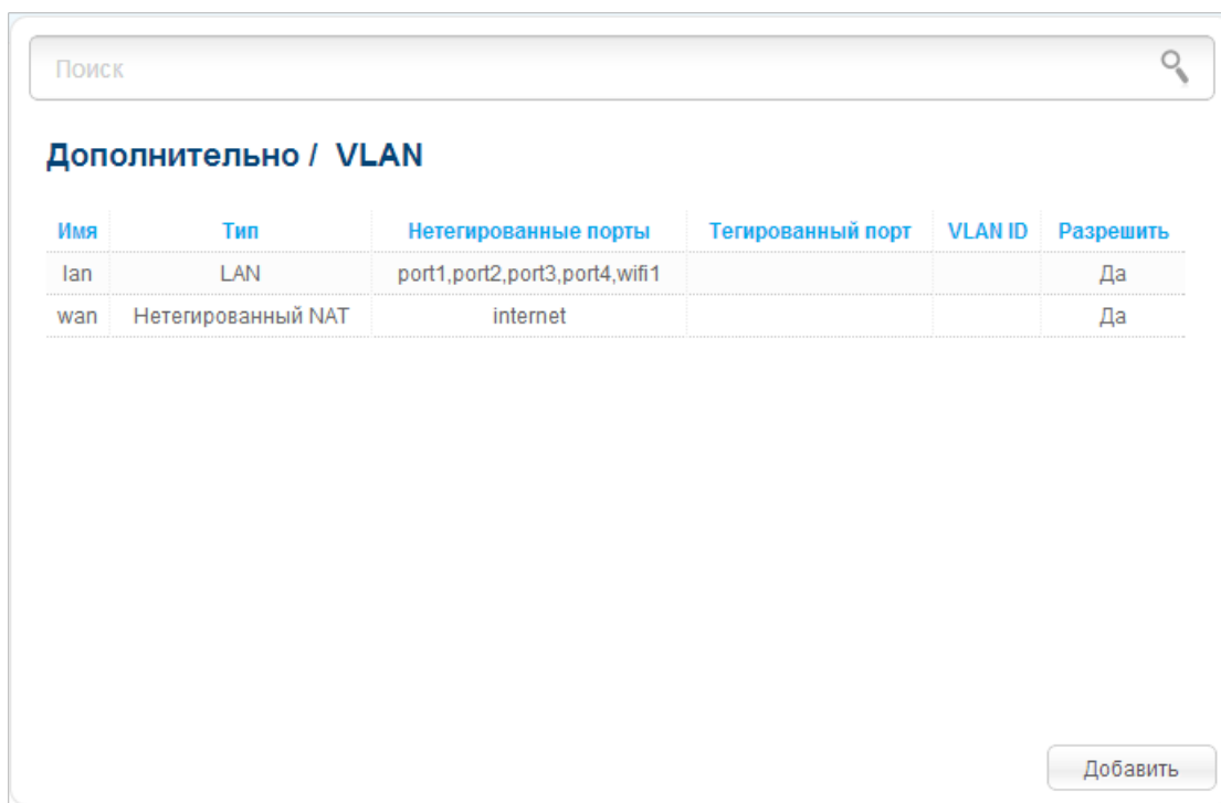
Рисунок 124. Страница Дополнительно / VLAN .
