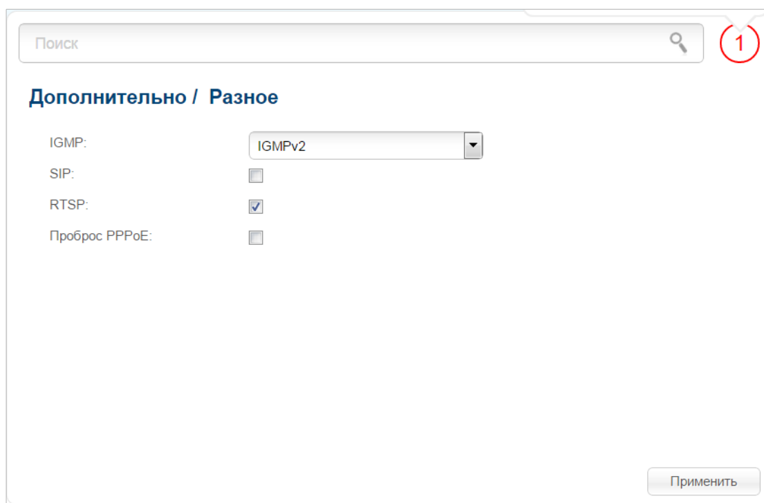
Рисунок 132. Страница Дополнительно / Разное .
