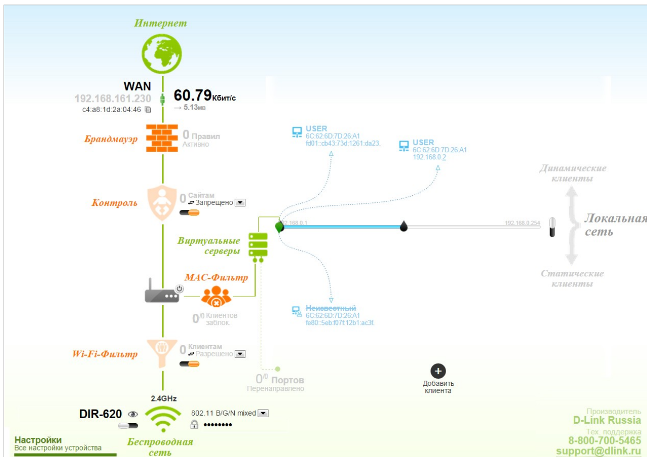
Рисунок 23. Страница Мониторинг .
