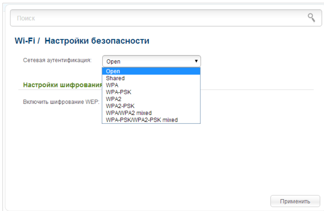
Рисунок 113. Типы аутентификации, поддерживаемые маршрутизатором.
