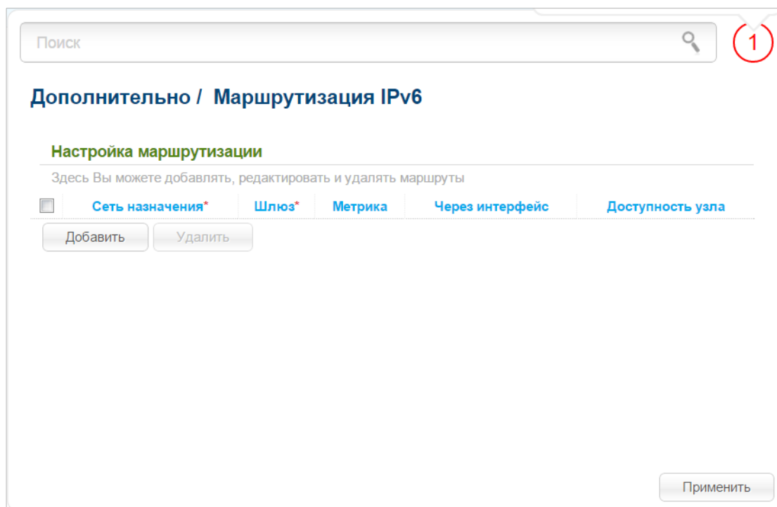
Рисунок 130. Страница Дополнительно / Маршрутизация IPv6 .
