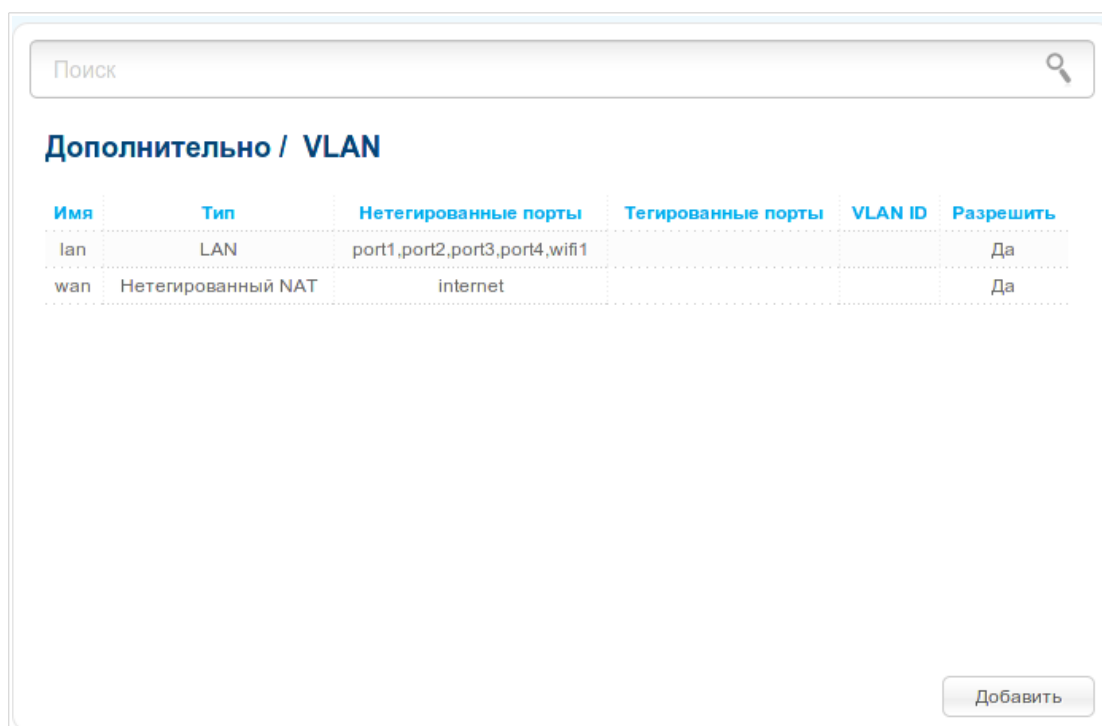
Рисунок 122. Страница Дополнительно / VLAN .
