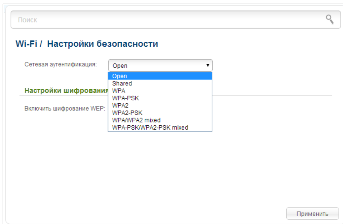
Рисунок 111. Типы аутентификации, поддерживаемые маршрутизатором.
