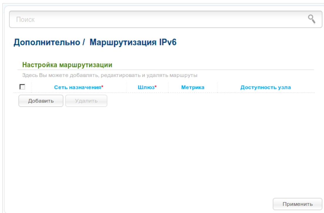
Рисунок 132. Страница Дополнительно / Маршрутизация IPv6 .
