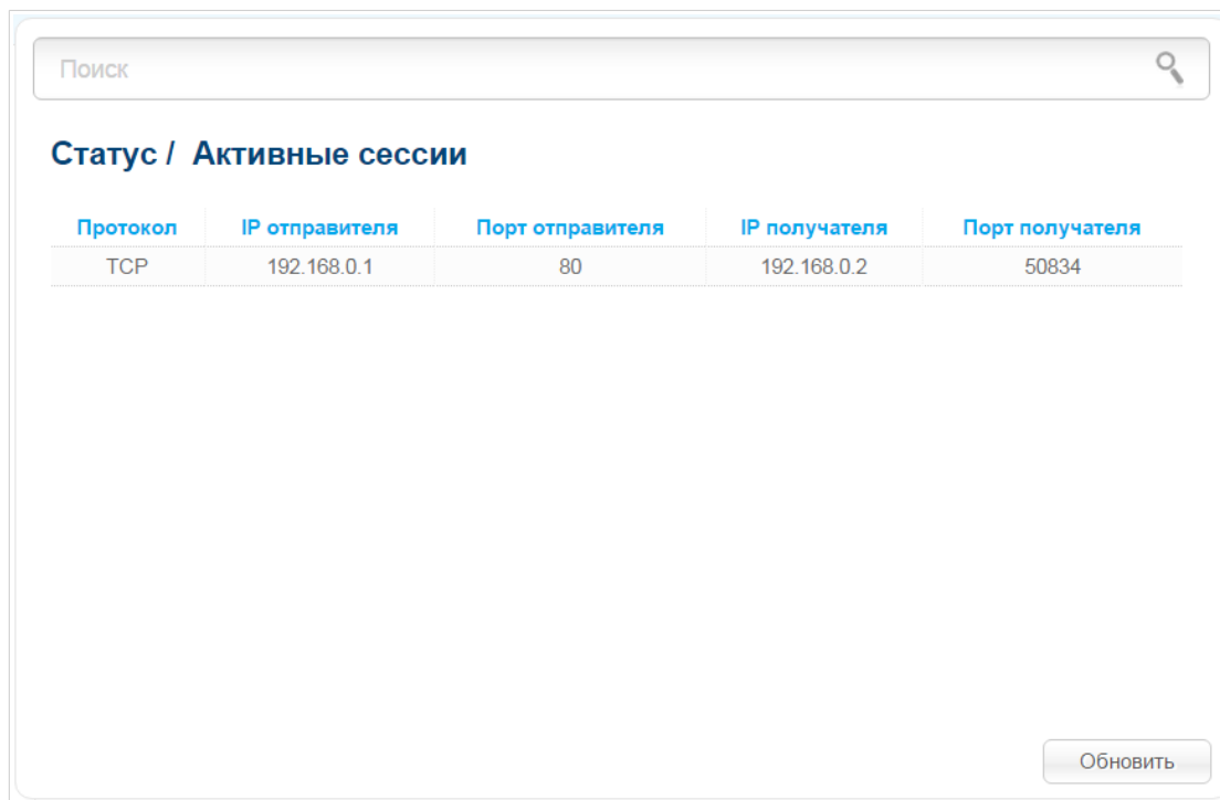
Рисунок 61. Страница Статус / Активные сессии .
