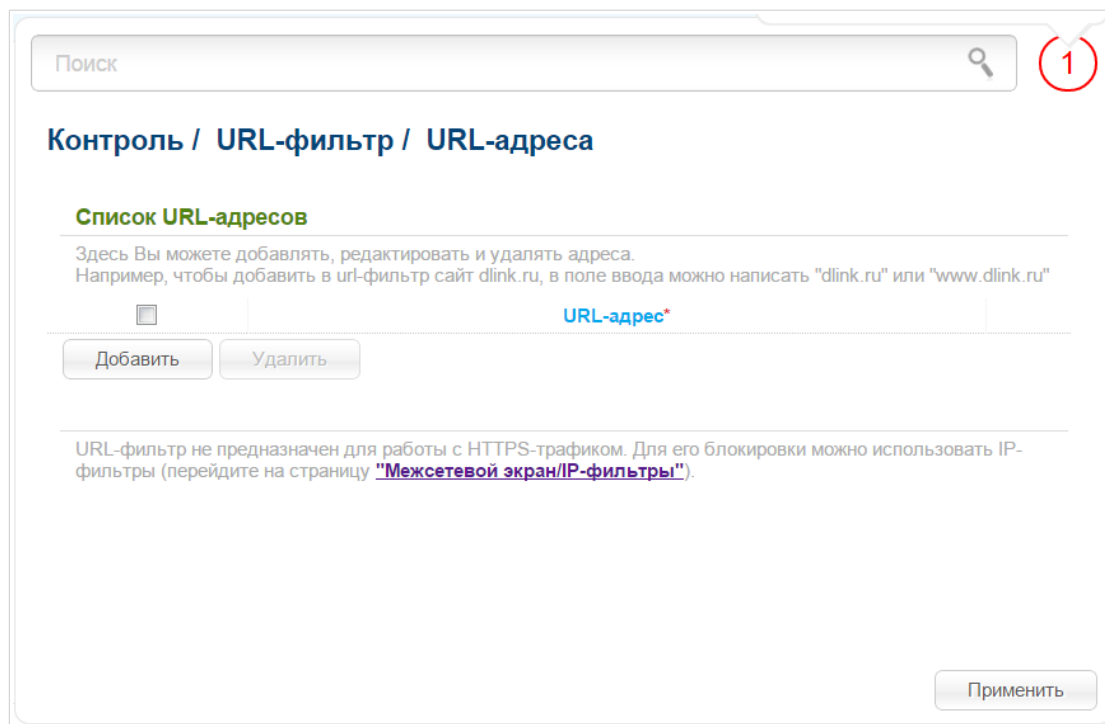
Рисунок 161. Страница Контроль / URL-фильтр / URL-адреса .
