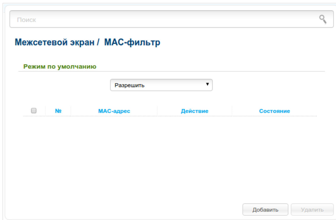
Рисунок 145. Страница Межсетевой экран / MAC-фильтр .
