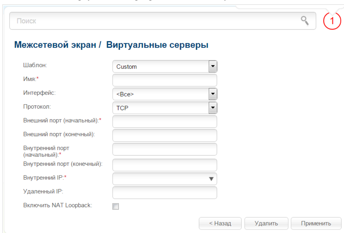
Рисунок 143. Страница добавления виртуального сервера.
