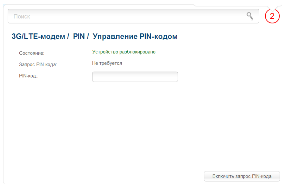
Рисунок 150. Страница 3G/LTE-модем / PIN / Управление PIN-кодом .
