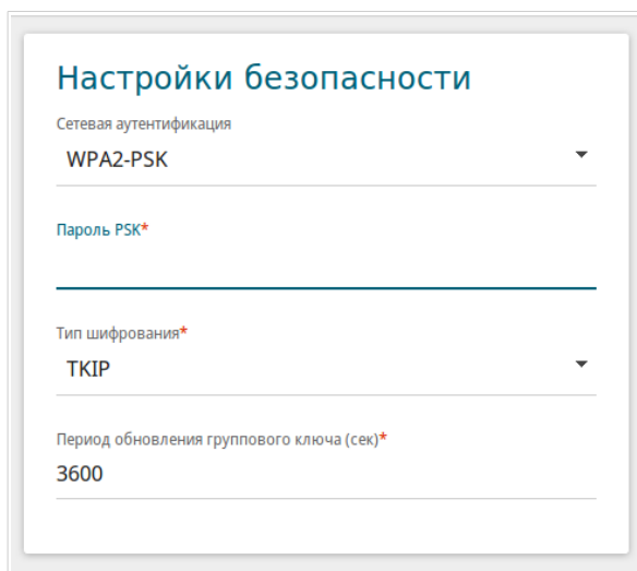
Рисунок 85. Значение WPA2-PSK в раскрывающемся списке Сетевая аутентификация .
