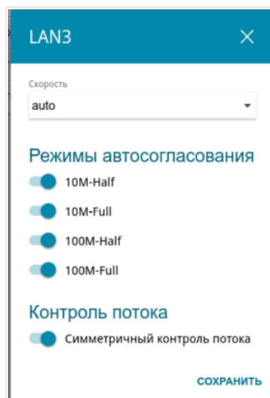
Рисунок 103. Окно изменения настроек порта маршрутизатора.
