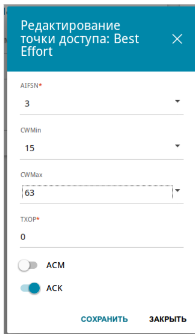
Рисунок 90. Окно для изменения параметров функции WMM.
