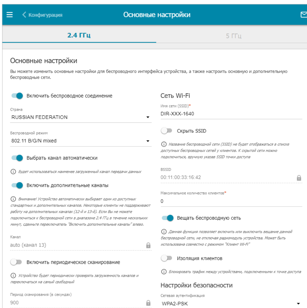
Рисунок 87. Общие настройки беспроводного соединения в диапазоне 2,4 ГГц.
