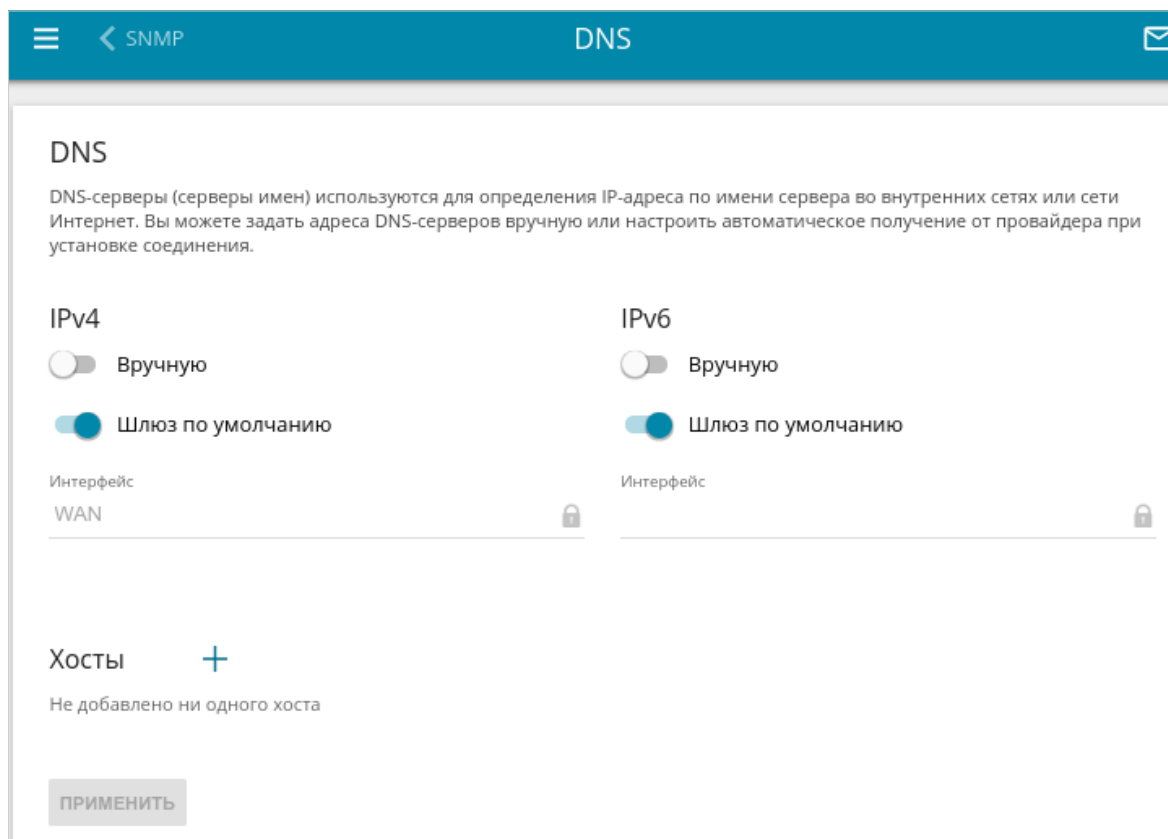
Рисунок 106. Страница Дополнительно / DNS .
