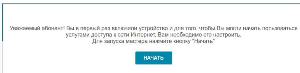
Рисунок 30. Запуск Мастера.
