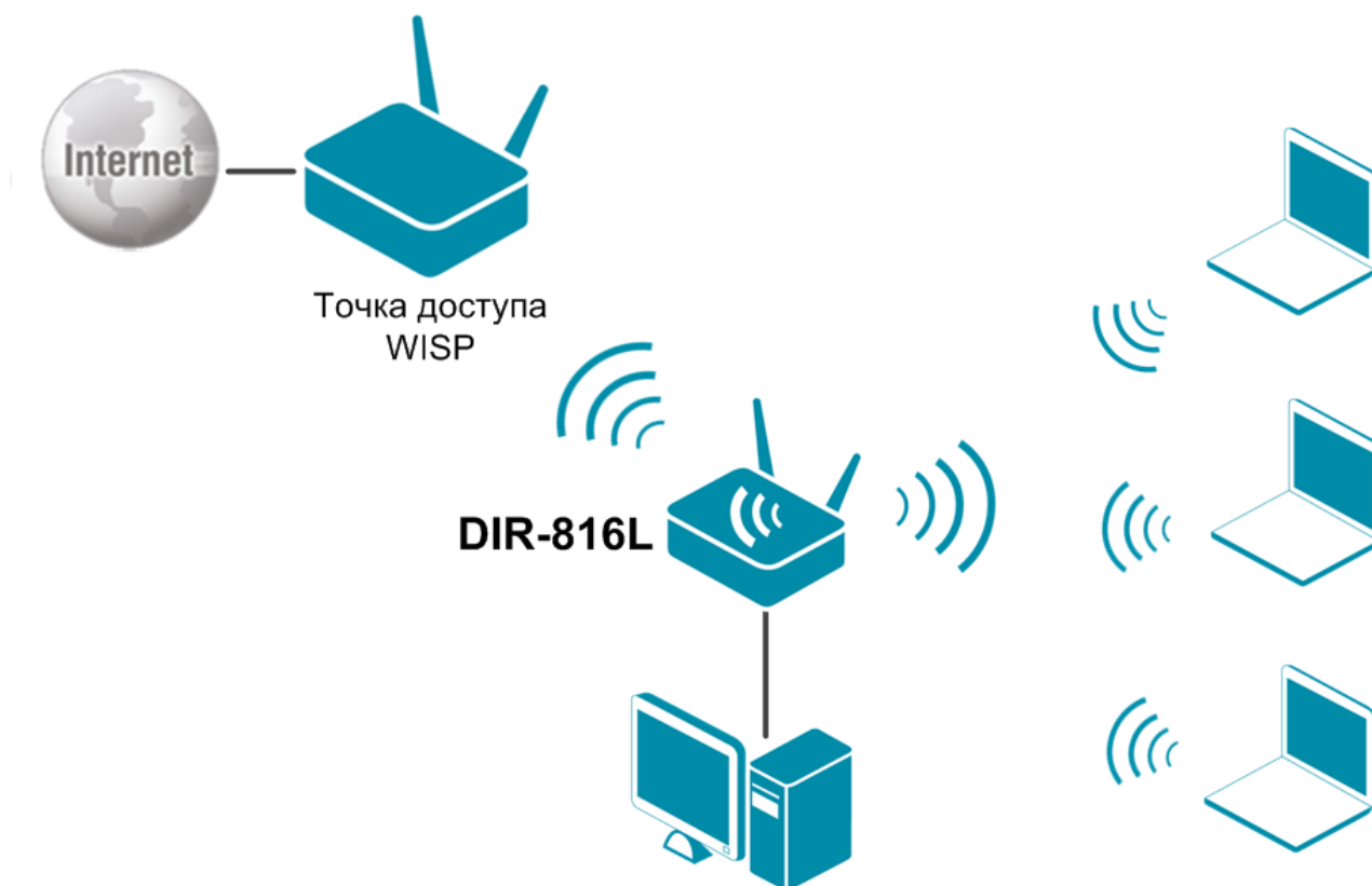
Рисунок 129. Подключение DIR-816L в режиме маршрутизатора в качестве клиента.
