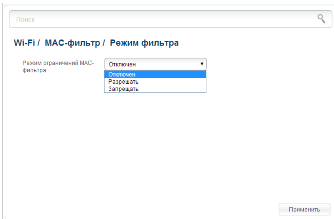
Рисунок 206. Страница для настройки MAC-фильтра для беспроводной сети.
