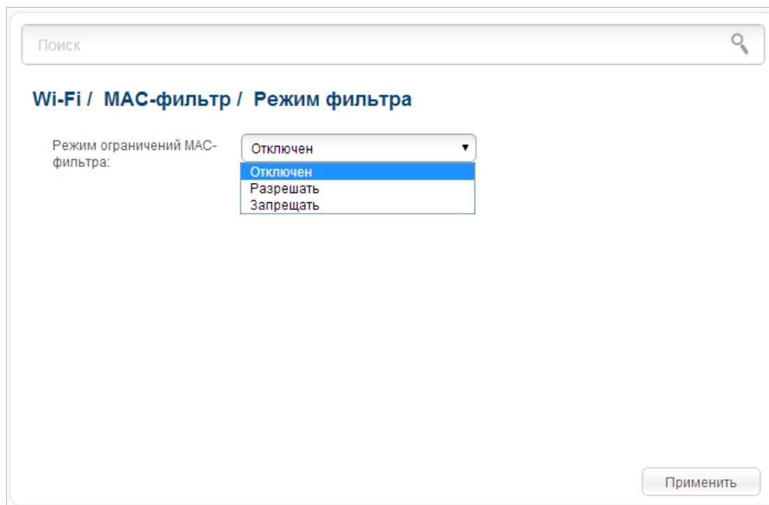
Рисунок 122. Страница для настройки MAC-фильтра для беспроводной сети.
