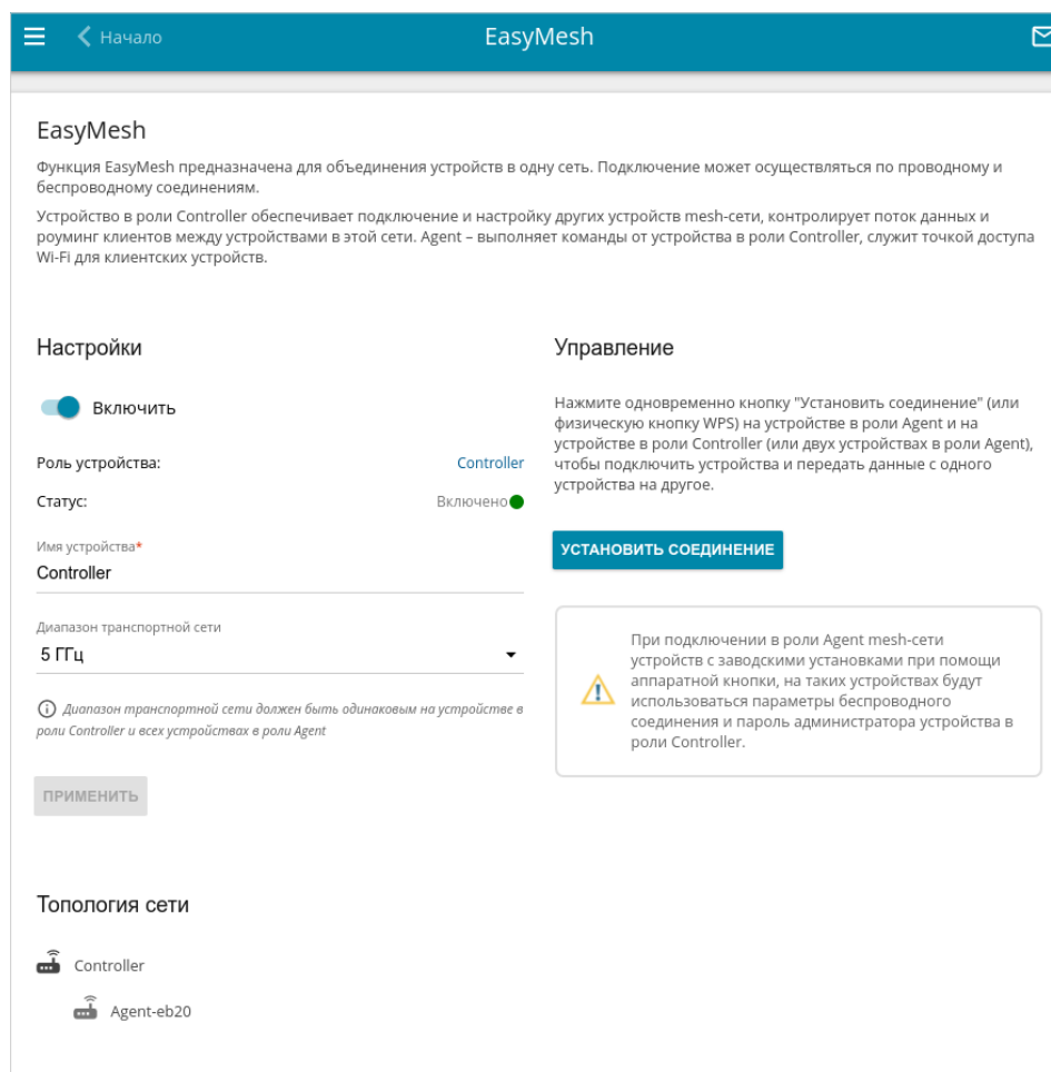
Рисунок 125. Страница Wi-Fi / EasyMesh .
