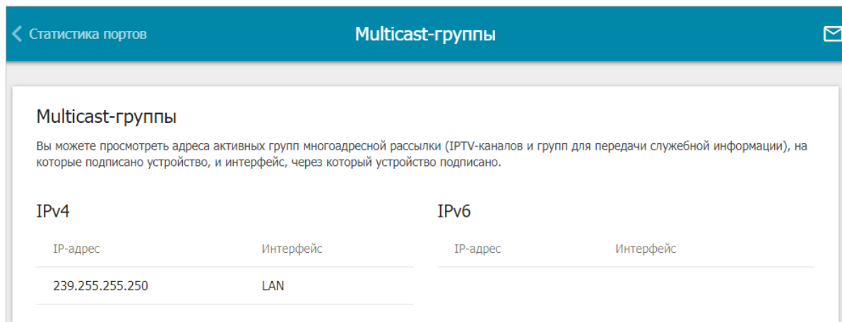
Рисунок 33. Страница Статистика / Multicast-группы .
