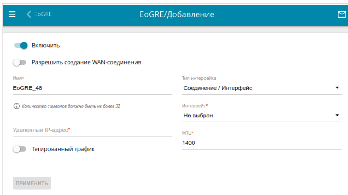
Рисунок 96. Страница добавления EoGRE-туннеля.
