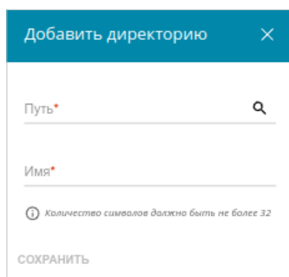
Рисунок 131. Добавление директории.
