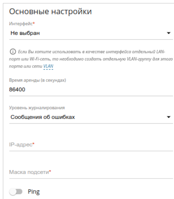
Рисунок 171. Страница добавления сервера авторизации. Раздел Основные настройки .
