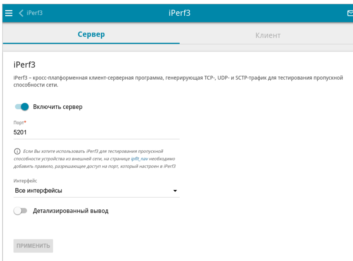
Рисунок 214. Страница Система / iPerf3 . Вкладка Сервер .
