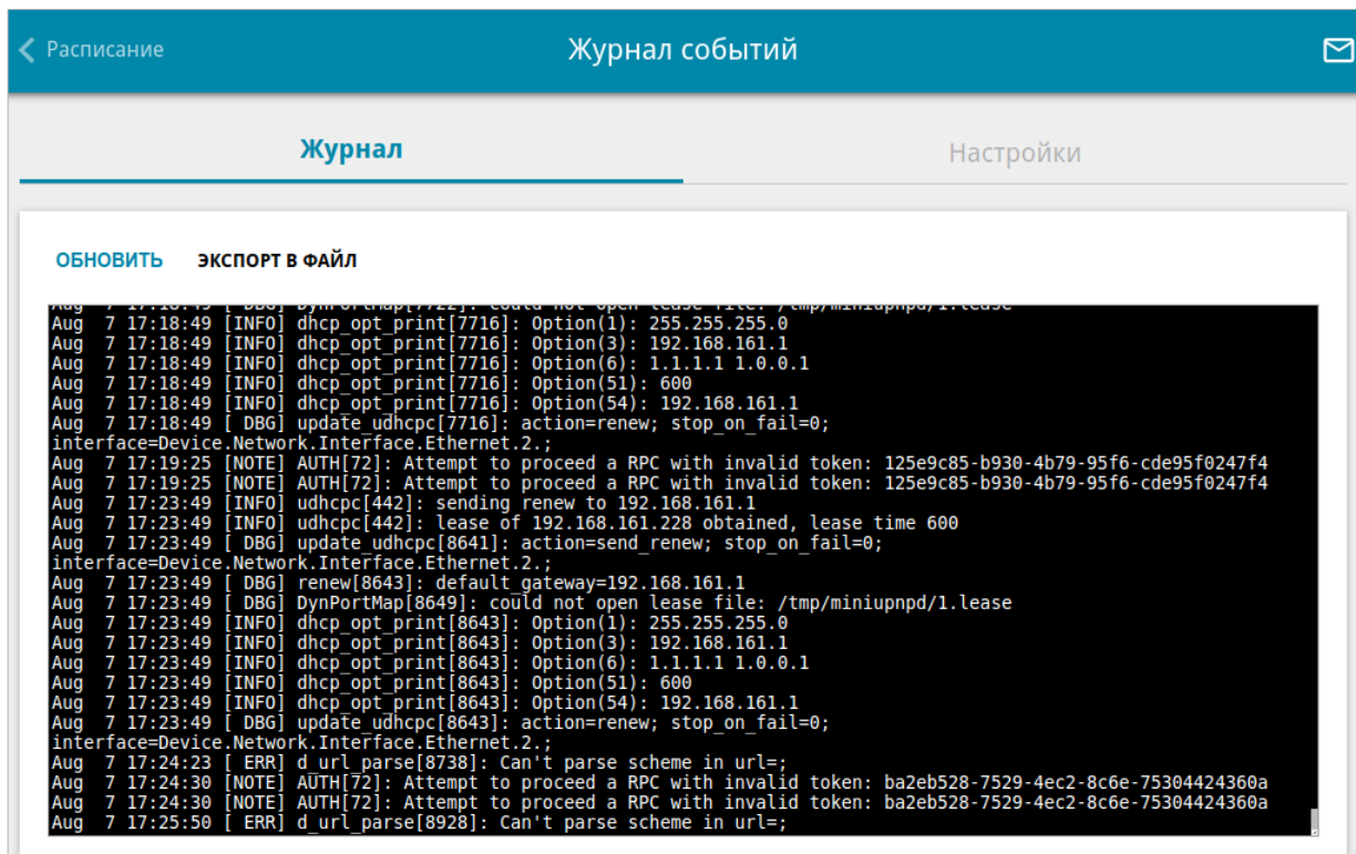
Рисунок 209. Страница Система / Журнал событий. Вкладка Журнал.
