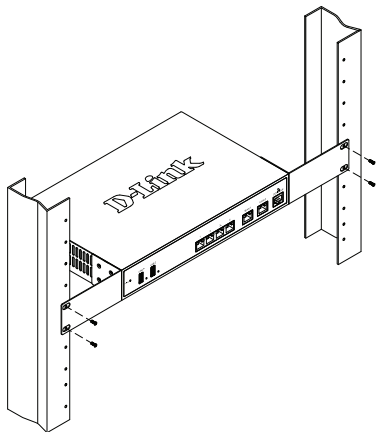
Рис.4 Установка маршрутизатора в стандартную стойку
