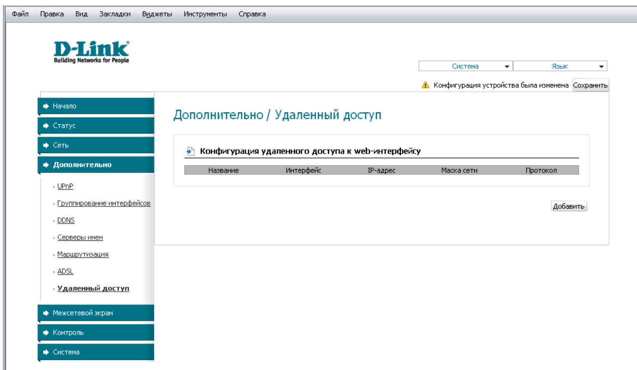
Рисунок 38. Страница Дополнительно / Удаленный доступ .
