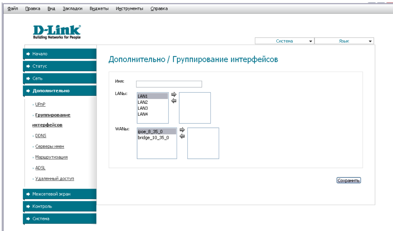
Рисунок 31. Страница добавления правила для группирования интерфейсов.
