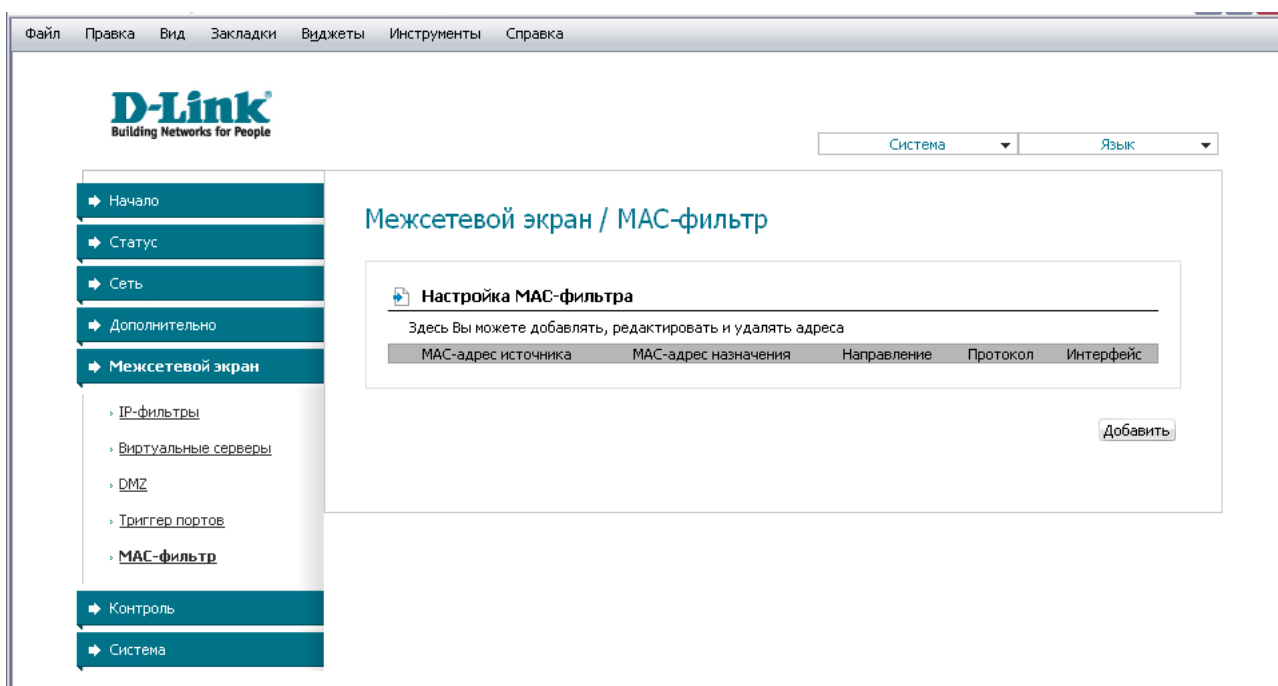
Рисунок 47. Страница Межсетевой экран / MAC-фильтр .
