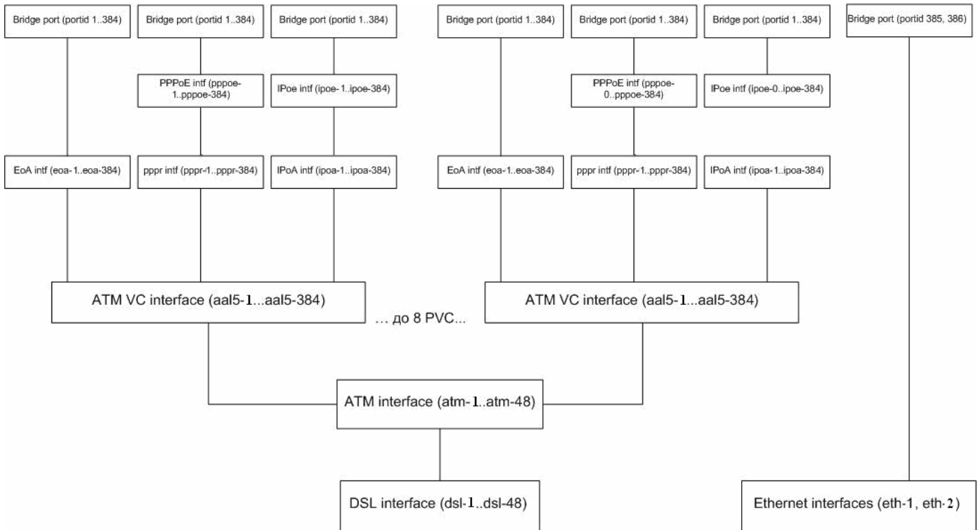
Рисунок 2-1. Логическая структура интерфейсов DAS-3248
