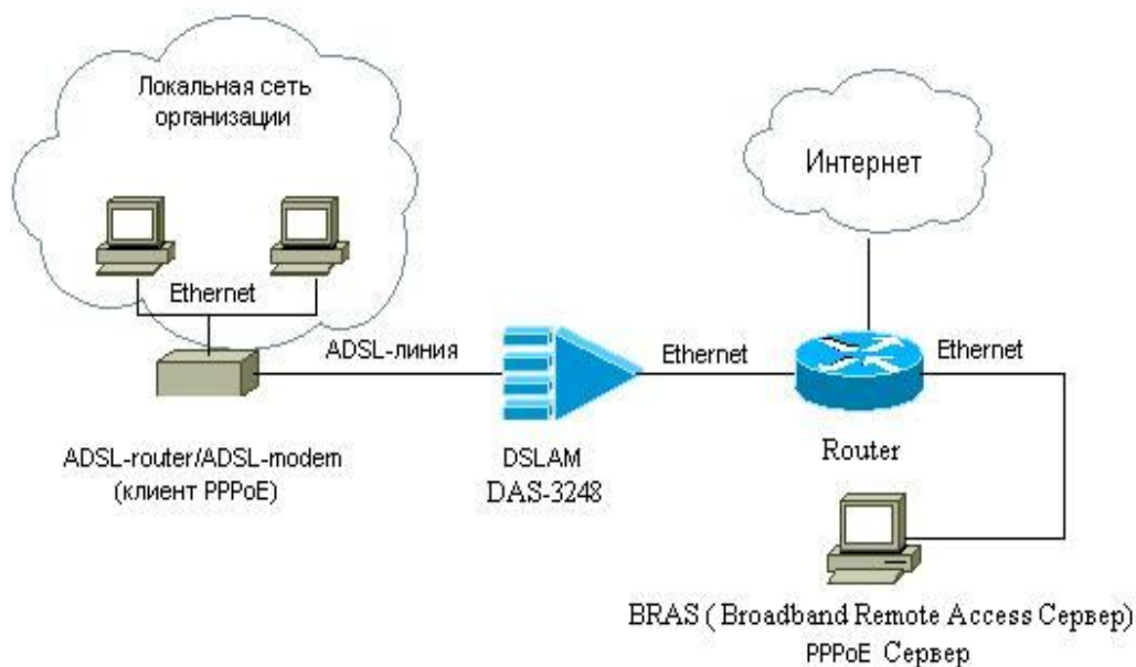
Рисунок 4-30. Схема ADSL доступа по PPPoE технологии
