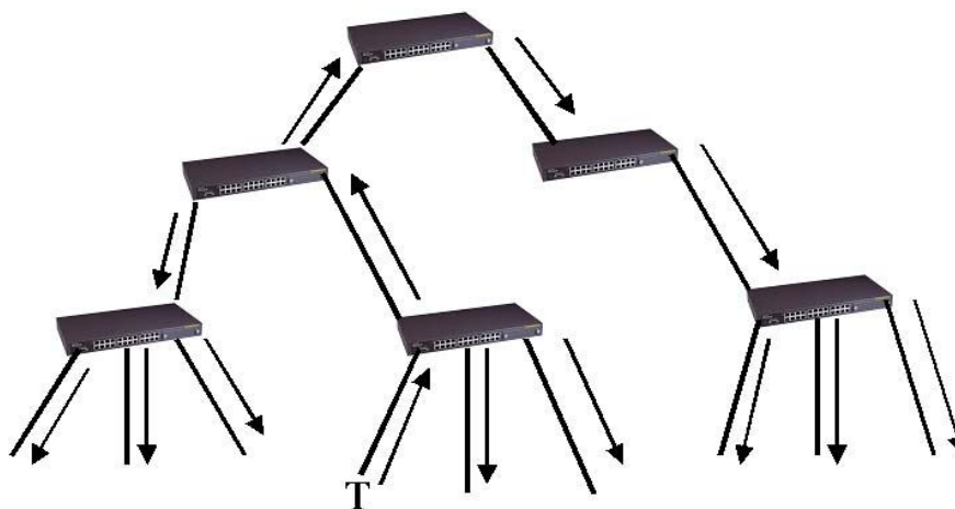
Рисунок 8-15. Новый механизм изменения топологии. Отправитель BPDU с битом TC непосредственно распространяет информацию об изменении топологии через всю сеть.
