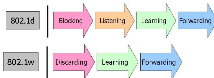
Рисунок 8-5. Состояния портов протоколов STP 802.1D и RSTP 802.1w.
