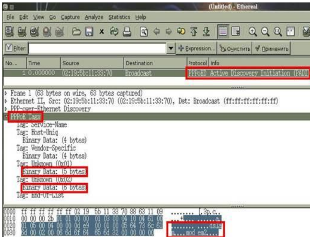
Рисунок 4-35. Перехват измененного пакета с использованием PPPoE Relay
