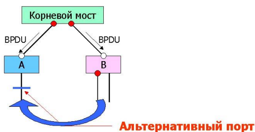
Рисунок 8-8. Альтернативный порт.
