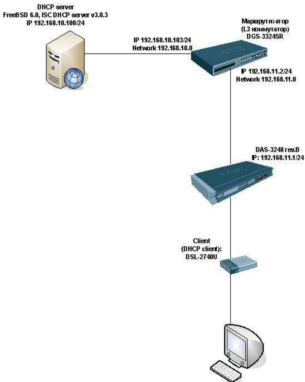
Рисунок 4-32. Пример схемы доступа с использованием DHCP Relay
