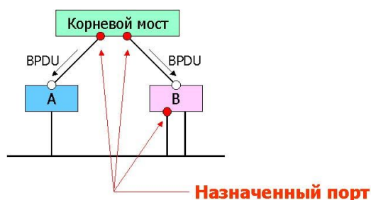
Рисунок 8-7. Назначенный порт.
