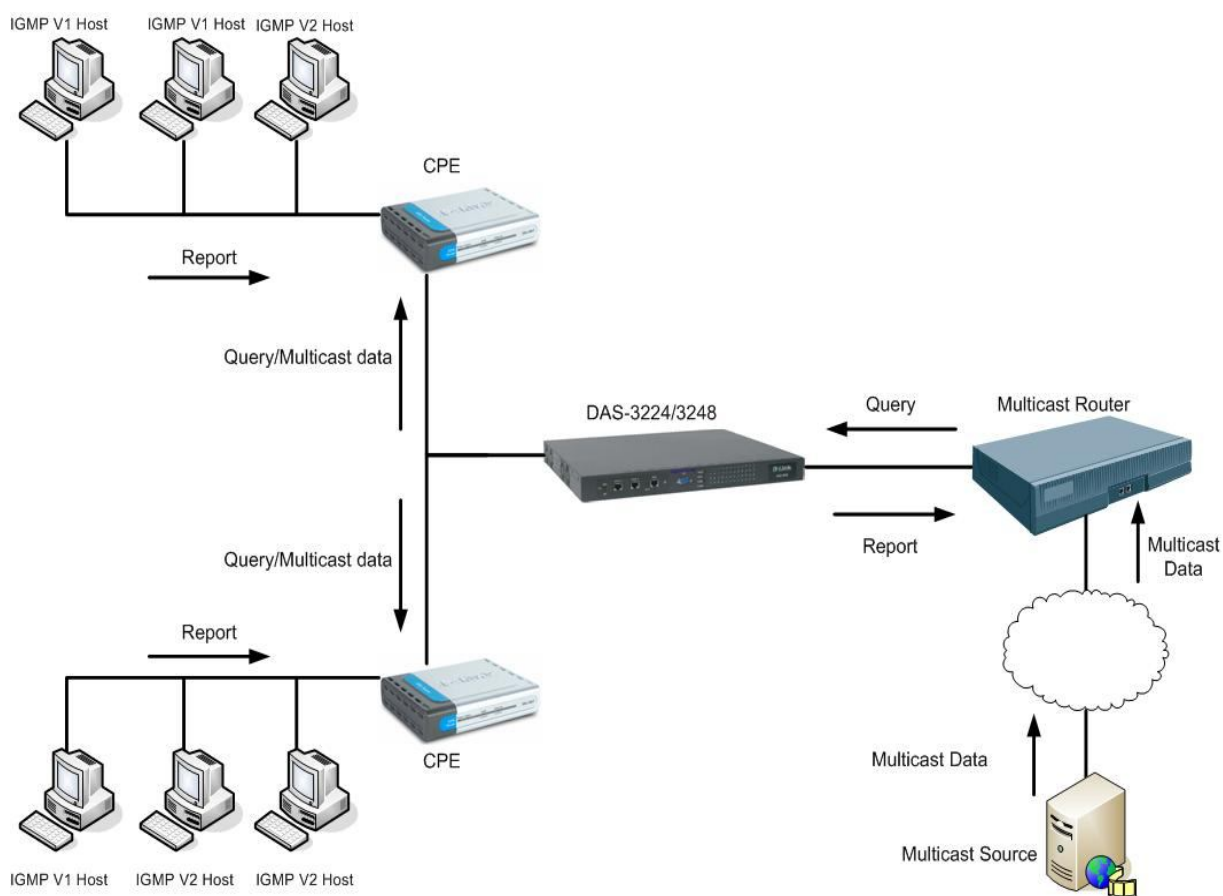
Рисунок 7-3: IGMP Snooping
