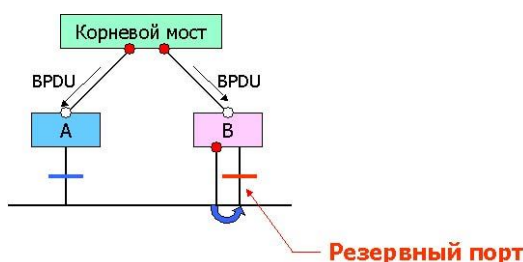
Рисунок 8-9. Резервный порт.
