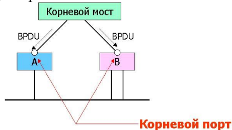
Рисунок 8-6. Корневой порт
