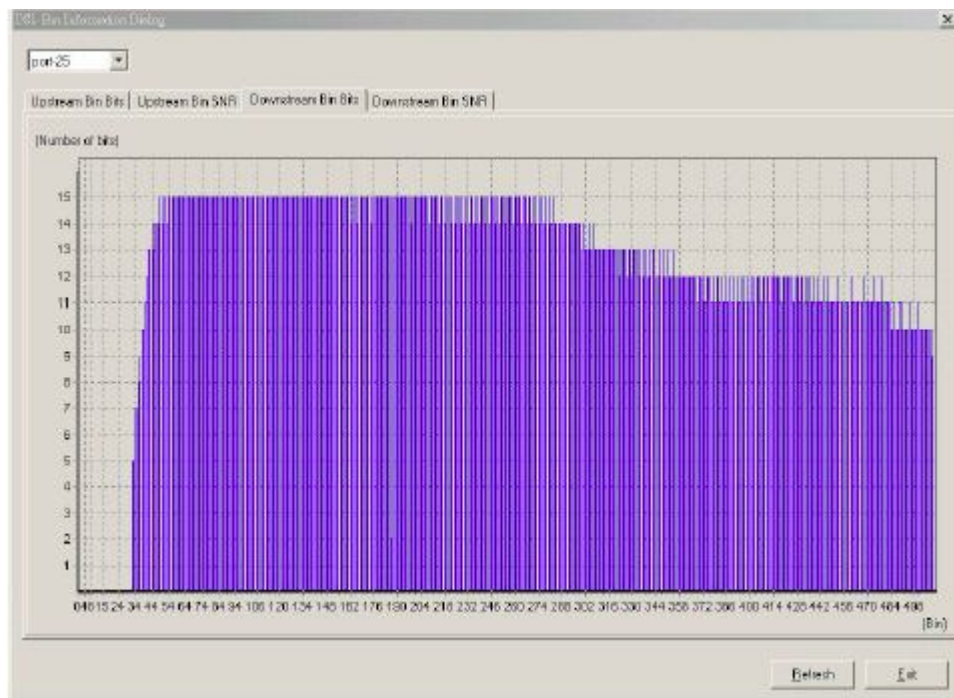
Рисунок 3-83. Диалог DSL Bin Information
