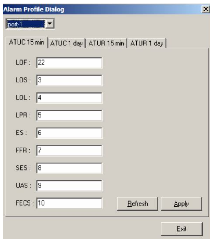
Рисунок 3-22. Диалог конфигурирования тревожного профиля (Alarm Profile)
