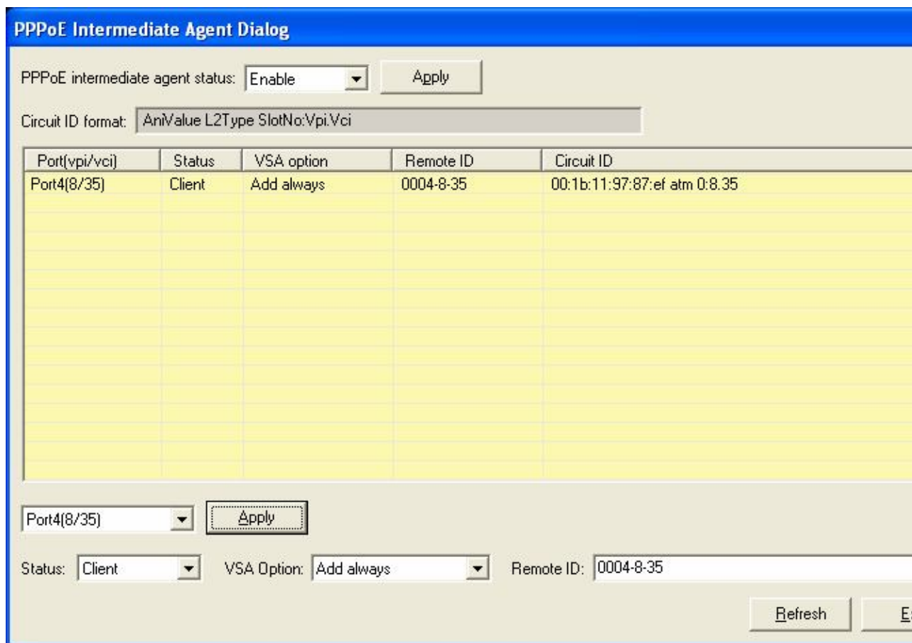
Рисунок 3-44. Диалог настройки функции PPPoE Intermediate Agent (PIA)
