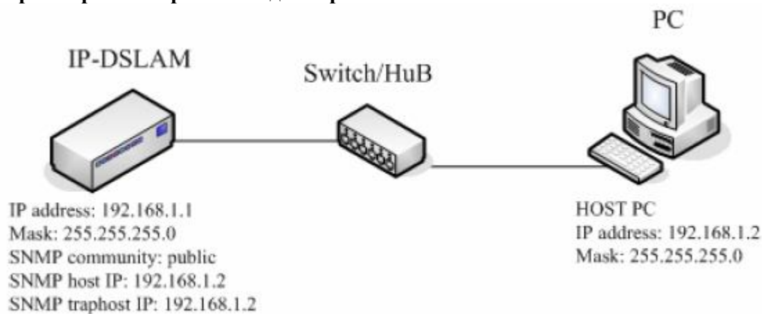
Рисунок 2-7. Пример настройки параметров соединения NE с клиентами LCT
