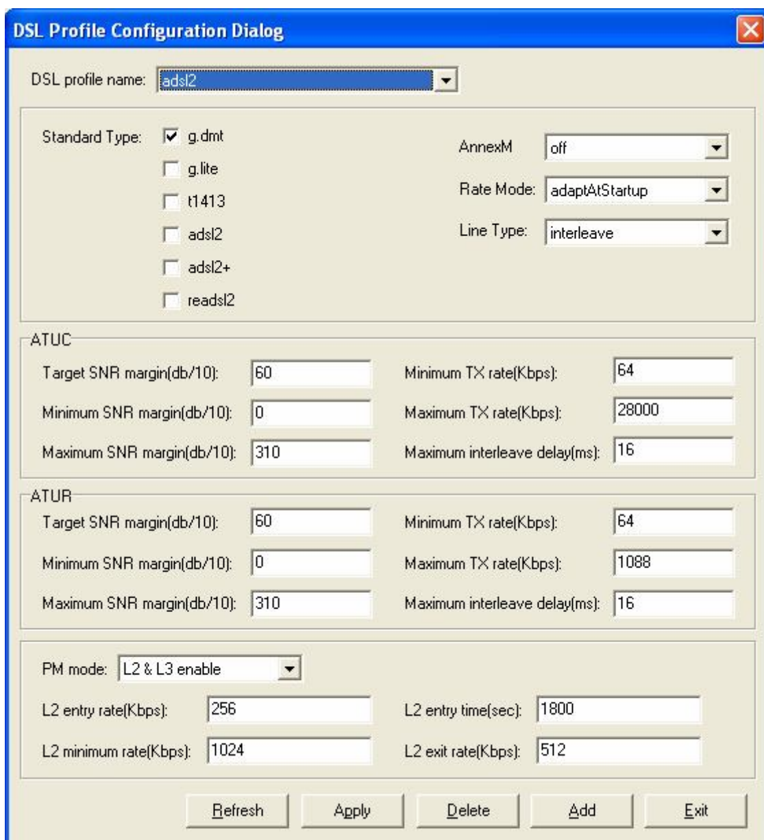
Рисунок 3-19. Диалог настройки профиля ADSL (Line Profile Configuration)
