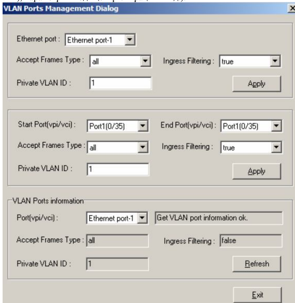
Рисунок 3-35. Диалог управления параметрами VLAN на отдельных портах
