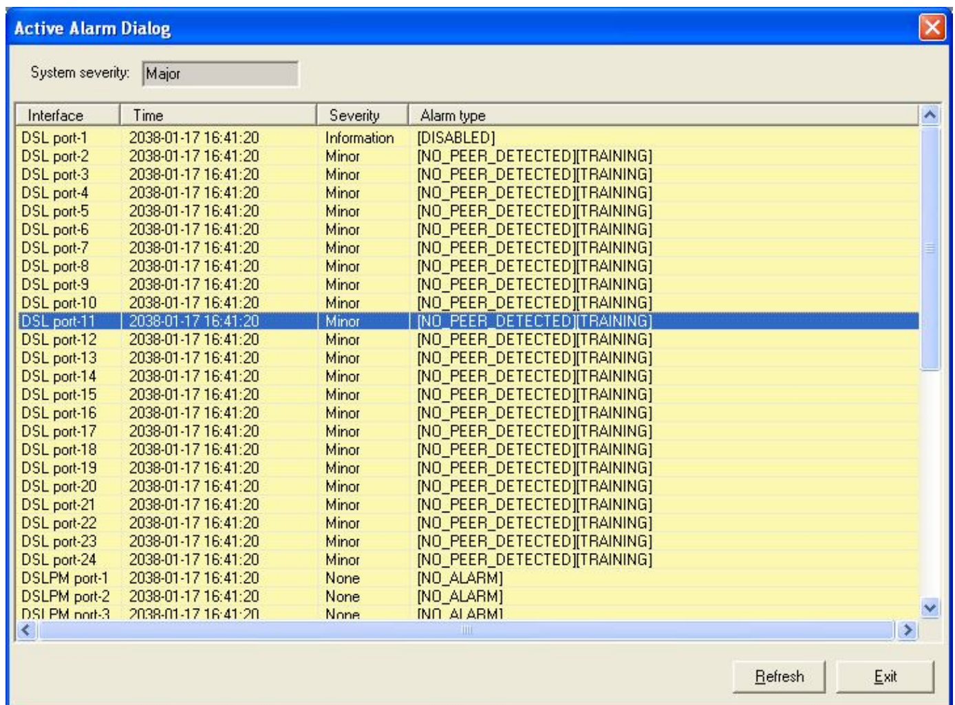
Рисунок 3-69. Диалог диагностических сообщений DSLSAM
