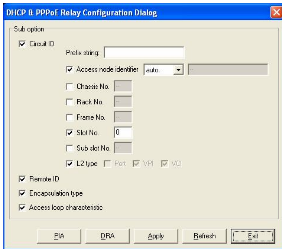
Рисунок 3-42. Диалог настройки функции DHCP& PPPoE Relay.
