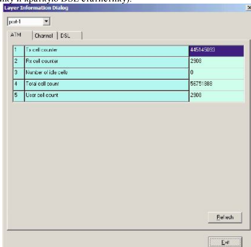
Рисунок 3-64. Диалог статуса транспортного уровня
