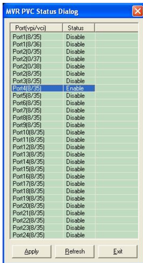
Рисунок 3-48. Диалог включения функции мультикаст VLAN на портах устройства
