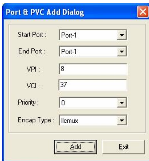
Рисунок 3-18. Диалог добавления нового PVC.
