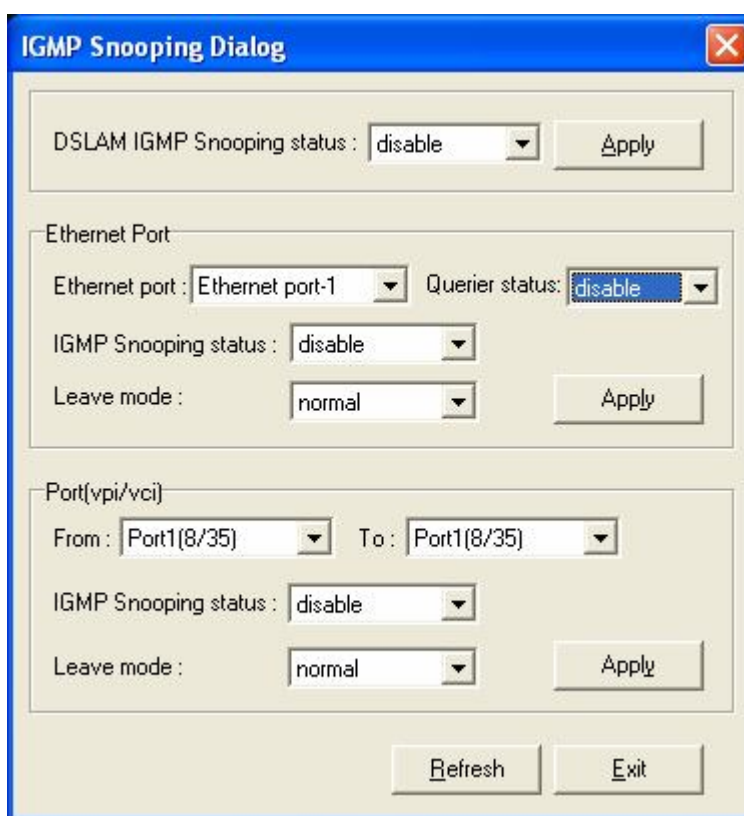
Рисунок 3-40. Диалог настройки IGMP Snooping
