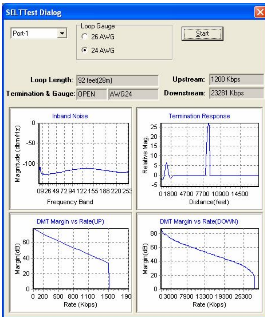
Рисунок 3-84. Диалог SELT теста
