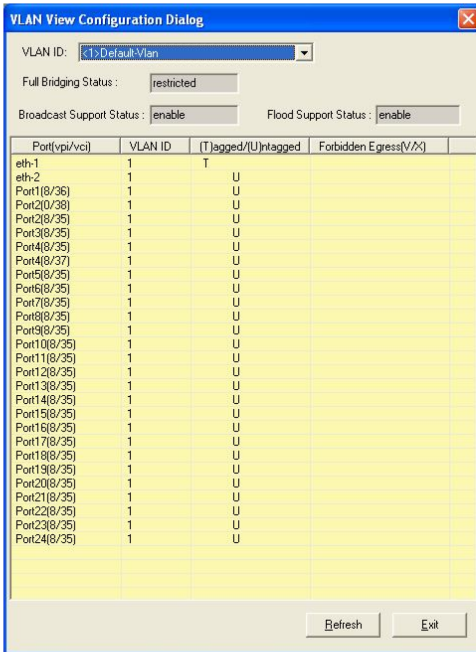
Рисунок 3-33. Диалог просмотра параметров VLAN
