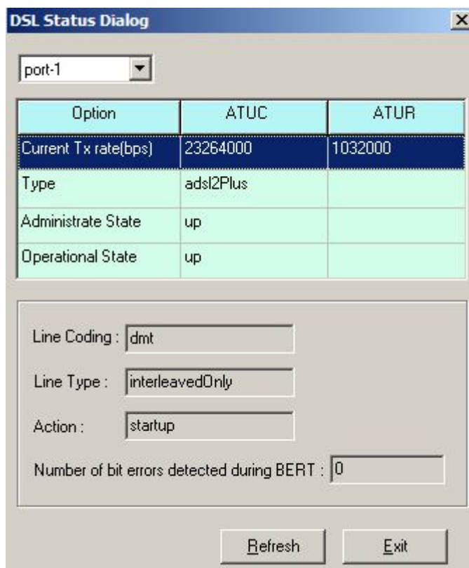
Рисунок 3-63. Диалог статуса ADSL линии
