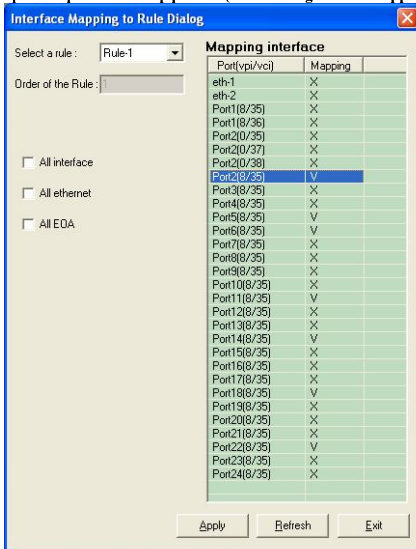
Рисунок 3-60. Диалог таблицы прикрепленных к интерфейсам правил
