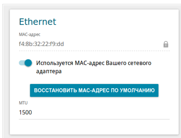
Рисунок 71. Страница добавления соединения типа PPPoE. Раздел Ethernet.
