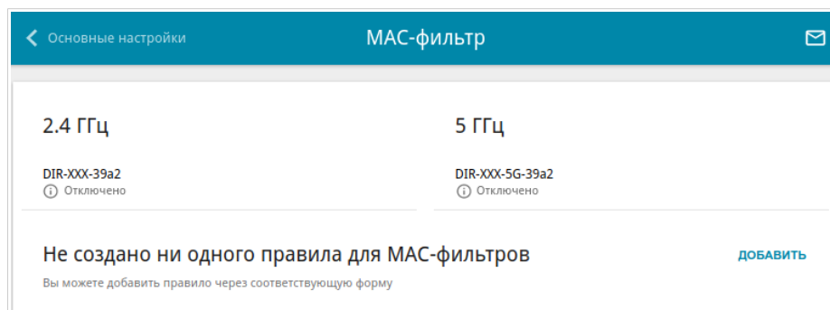
Рисунок 110. Страница для настройки MAC-фильтра для беспроводной сети.
