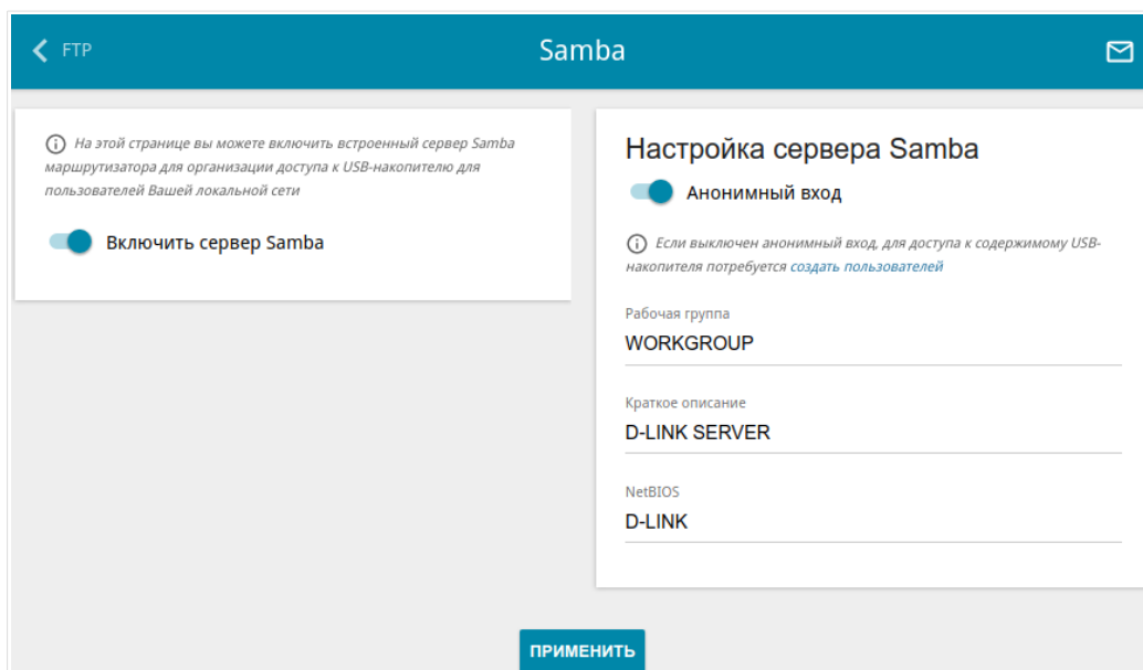
Рисунок 117. Страница USB-накопитель / Samba .
