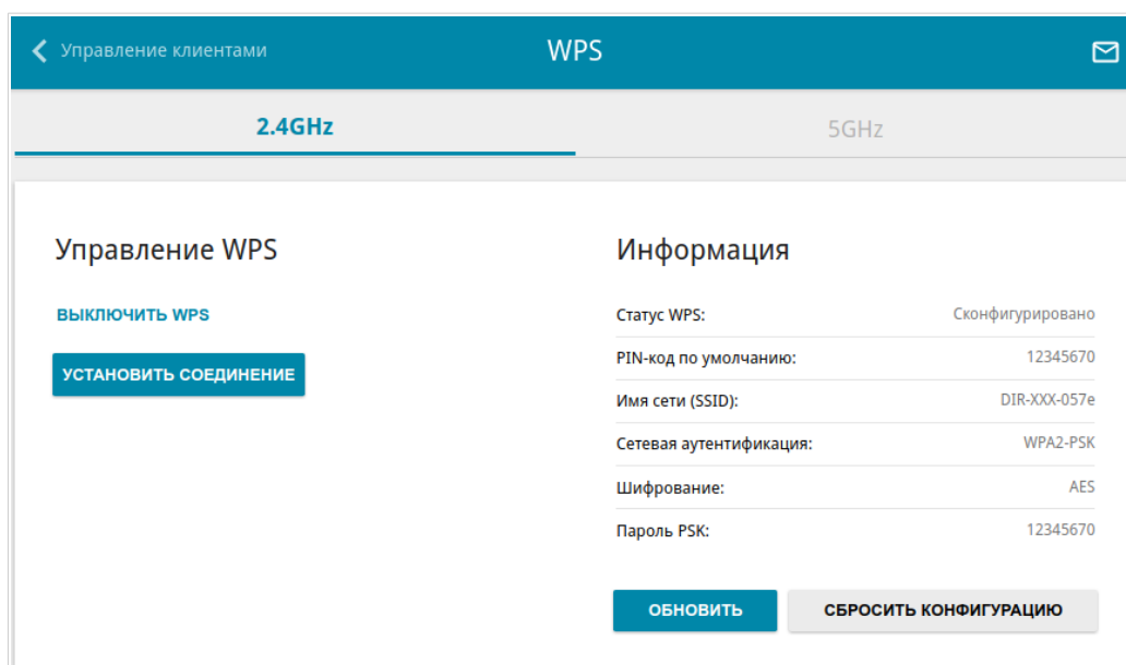
Рисунок 103. Страница для настройки функции WPS.
