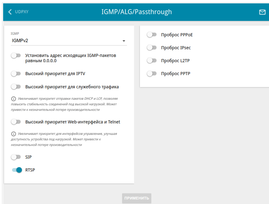
Рисунок 151. Страница Дополнительно / IGMP/ALG/Passthrough.
