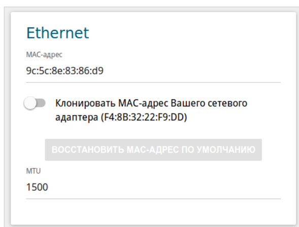
Рисунок 62. Страница добавления соединения типа Статический IPv4 . Раздел Ethernet .
