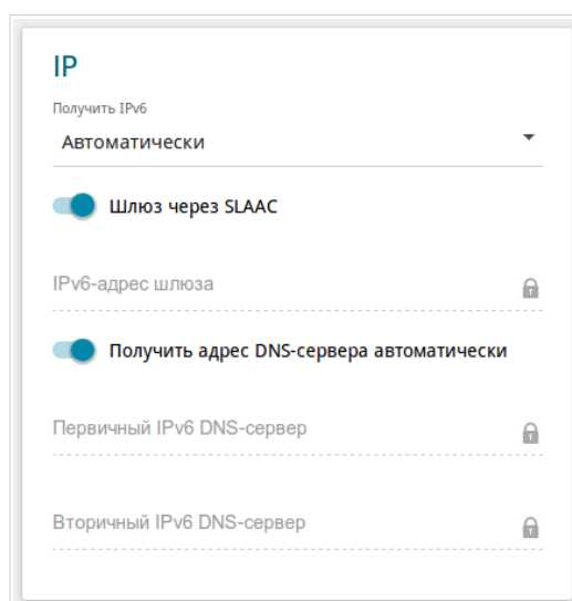
Рисунок 80. Страница добавления соединения типа PPPoE IPv6 . Раздел IP .
