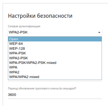
Рисунок 98. Типы аутентификации, поддерживаемые маршрутизатором.
