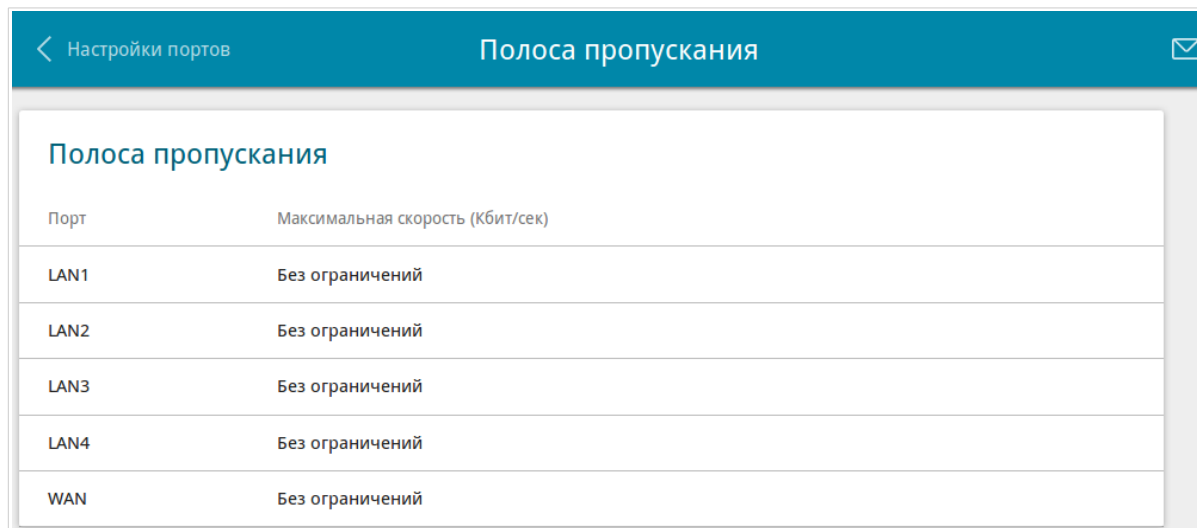
Рисунок 139. Страница Дополнительно / Полоса пропускания .
