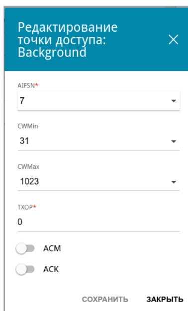
Рисунок 105. Окно для изменения параметров функции WMM.
