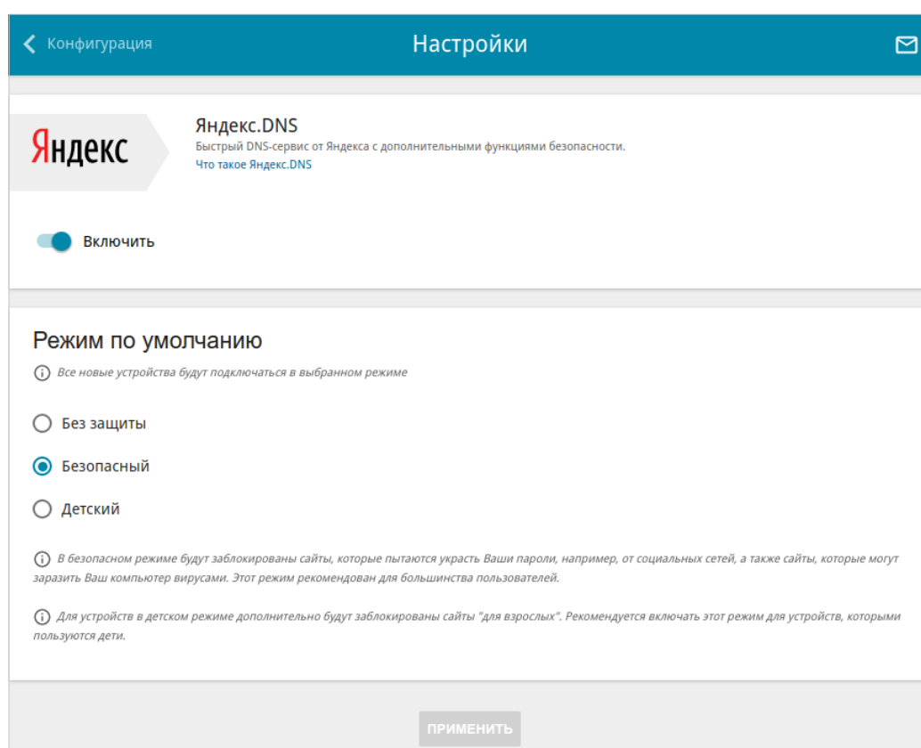
Рисунок 175. Страница Яндекс.DNS / Настройки .
