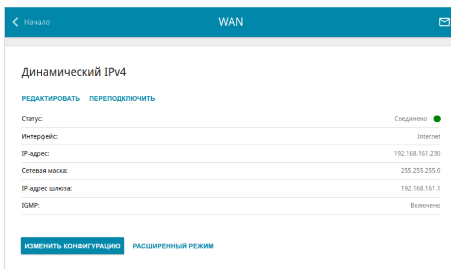
Рисунок 59. Страница Настройка соединений / WAN . Упрощенный режим.
