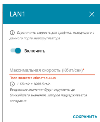
Рисунок 140. Окно для настройки ограничения скорости.
