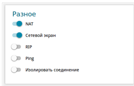
Рисунок 76. Страница добавления соединения типа PPTP . Раздел Разное .
