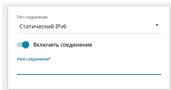
Рисунок 66. Страница добавления соединения типа Статический IPv6 . Выбор типа соединения.
