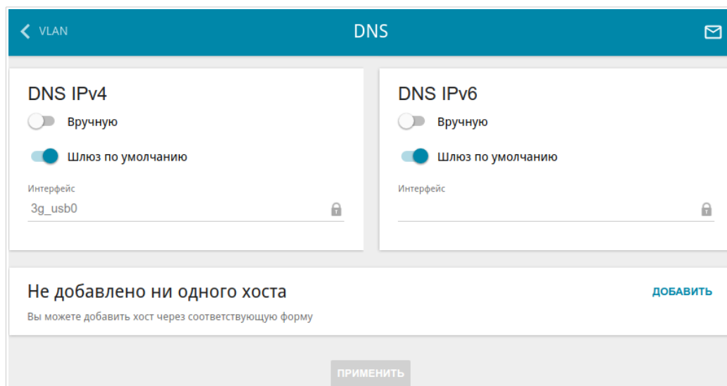
Рисунок 133. Страница Дополнительно / DNS .
