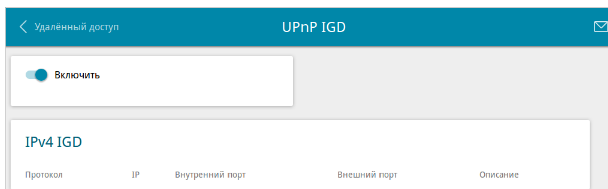
Рисунок 148. Страница Дополнительно / UPnP IGD .
