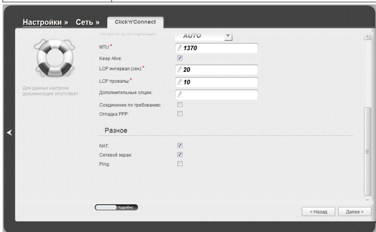
Рисунок 56. Настройка WAN-соединения типа 3G. Экспертный режим настроек. Раздел Разное .
