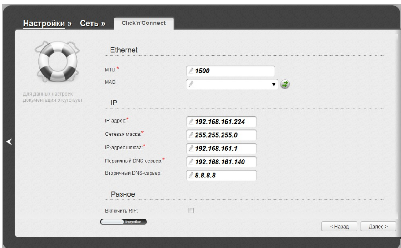
Рисунок 42. Настройка WAN-соединения типа PPTP + Статический IP. Экспертный режим настроек. Раздел Ethernet .
