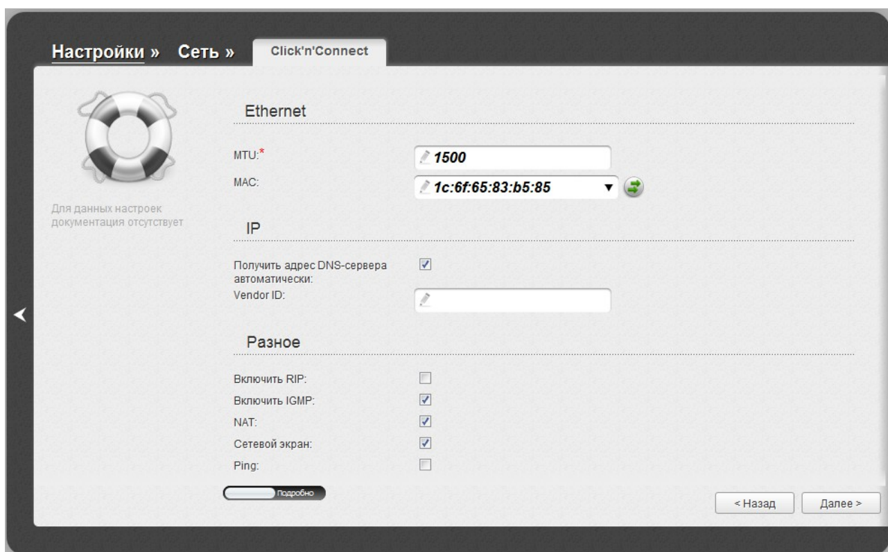
Рисунок 49. Настройка WAN-соединения типа PPTP + Динамический IP. Экспертный режим настроек. Раздел Ethernet .
