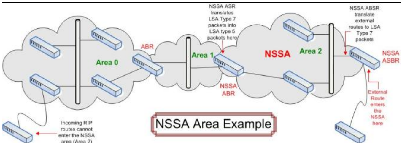
Figure 5-42 NSSA Area example
