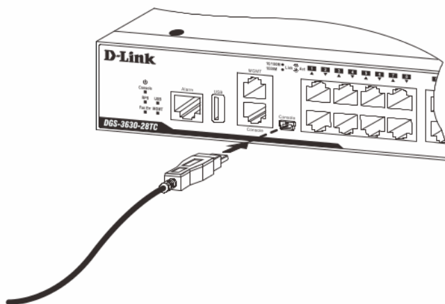
Рисунок 7 — Подключение консольного кабеля к порту mini-USB коммутатора
