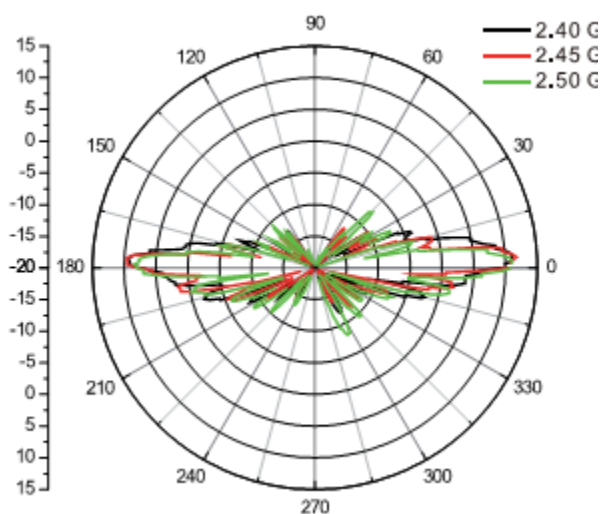
Вертикальная ДНА
