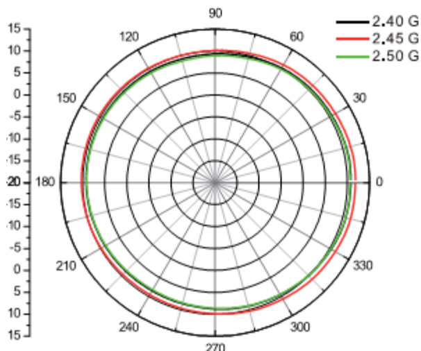
Горизонтальная ДНА
