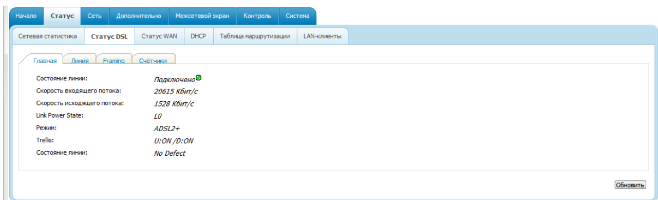
Рисунок 38. Страница Статус / Статус DSL.
