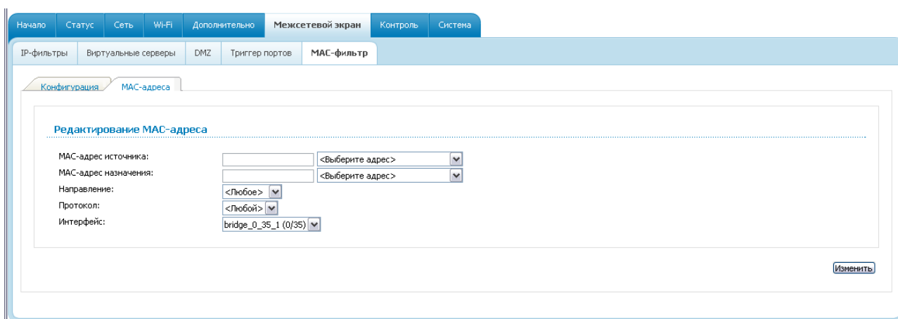
Рисунок 92. Страница добавления правила фильтрации на основе MAC-адресов.
