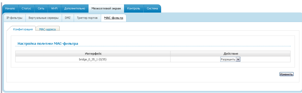
Рисунок 90. Страница Межсетевой экран / MAC-фильтр . Закладка Конфигурация .
