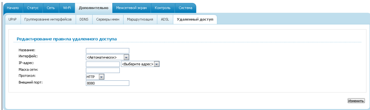
Рисунок 82. Страница добавления правила удаленного доступа.
