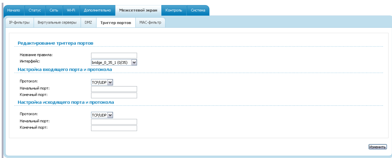
Рисунок 89. Страница добавления правила для функции Port Triggering.
