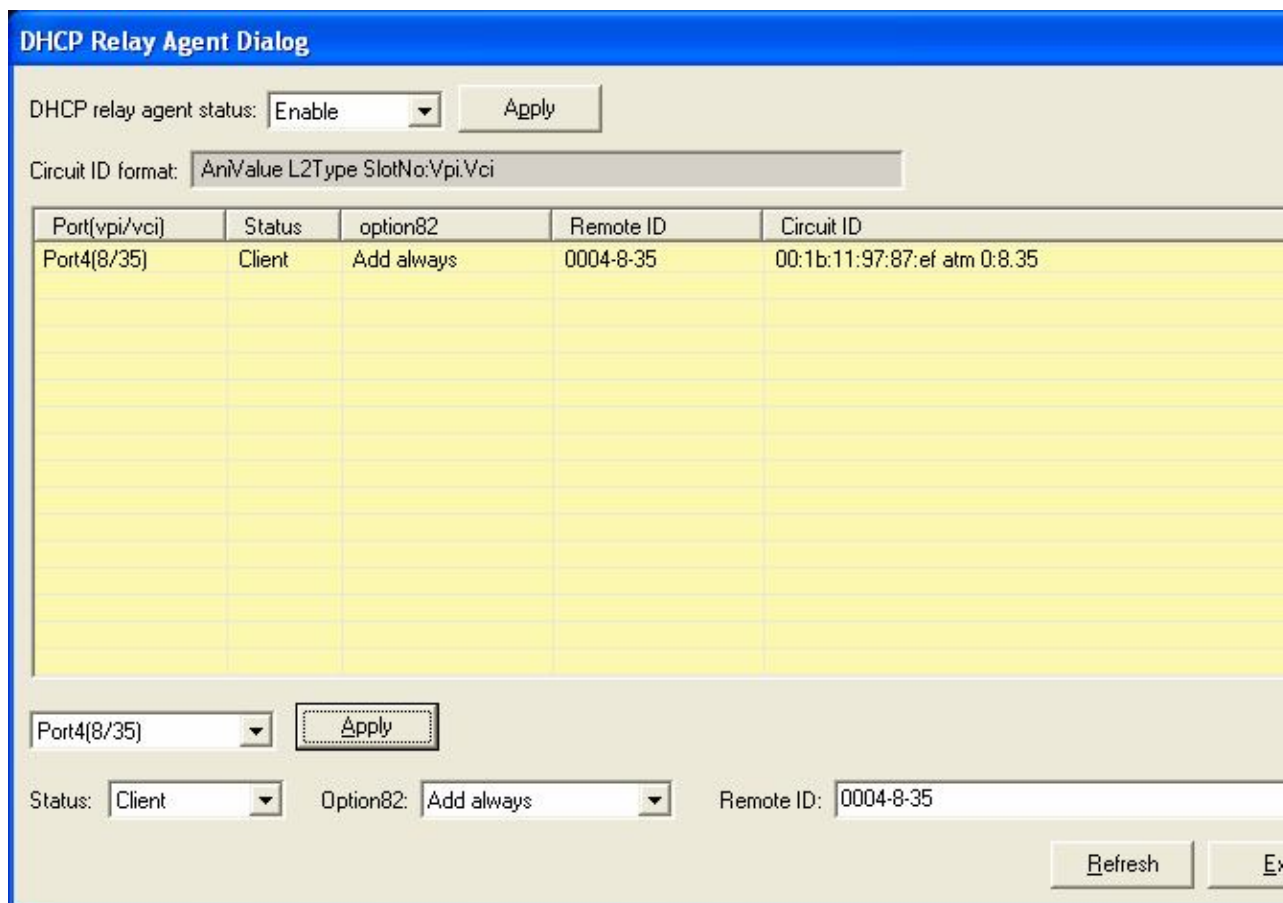
Рисунок 3-43. Диалог настройки функции DHCP Relay Agent (DRA)
