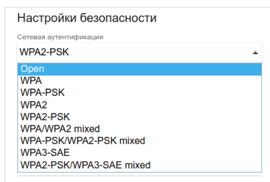
Рисунок 138. Типы аутентификации, поддерживаемые маршрутизатором.
