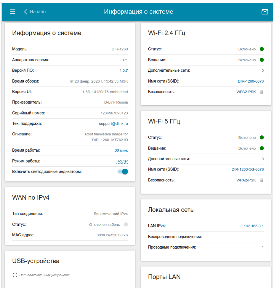
Рисунок 25. Страница информации о системе.
