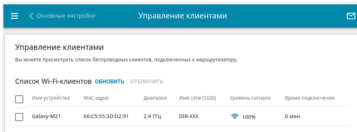
Рисунок 142. Страница для управления подключенными беспроводными устройствами.
