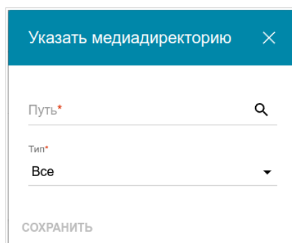
Рисунок 162. Добавление медиадиректории.
