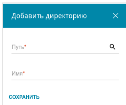
Рисунок 158. Добавление директории.
