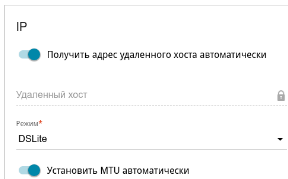
Рисунок 100. Страница добавления соединения типа IPv4 over IPv6. Раздел IP.
