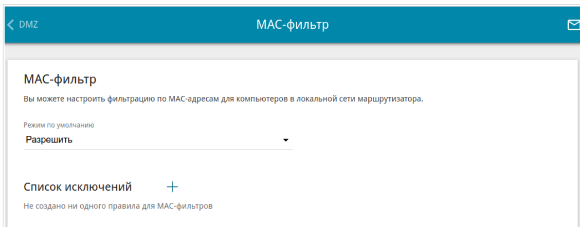
Рисунок 207. Страница Межсетевой экран / MAC-фильтр .
