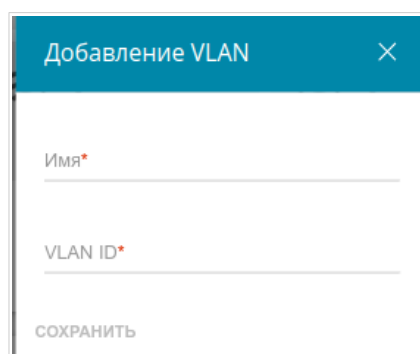
Рисунок 61. Добавление подключения.
