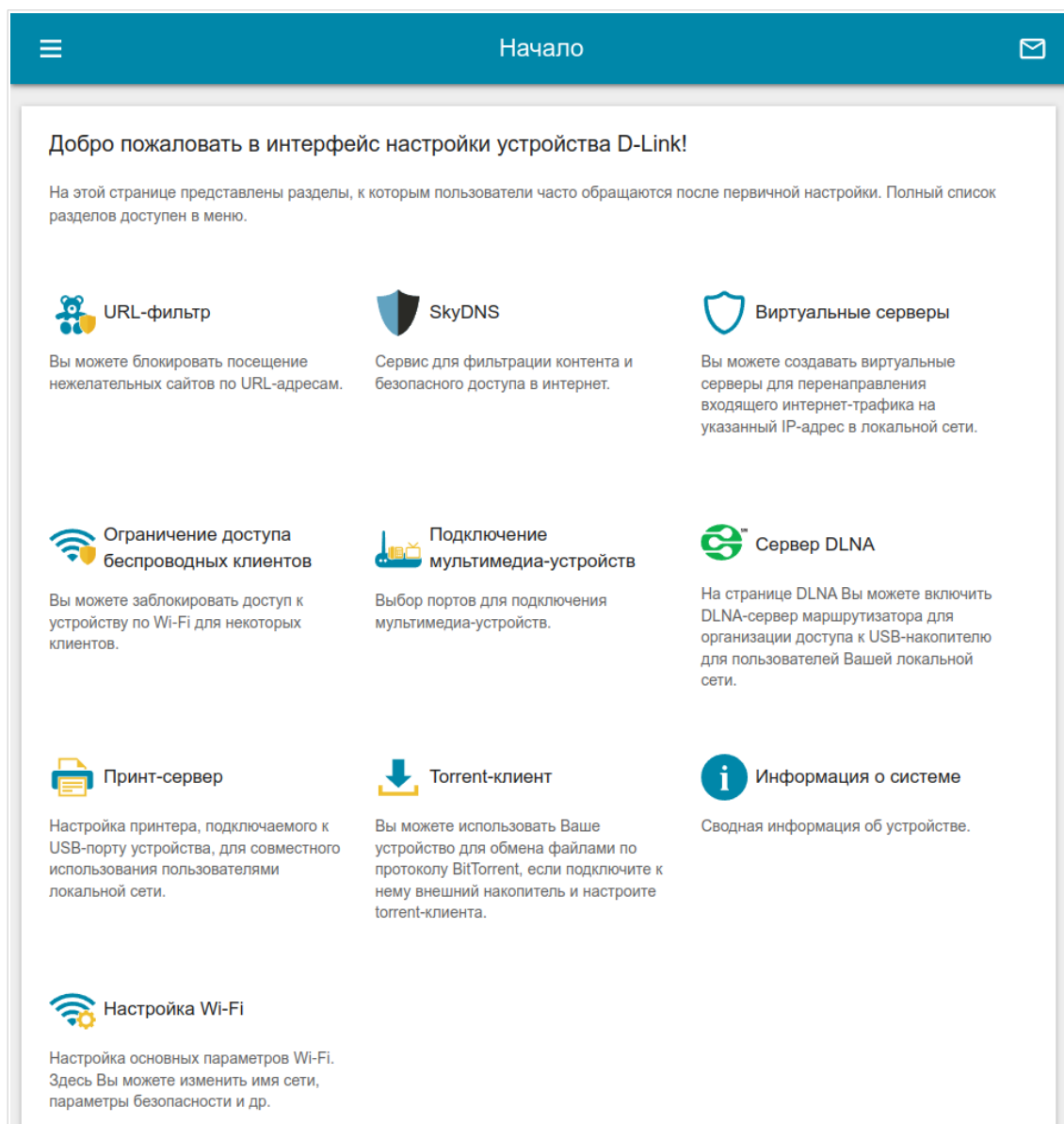
Рисунок 26. Страница Начало .
