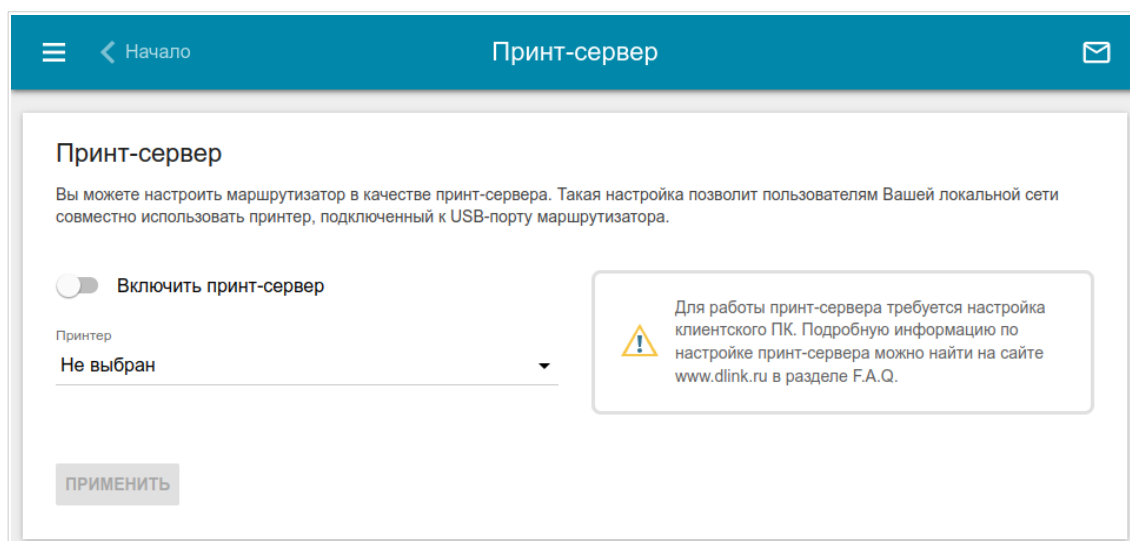
Рисунок 153. Страница Принт-сервер .
