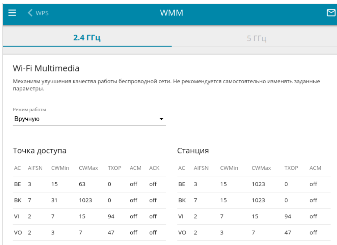
Рисунок 144. Страница для настройки функции WMM.
