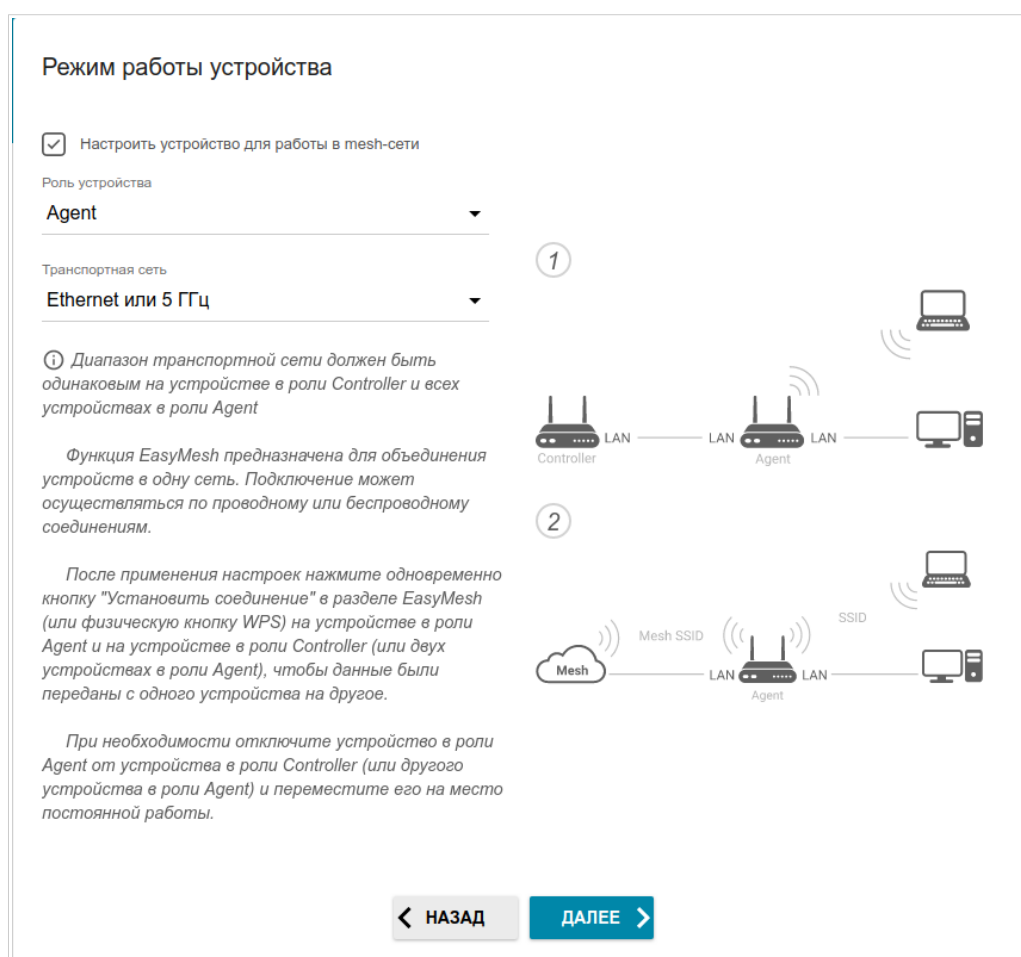
Рисунок 41. Настройка функции EasyMesh для зависимого устройства.
