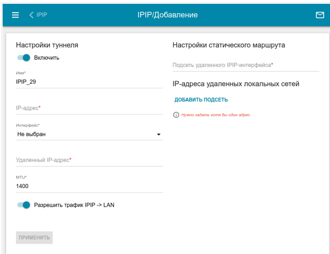
Рисунок 126. Страница добавления IPIP-туннеля.
