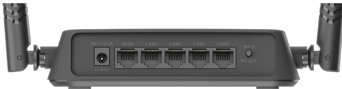
Рисунок 2. Вид задней панели.
