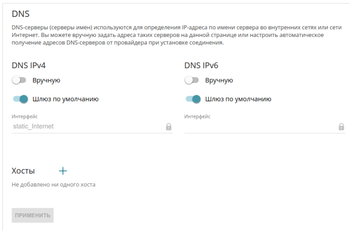
Рисунок 73. Страница Настройки / Интернет / DNS .
