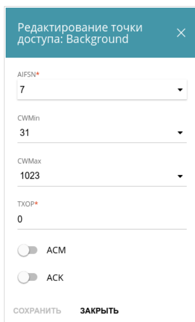
Рисунок 100. Окно для изменения параметров функции WMM.
