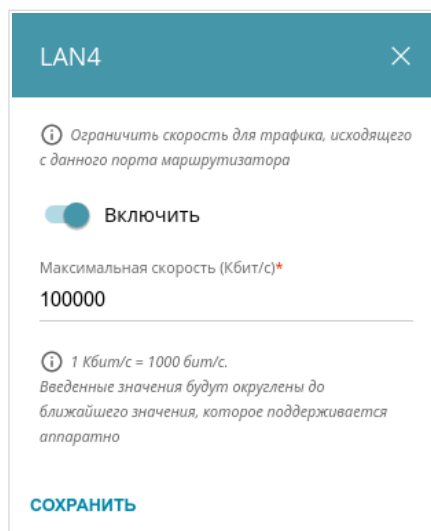
Рисунок 118. Окно для настройки ограничения скорости.
