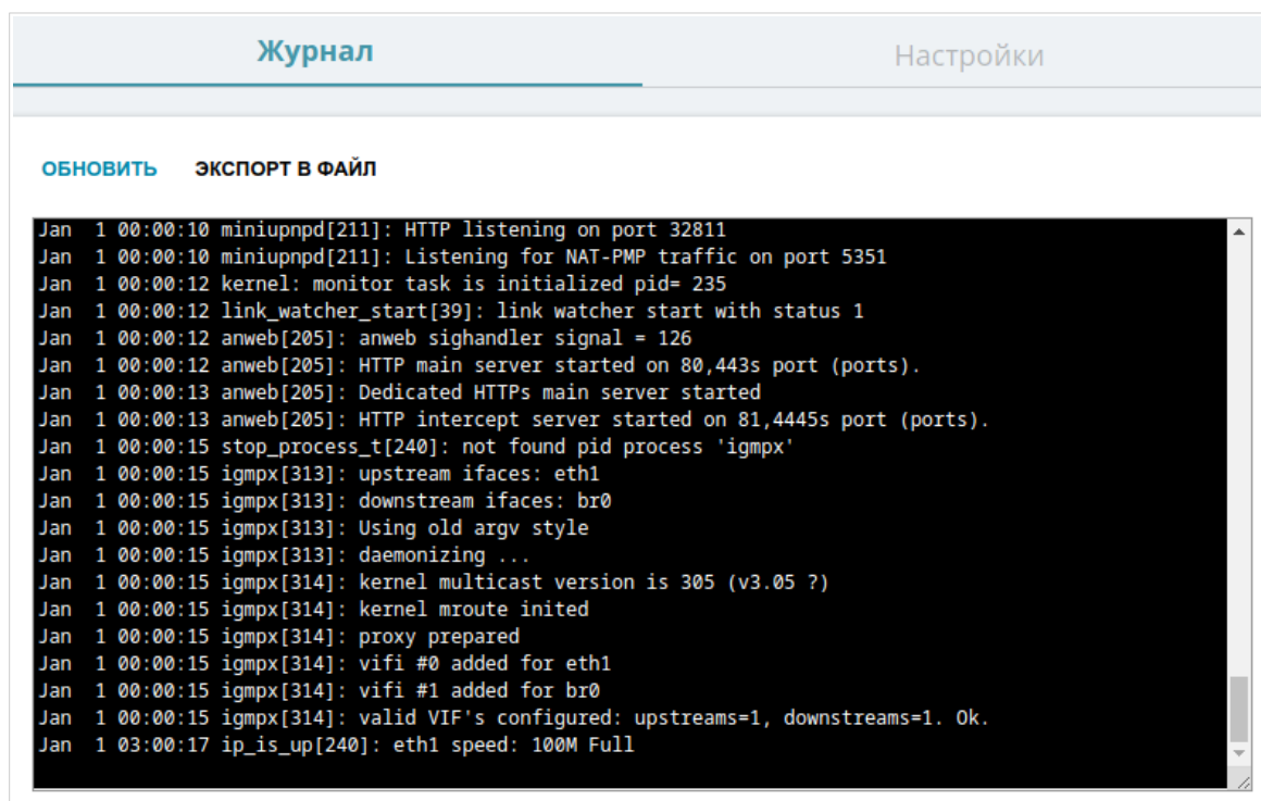
Рисунок 126. Страница Управление / Журнал событий . Вкладка Журнал .
