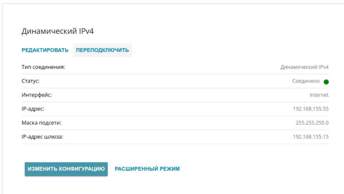
Рисунок 54. Страница Настройки / Интернет / WAN . Упрощенный режим.
