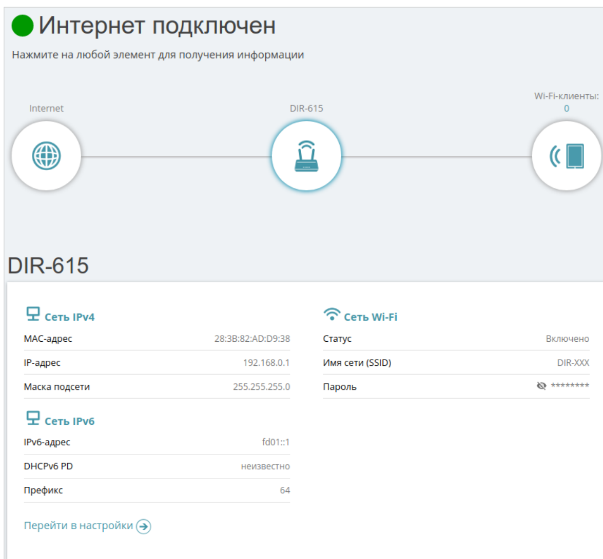
Рисунок 28. Страница Начало . Раздел DIR-615 .
