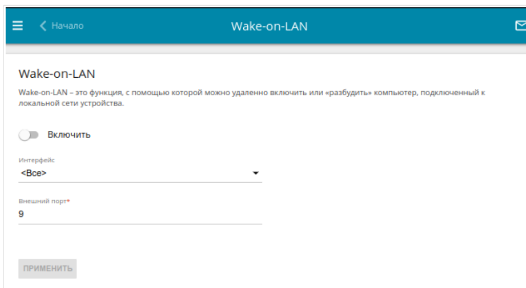
Рисунок 126. Страница Дополнительно / Wake-on-LAN .
