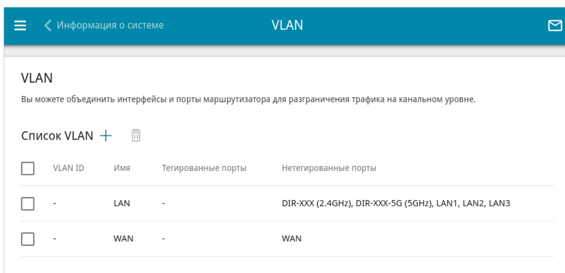
Рисунок 107. Страница Дополнительно / VLAN .
