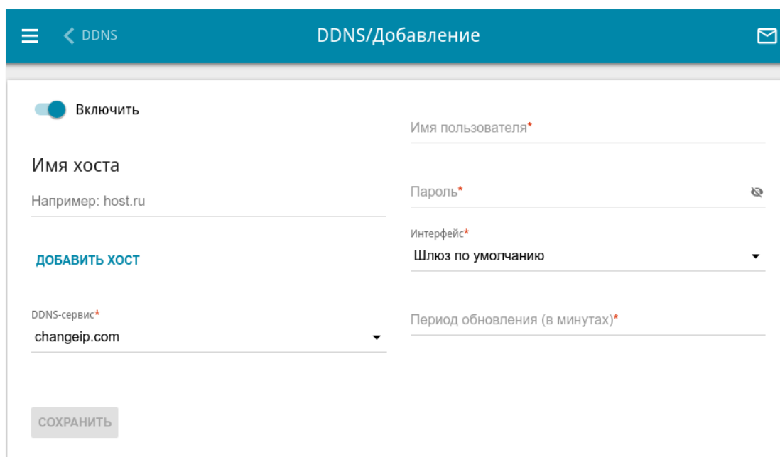
Рисунок 155. Страница добавления нового DDNS-сервиса.
