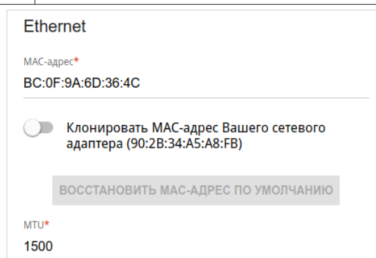
Рисунок 76. Страница добавления соединения типа Статический IPv6 . Раздел Ethernet .
