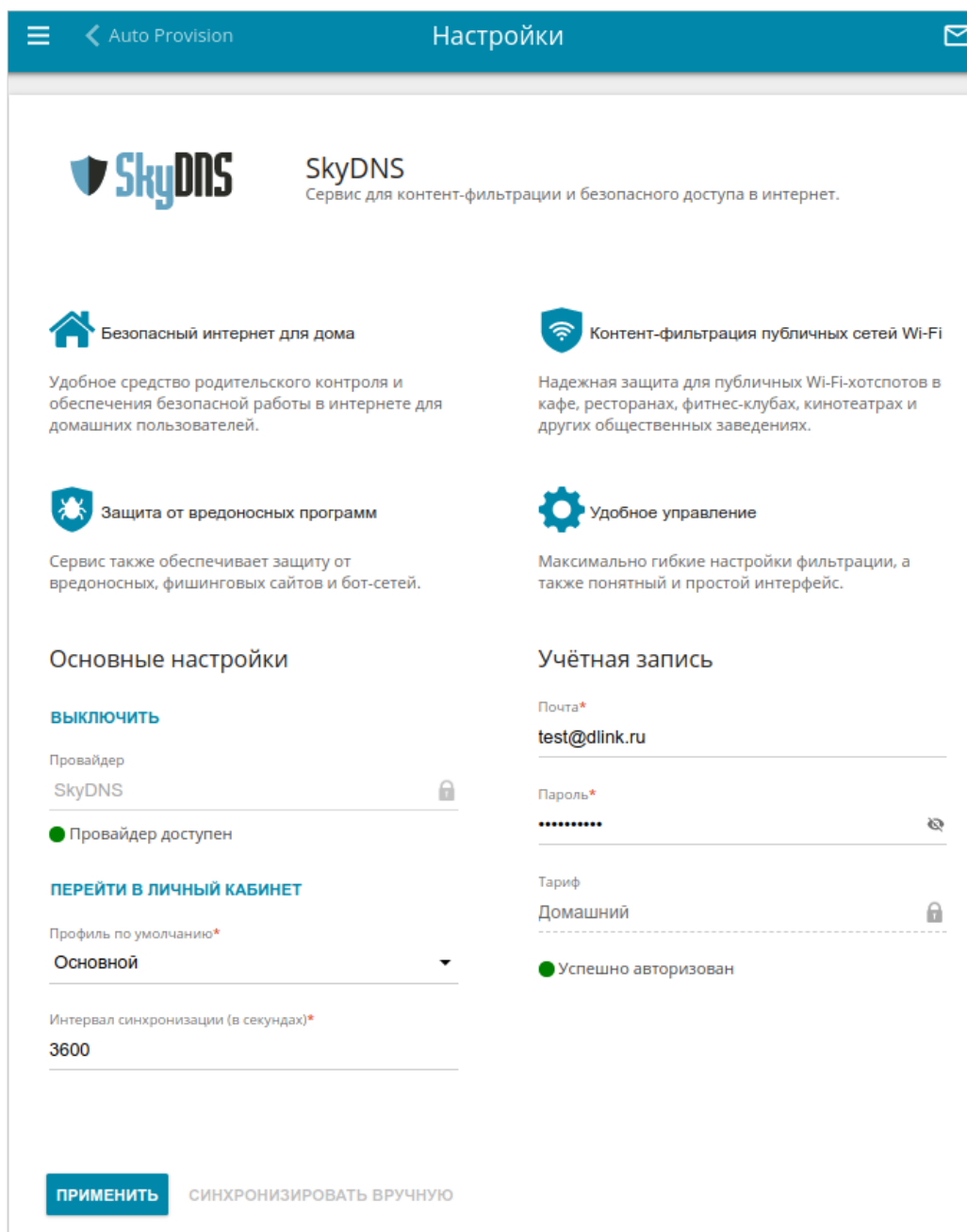
Рисунок 206. Страница SkyDNS / Настройки .
