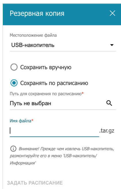
Рисунок 190. Окно создания резервной копии.
