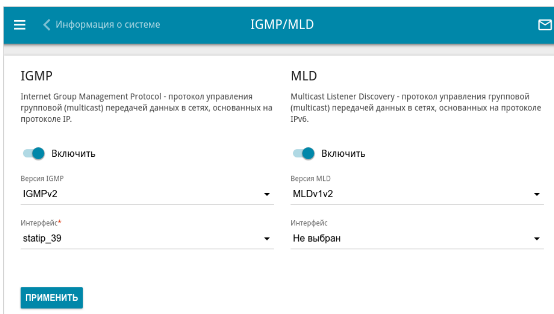
Рисунок 165. Страница Дополнительно / IGMP/MLD .
