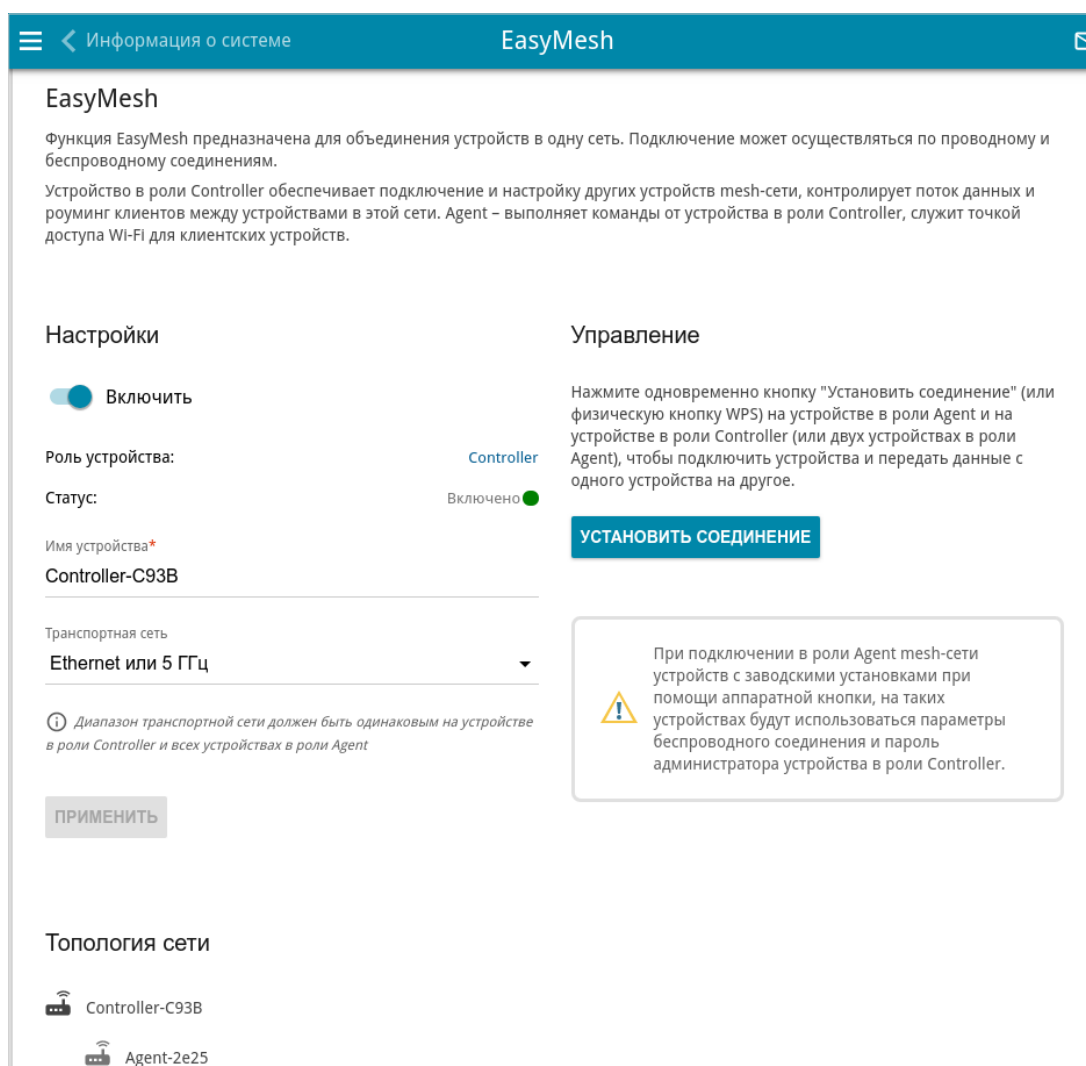
Рисунок 126. Страница Wi-Fi / EasyMesh .
