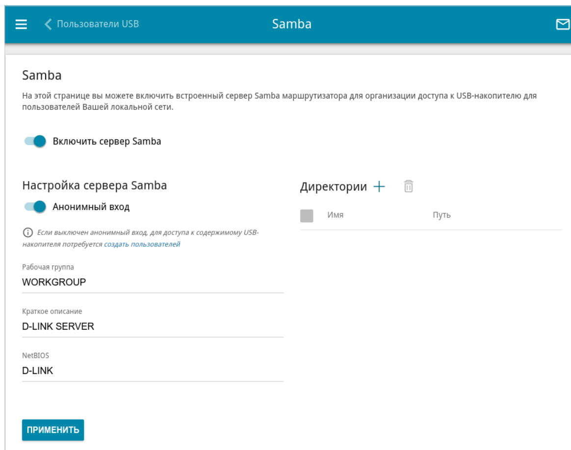
Рисунок 133. Страница USB-накопитель / Samba .
