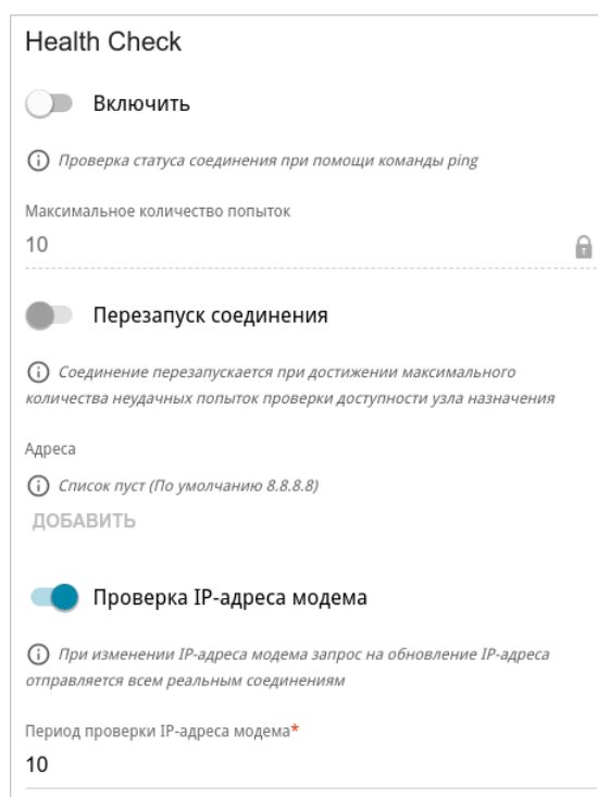
Рисунок 96. Страница добавления соединения типа Мобильный интернет . Раздел Health Check .
