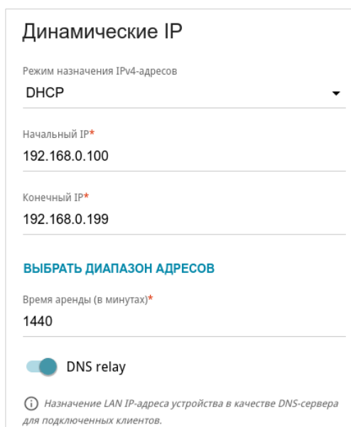
Рисунок 98. Настройка локального интерфейса. Вкладка IPv4. Раздел Динамические IP.
