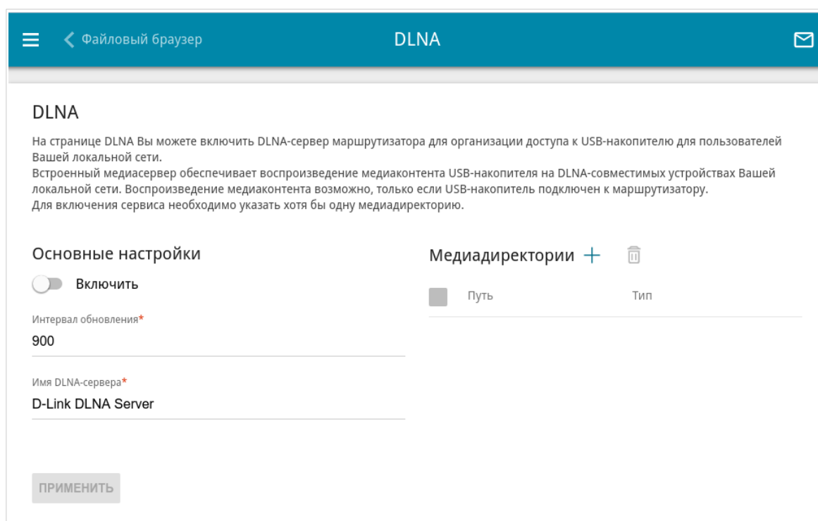
Рисунок 137. Страница USB-накопитель / DLNA .
