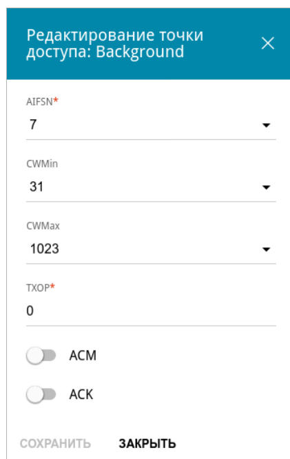
Рисунок 119. Окно для изменения параметров функции WMM.
