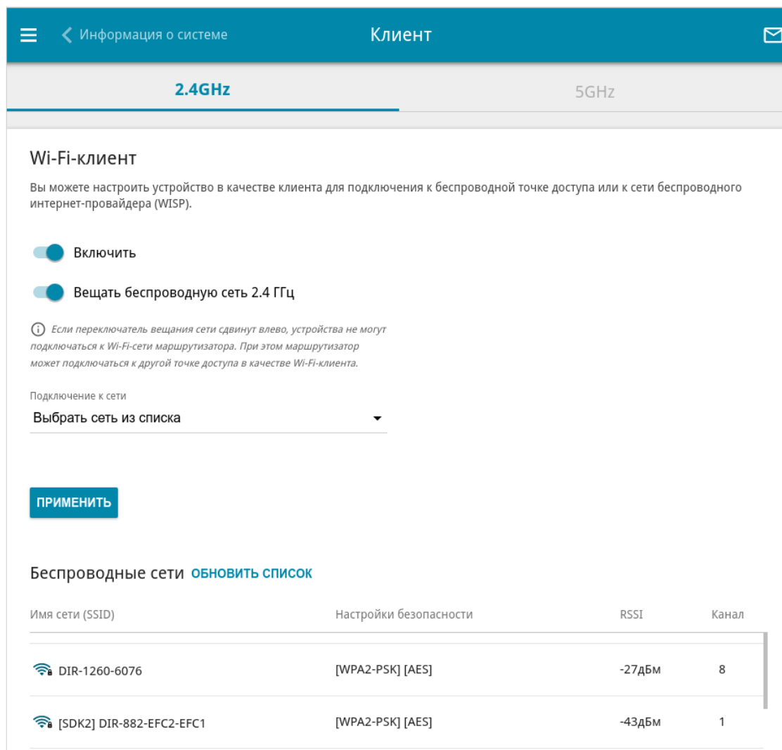
Рисунок 120. Страница для настройки маршрутизатора в качестве клиента.
