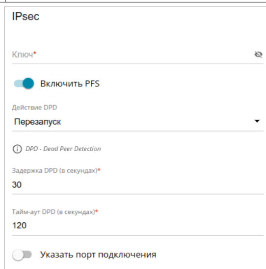
Рисунок 85. Страница добавления соединения типа L2TP over IPsec . Раздел IPsec .
