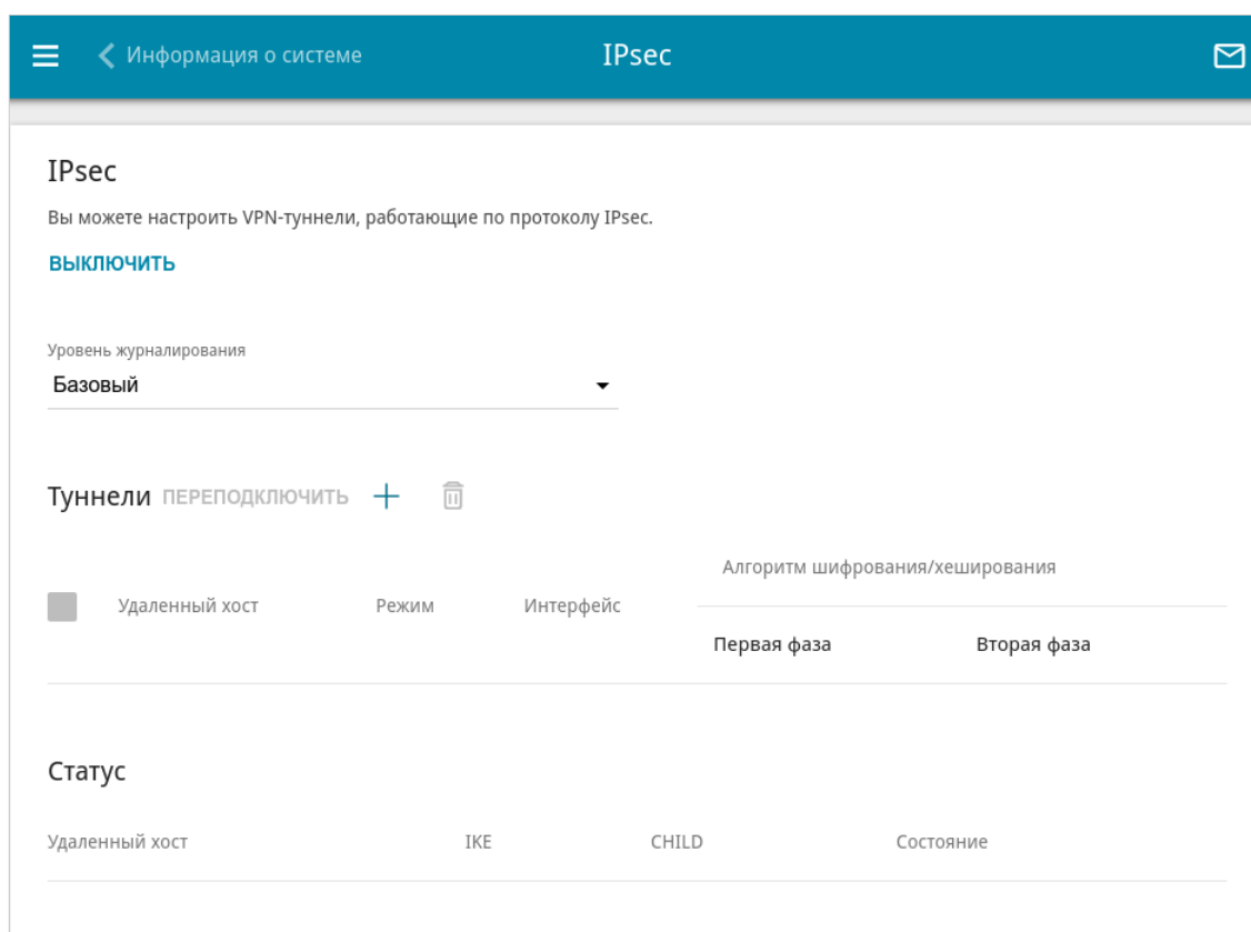
Рисунок 167. Страница VPN / IPsec.
