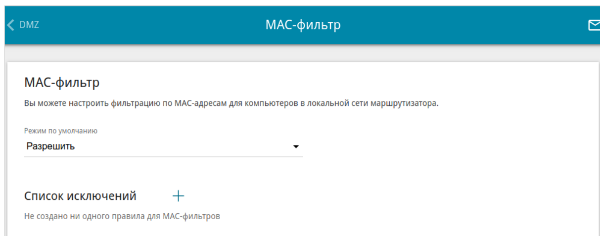
Рисунок 182. Страница Межсетевой экран / MAC-фильтр .
