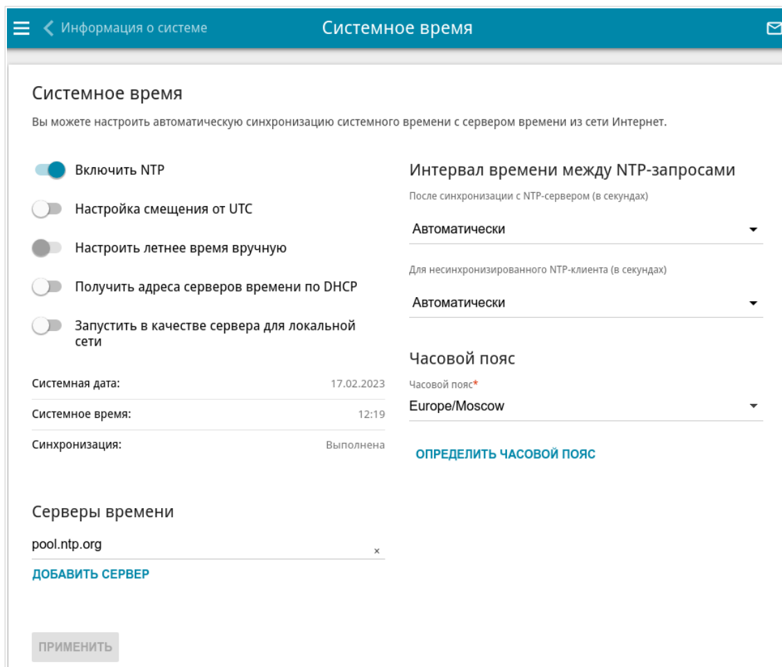
Рисунок 204. Страница Система / Системное время .
