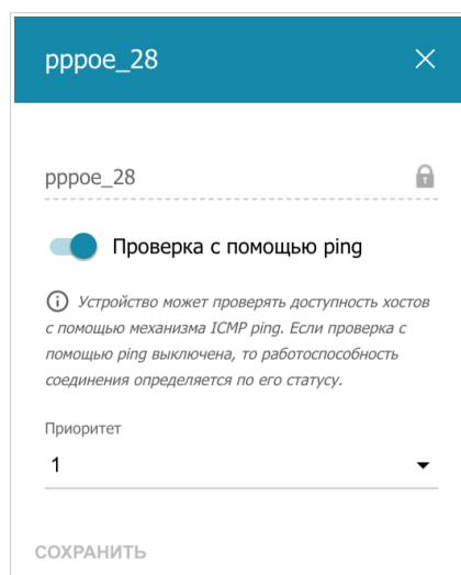
Рисунок 108. Окно изменения уровня приоритета соединения.
