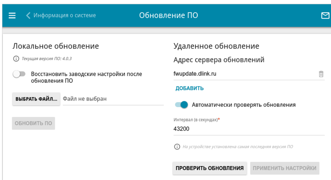
Рисунок 193. Страница Система / Обновление ПО .
