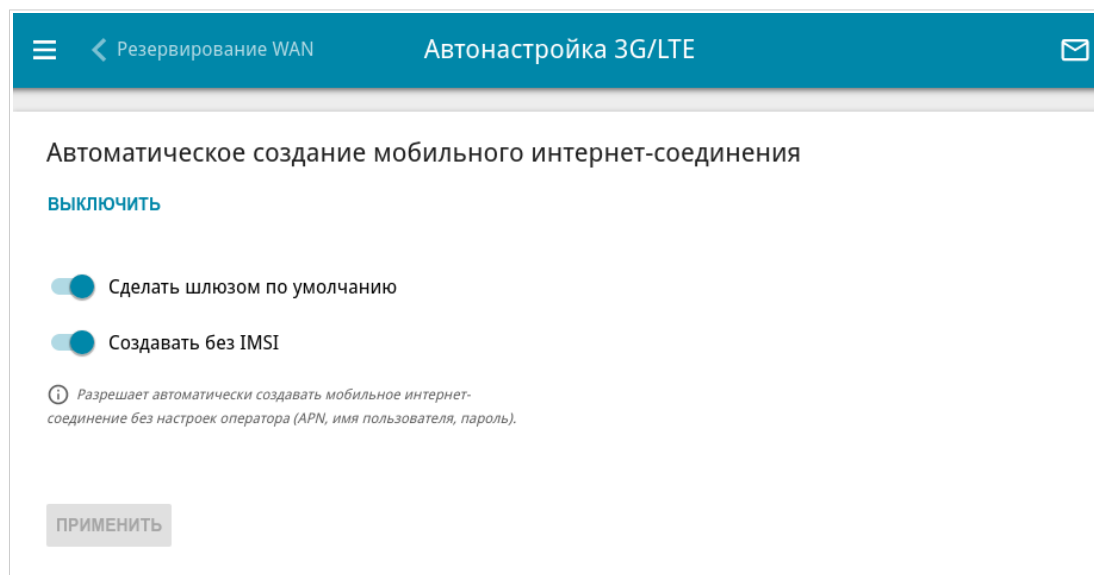
Рисунок 109. Страница Настройка соединений / Автонастройка 3G/LTE .
