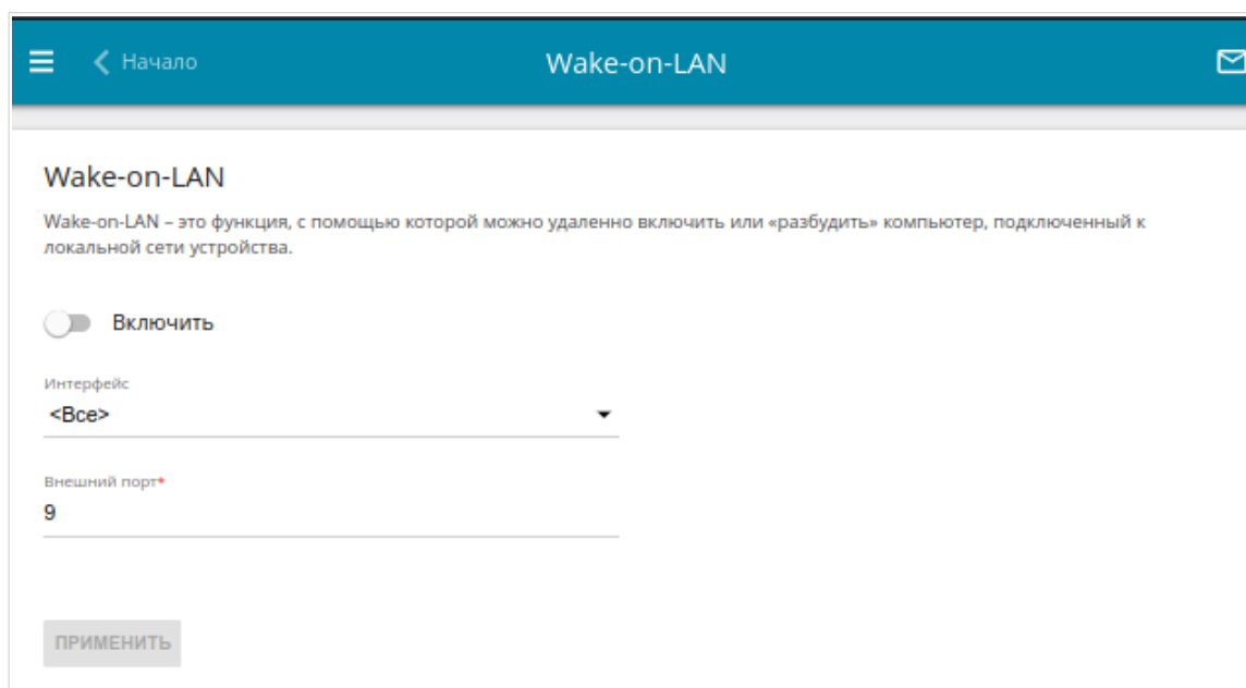
Рисунок 176. Страница Дополнительно / Wake-on-LAN .
