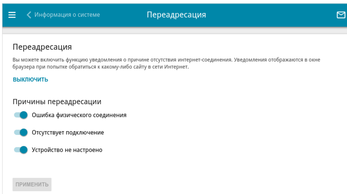
Рисунок 158. Страница Дополнительно / Переадресация .
