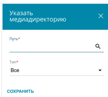
Рисунок 138. Добавление медиадиректории.
