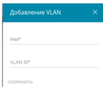
Рисунок 61. Добавление подключения.
