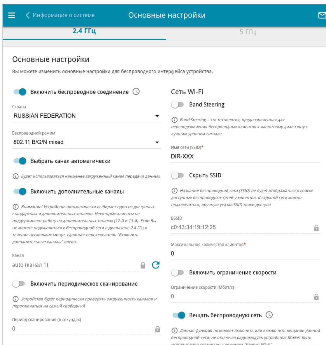
Рисунок 110. Основные настройки беспроводной локальной сети в диапазоне 2,4 ГГц.
