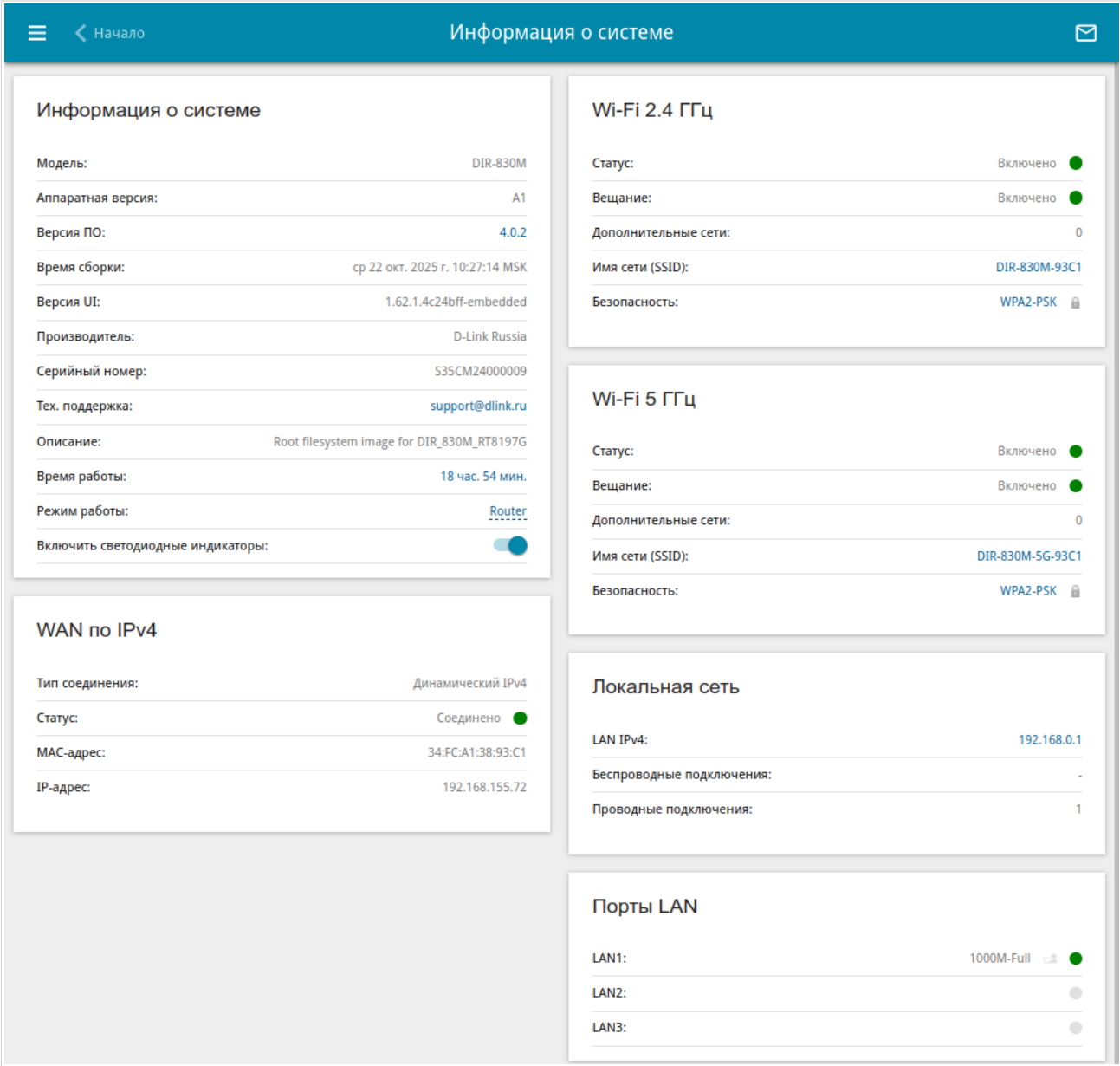
Рисунок 25. Страница информации о системе.
