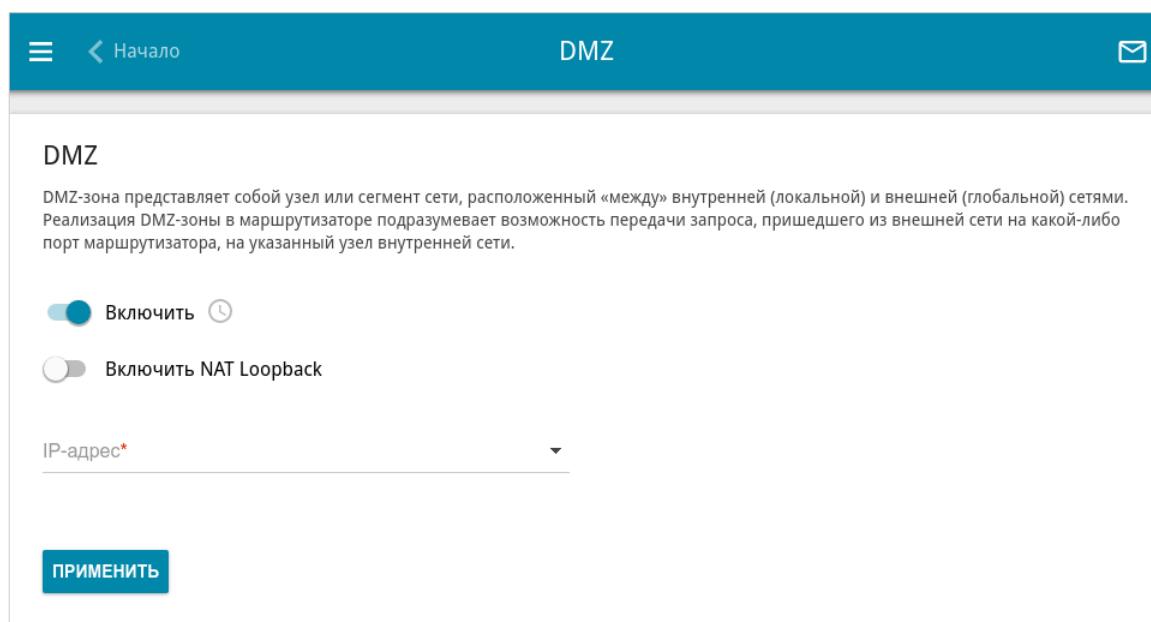
Рисунок 143. Страница Межсетевой экран / DMZ .
