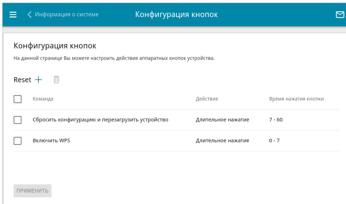
Рисунок 152. Страница Система / Конфигурация кнопок .
