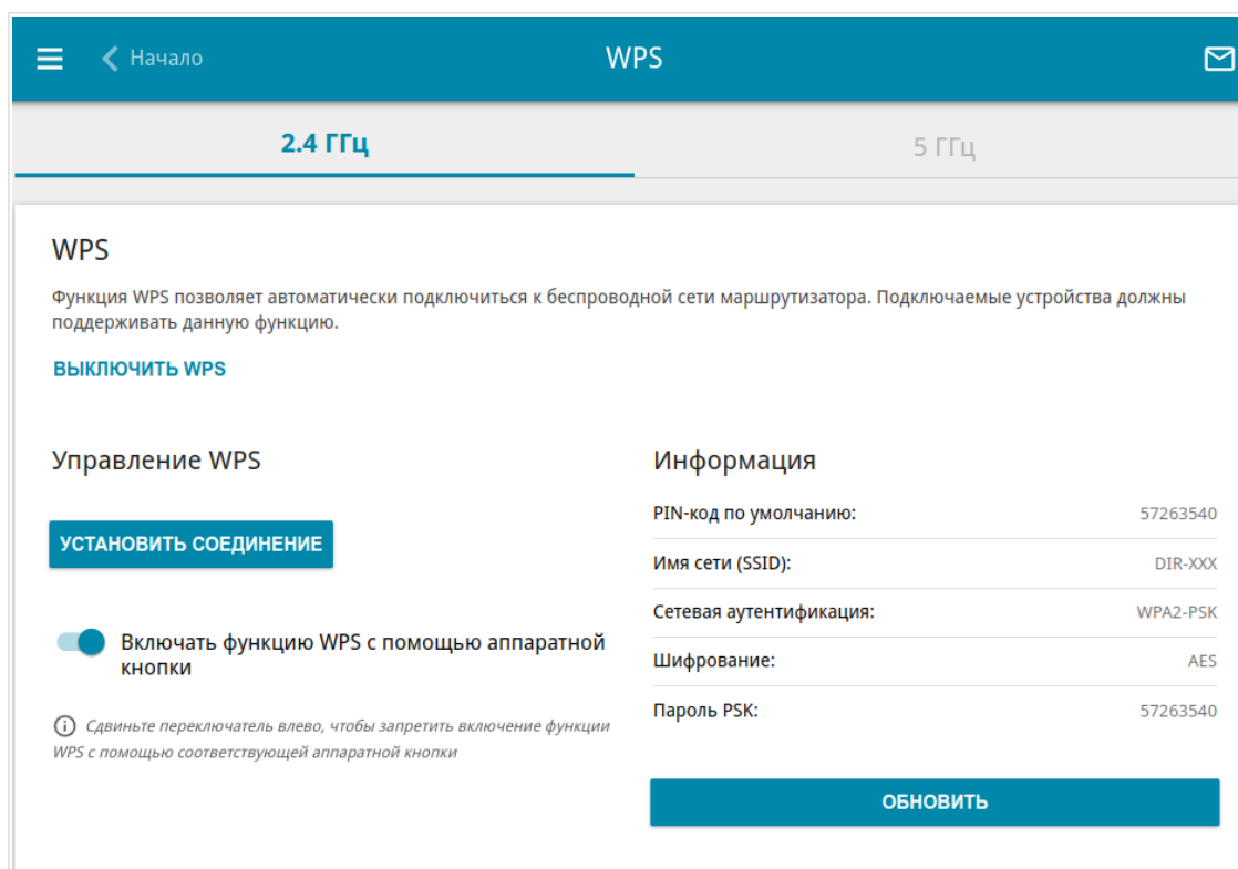
Рисунок 105. Страница для настройки функции WPS.
