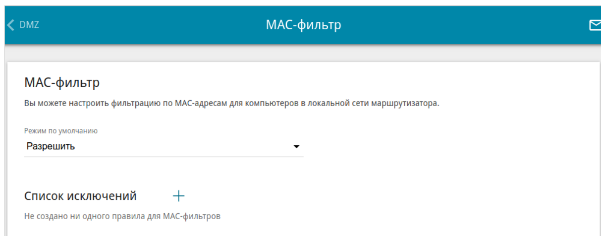
Рисунок 144. Страница Межсетевой экран / MAC-фильтр .
