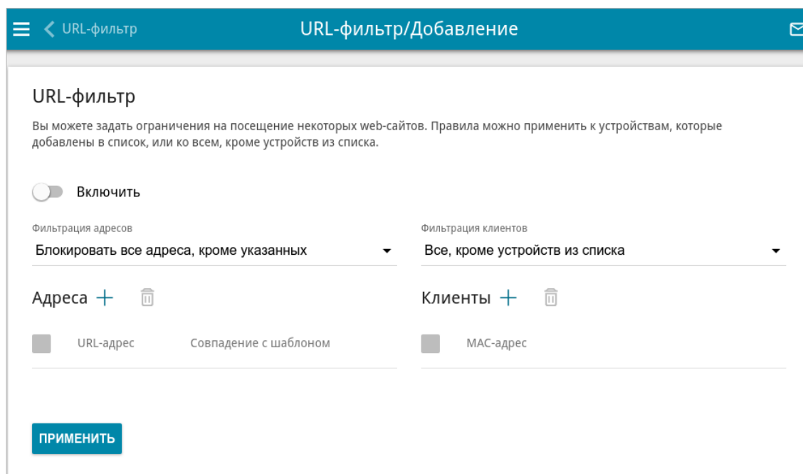
Рисунок 147. Страница добавления правила для URL-фильтра.
