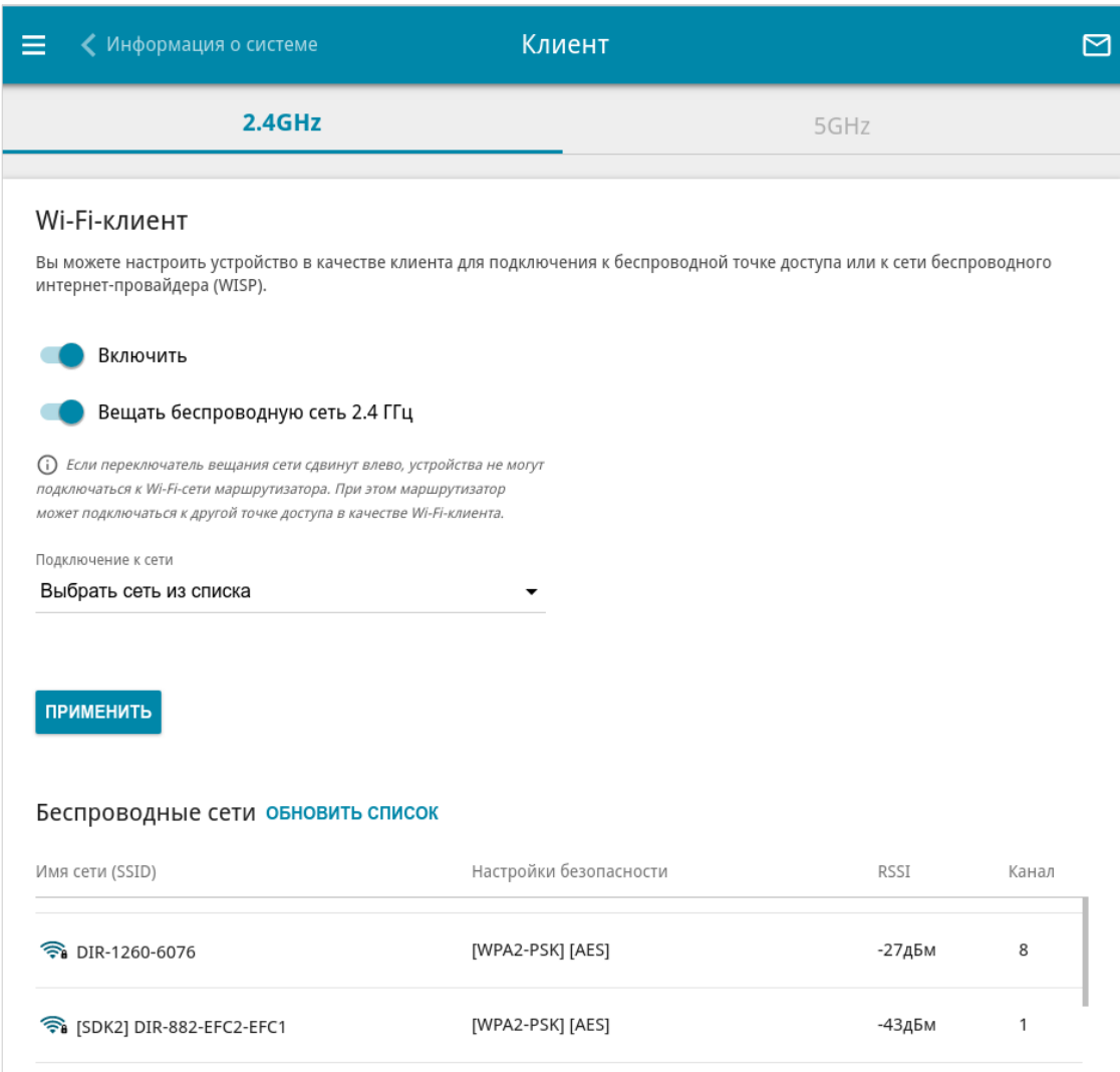
Рисунок 108. Страница для настройки маршрутизатора в качестве клиента.
