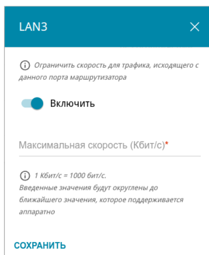
Рисунок 124. Окно для настройки ограничения скорости.
