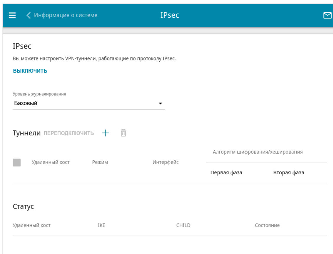
Рисунок 134. Страница Дополнительно / IPsec .
