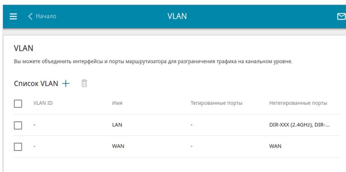
Рисунок 116. Страница Дополнительно / VLAN .
