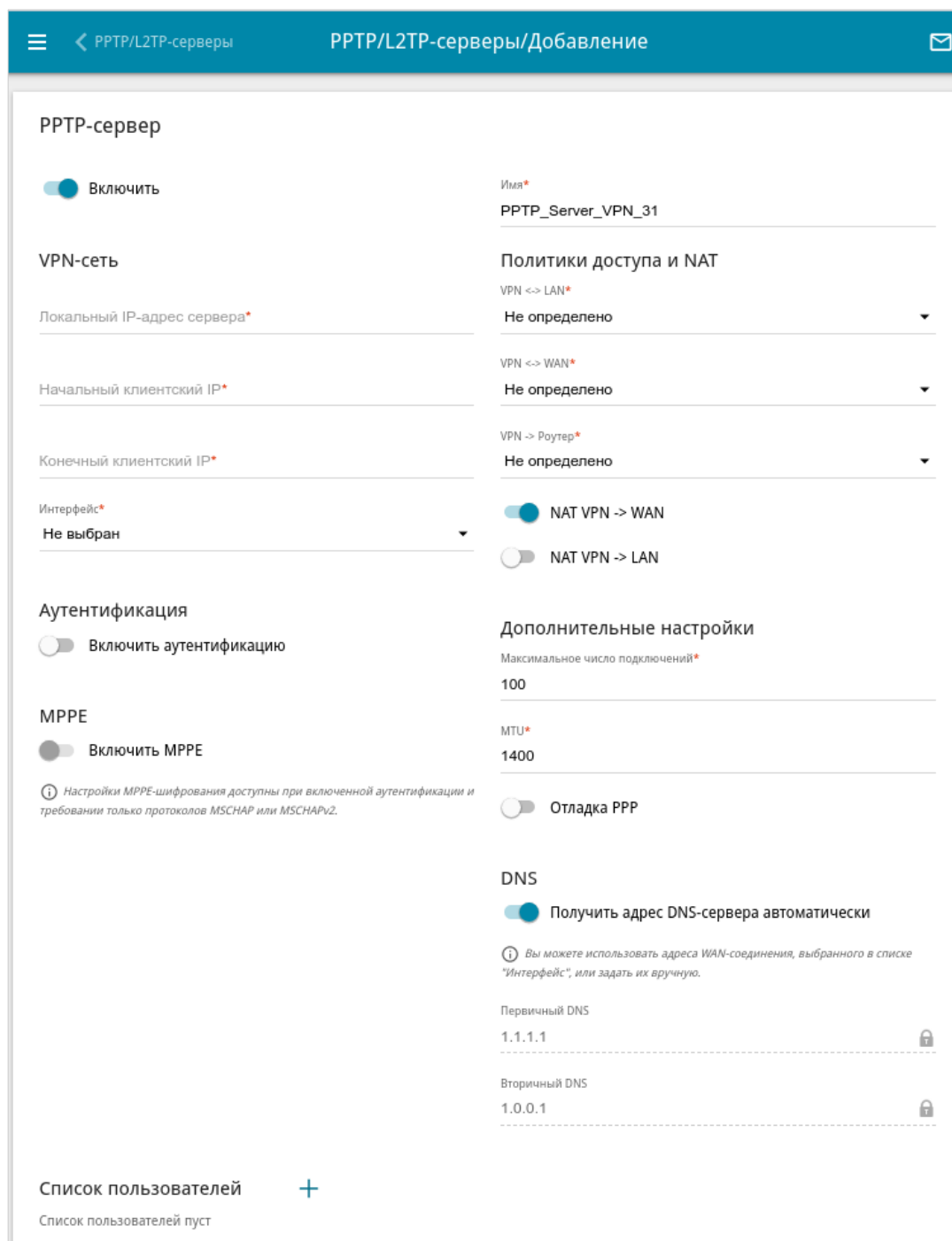
Рисунок 123. Страница добавления PPTP-сервера.
