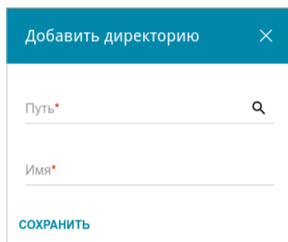
Рисунок 151. Добавление директории.
