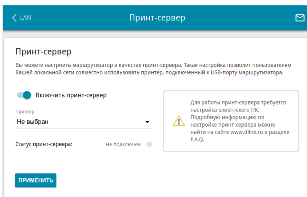
Рисунок 146. Страница Принт-сервер .
