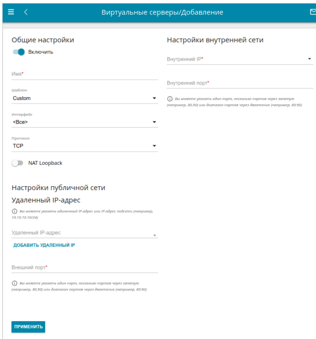
Рисунок 169. Страница добавления виртуального сервера.
