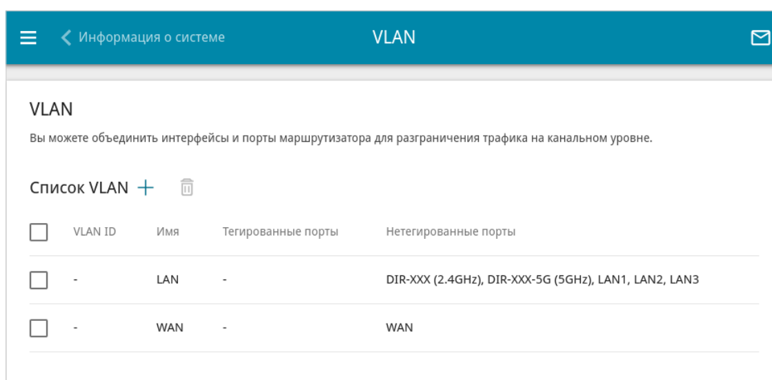
Рисунок 139. Страница Дополнительно / VLAN .
