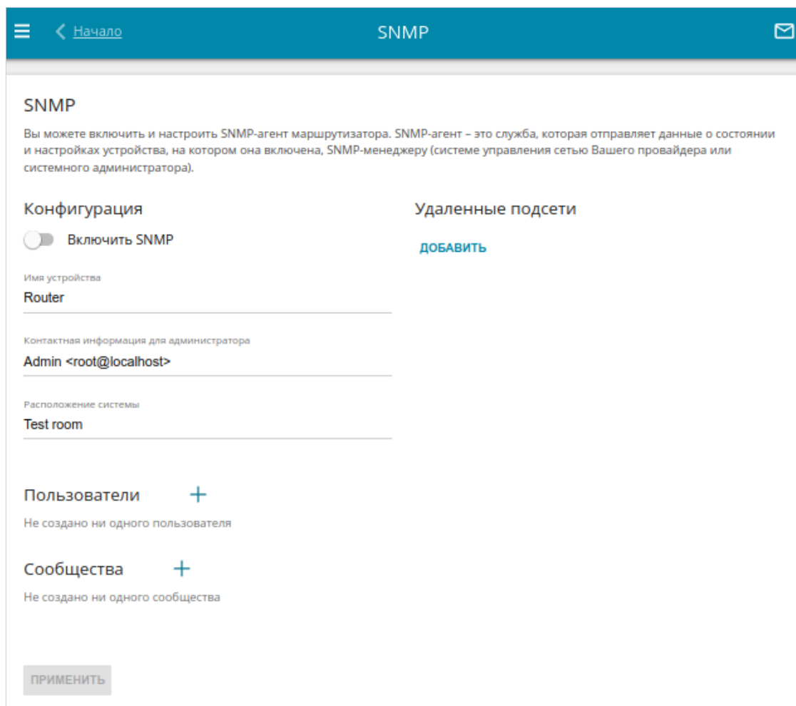
Рисунок 142. Страница Дополнительно / SNMP .
