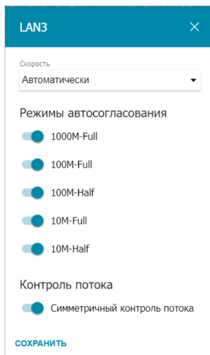
Рисунок 148. Окно изменения настроек порта маршрутизатора.
