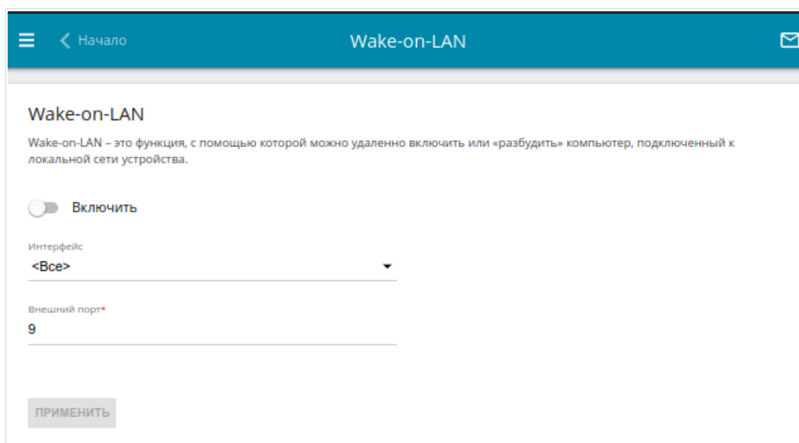
Рисунок 165. Страница Дополнительно / Wake-on-LAN .
