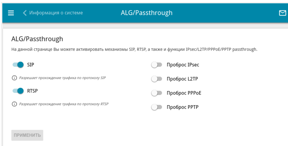
Рисунок 158. Страница Дополнительно / ALG/Passthrough .
