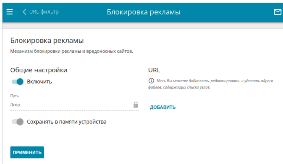
Рисунок 175. Страница Межсетевой экран / Блокировка рекламы .
