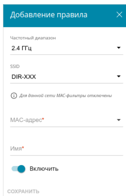
Рисунок 135. Окно для добавления правила MAC-фильтра.
