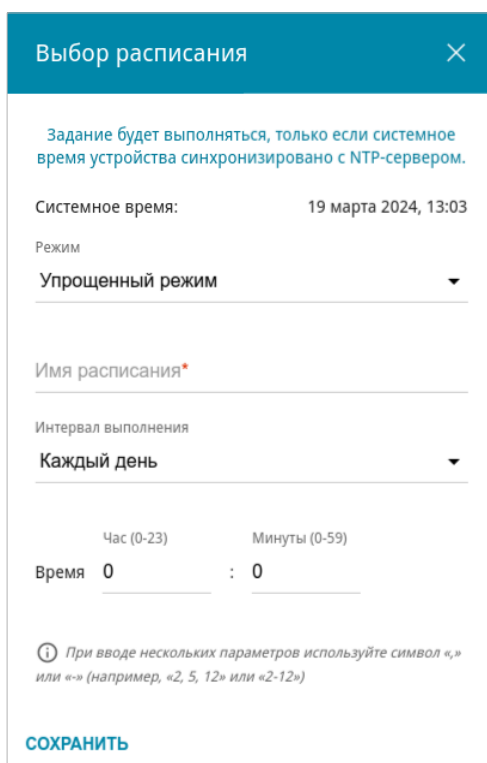
Рисунок 183. Окно настройки автоматической перезагрузки устройства по расписанию.
