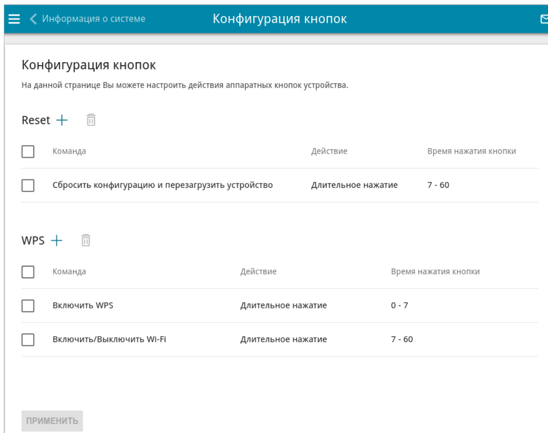
Рисунок 179. Страница Система / Конфигурация кнопок .
