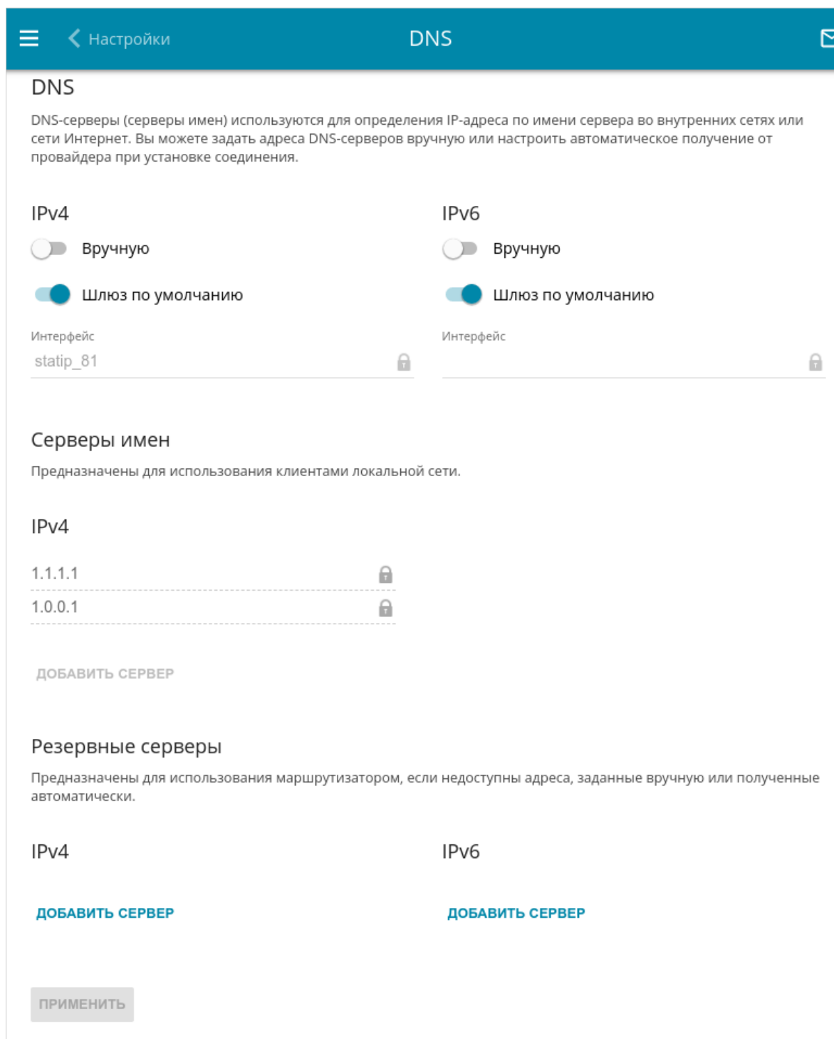
Рисунок 144. Страница Дополнительно / DNS .
