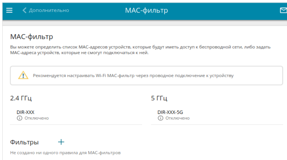
Рисунок 134. Страница для настройки MAC-фильтра для беспроводной сети.
