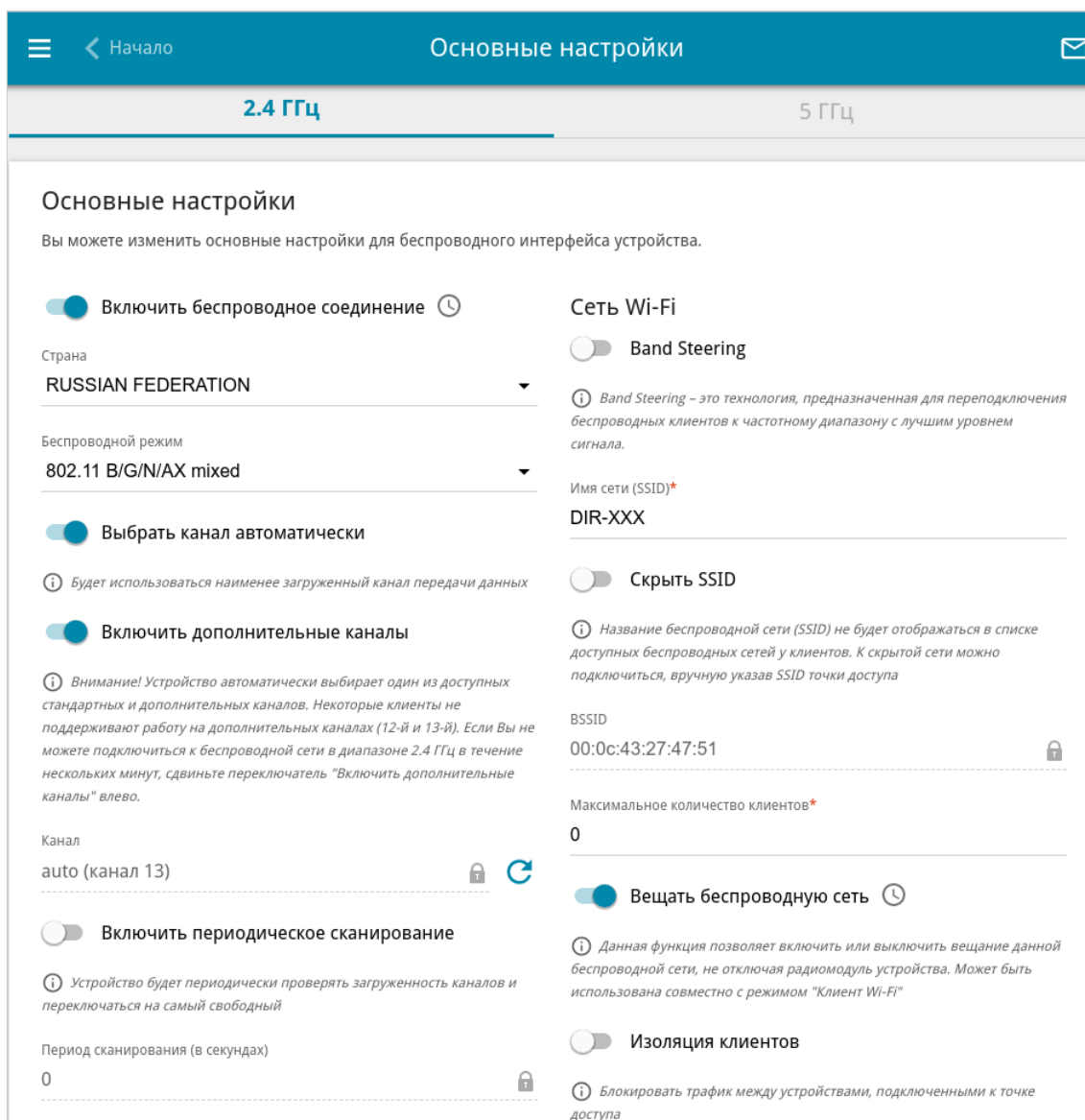
Рисунок 122. Основные настройки беспроводной локальной сети в диапазоне 2,4 ГГц.
