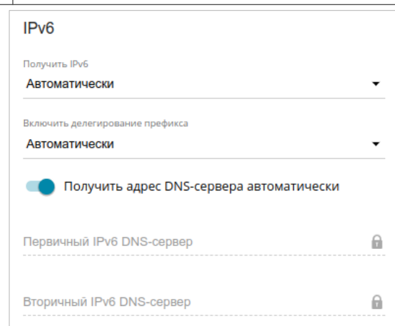
Рисунок 81. Страница добавления соединения типа L2TP Dual Stack . Раздел IPv6 .
