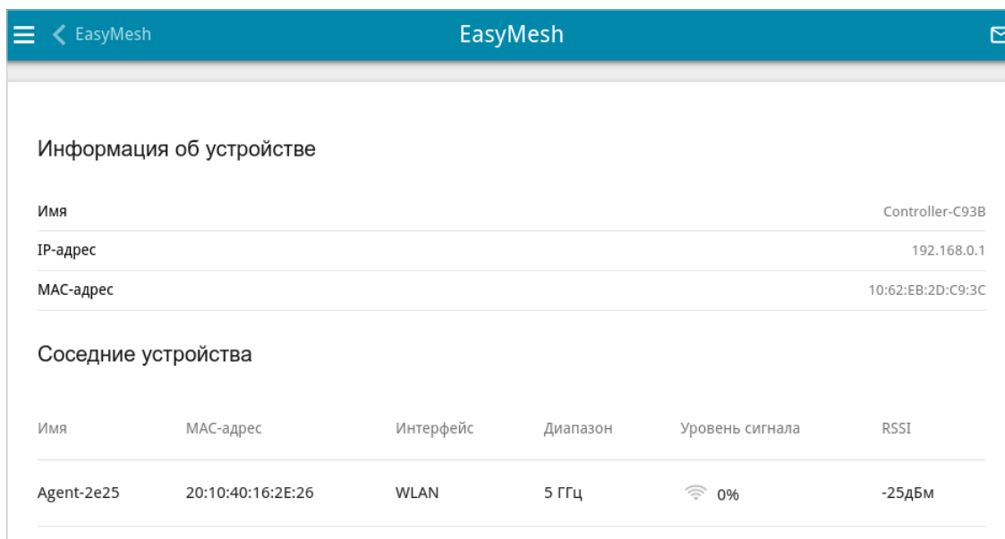
Рисунок 137. Страница с информацией об устройстве.
