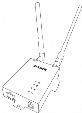
Рис. 4: Подключение антенн
