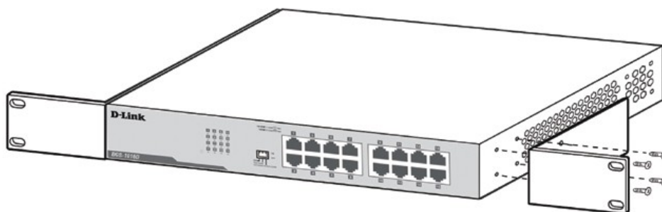
Рисунок 1 — Крепление кронштейнов
