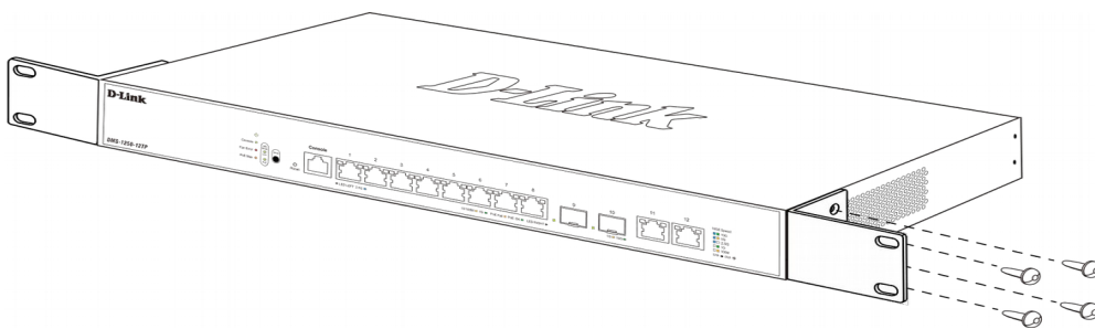
Рисунок 2 — Крепление кронштейнов
