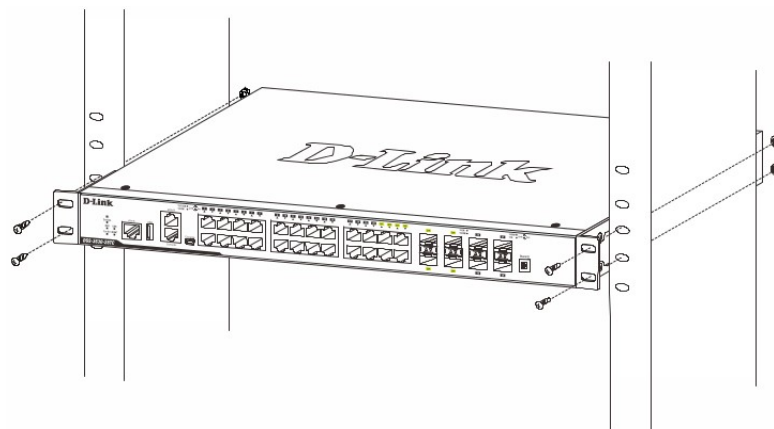
Рисунок 3 — Установка коммутатора в стойку
