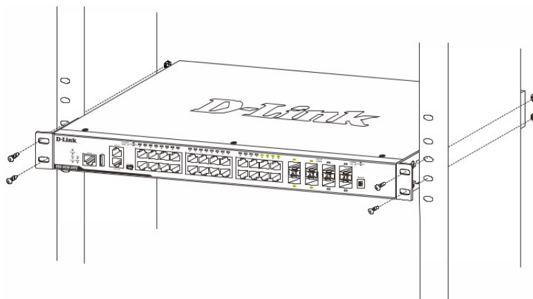
Рисунок 3 — Установка коммутатора в стойку
