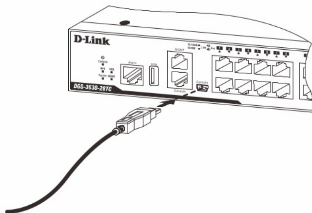
Рисунок 14 — Подключение консольного кабеля к порту mini-USB коммутатора
