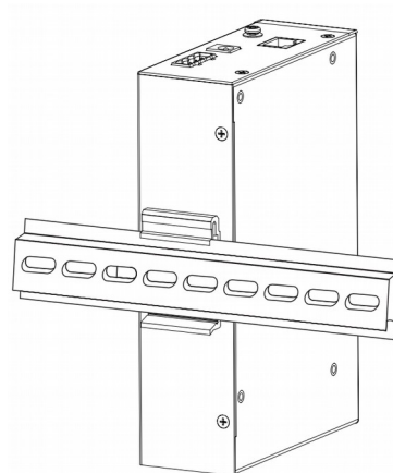
Рисунок 3 — Установка коммутатора на DIN-рейку
