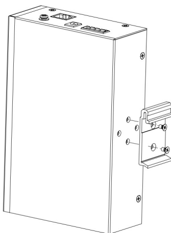
Рисунок 1 — Крепление кронштейна к коммутатору
