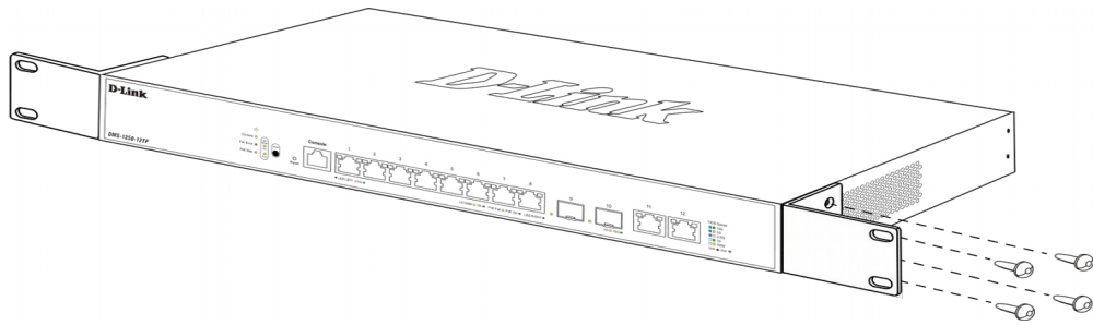
Рисунок 2 — Крепление кронштейнов
