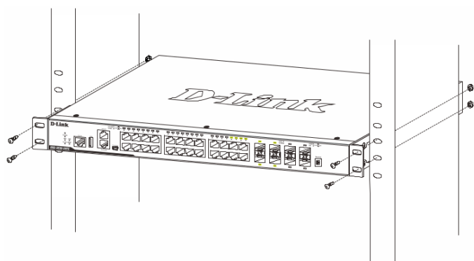
Рисунок 3 — Установка коммутатора в стойку
