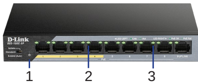
Рисунок 1: Индикаторы передней панели
