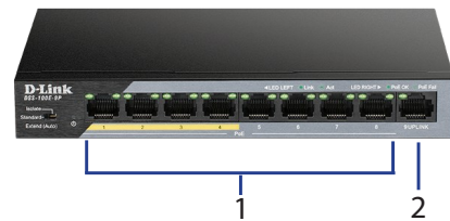
Рисунок 2: Интерфейсы передней панели
