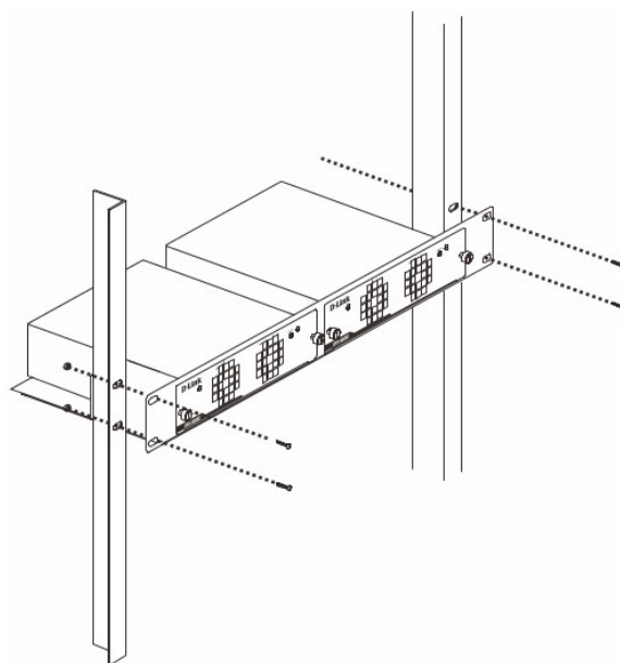
Рисунок 7 — Установка DPS-800 в стандартную стойку для оборудования
