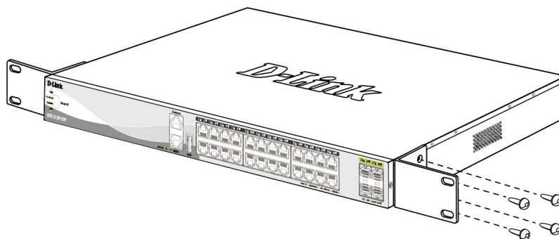
Рисунок 2 — Крепление кронштейнов
