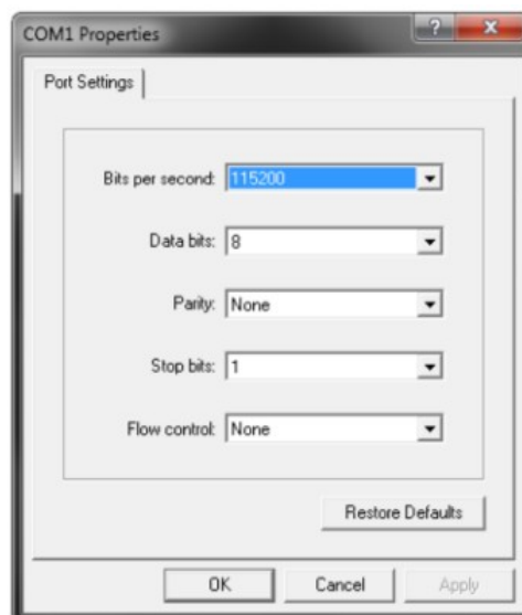
Рисунок 8 — Параметры настройки COM-порта
