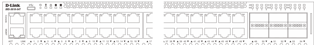
Рис. 2. Индикаторы передней панели DXS-3610-54T
