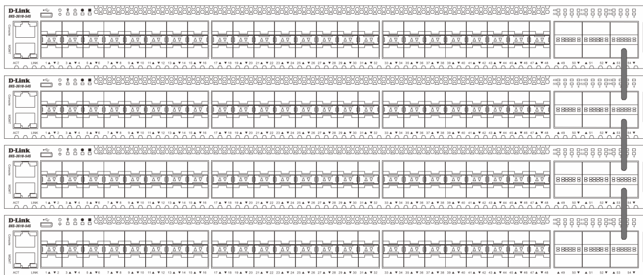
Рис. 20. Линейная топология
