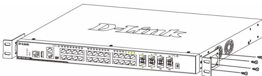
Рисунок 2 — Крепление кронштейнов
