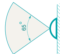
Направленность антенны в вертикальной плоскости
