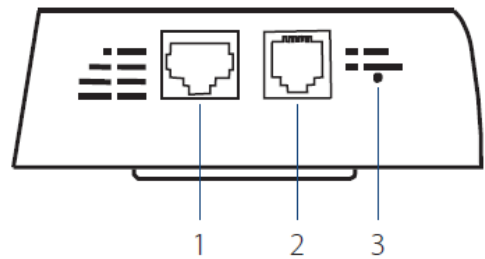
Рисунок 2: Интерфейсы нижней панели
