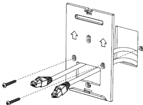
Рисунок 4: Крепление кронштейна
