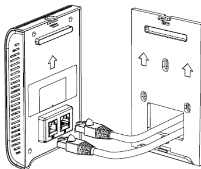
Рисунок 5: Подключение кабеля
