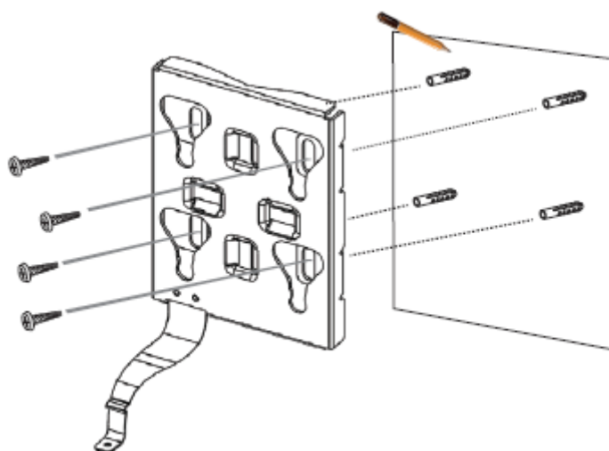
Рисунок 7: Крепление кронштейна
