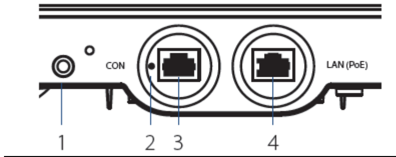
Рисунок 2: Разъемы
